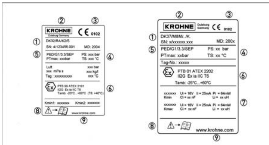
Рисунок 2-2: Шильды
