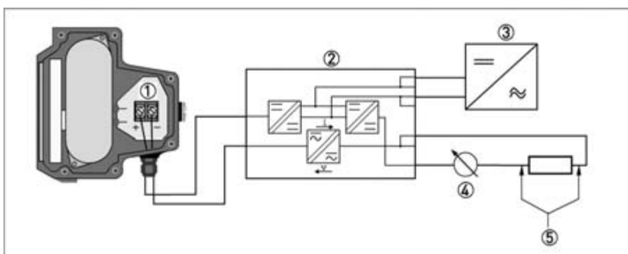
Рисунок 4-6: Электрическое соединение с гальванической изоляцией
