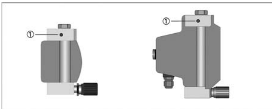
Рисунок 4-7: Заземляющие соединения
