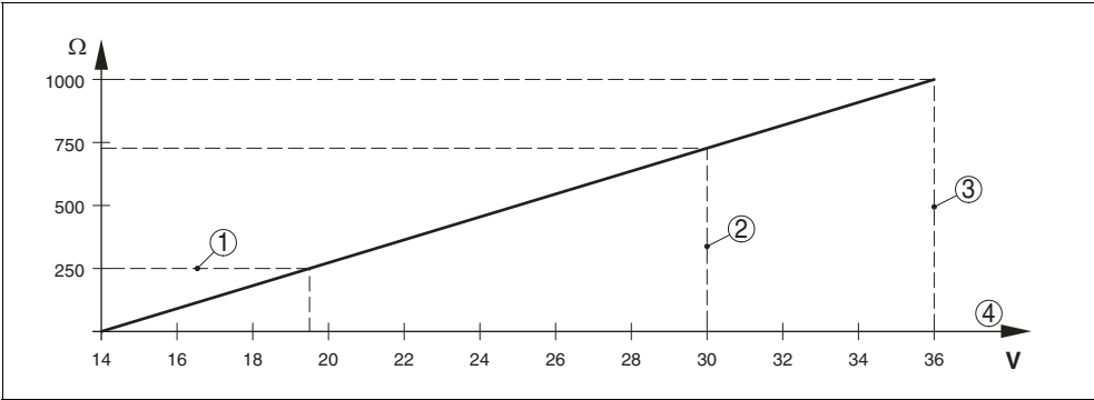
Рис. 26: Диаграмма напряжения 1 Нагрузка HART 2 Предел напряжения для прибора EEx ia 3 Предел напряжения для прибора не-Ex 4 Напряжение питания
