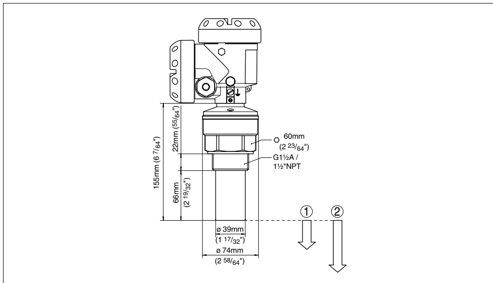
Рис. 23: OPTISOUND 3010 C
