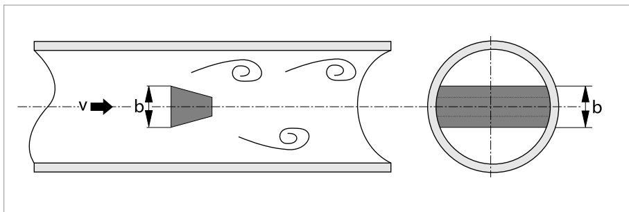
Рисунок 8-1: Принцип действия
