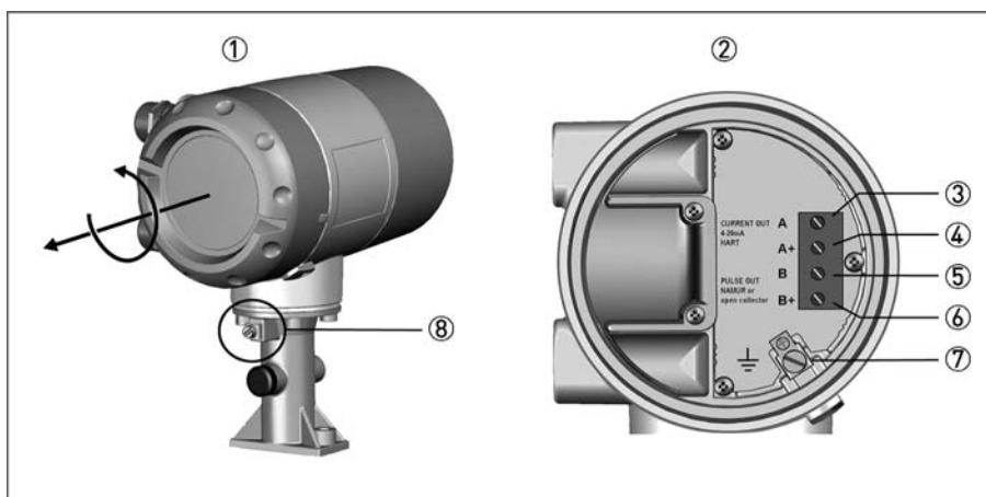
Рисунок 4-1: Корпус конвертера сигналов с крышкой
