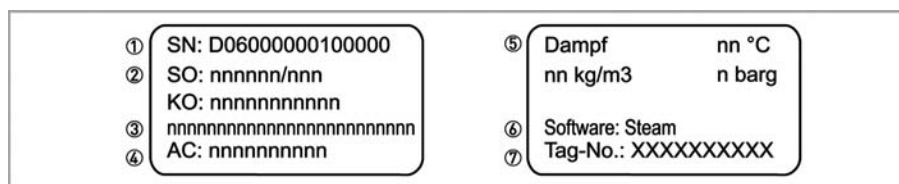
Рисунок 2-6: Пример шильды прибора
