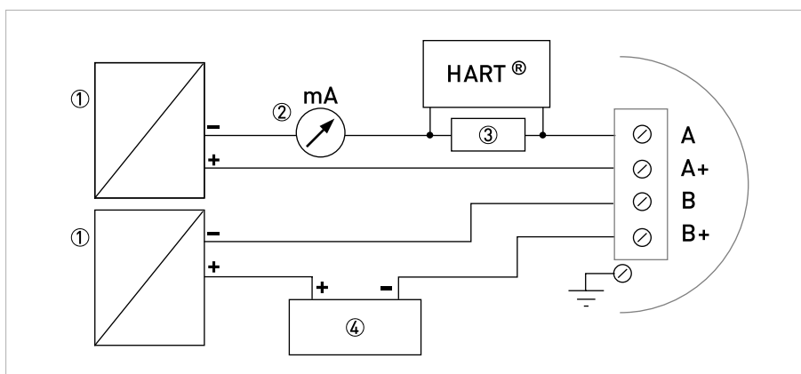
Рисунок 4-2: Подключение токового и импульсного выхода
