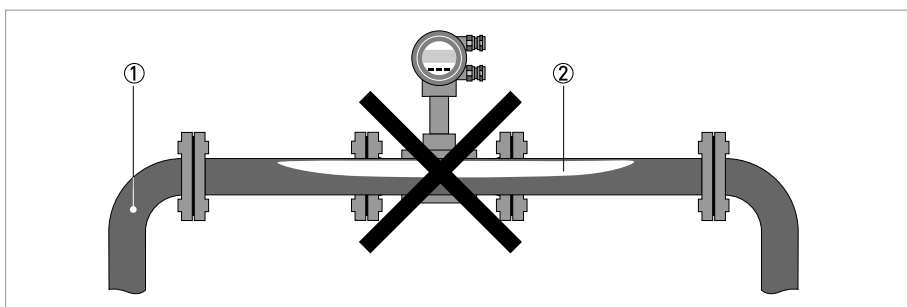
Рисунок 3-2: Восходящий изгиб трубы
