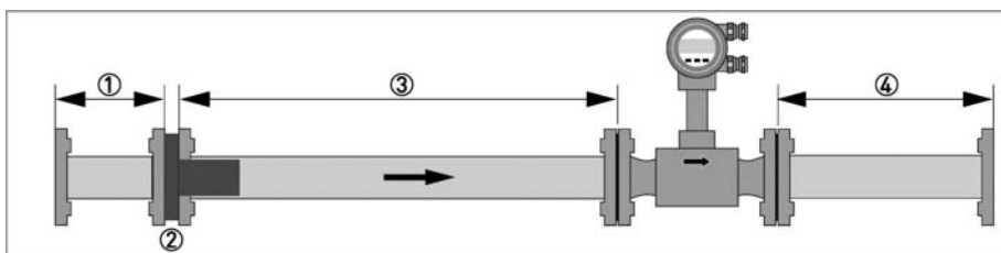
Рисунок 3-9: Струевыпрямитель
