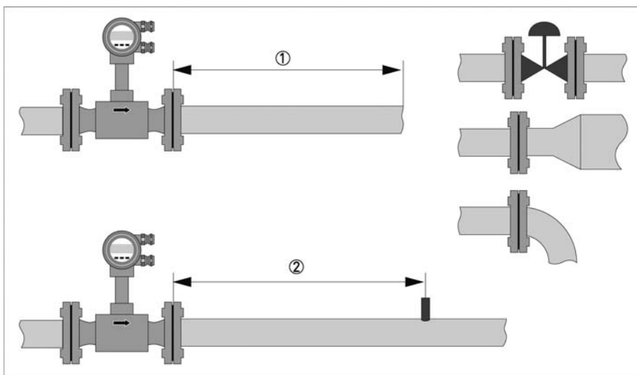
Рисунок 3-8: Минимальные выходные участки
