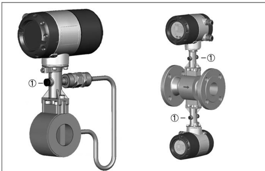
① Клапан оповещения (мембранный вентиляционный клапан)
