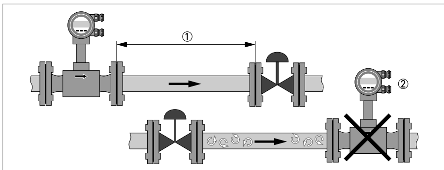
Рисунок 3-4: Трубопровод с регулирующим клапаном
