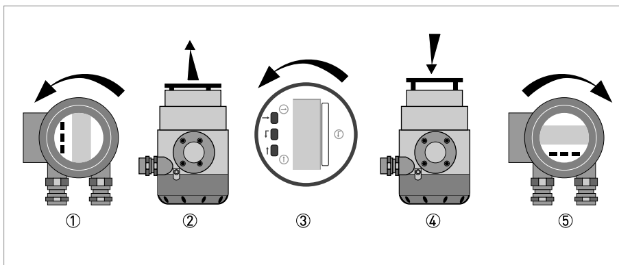
Рисунок 3-6: Поворот дисплея
