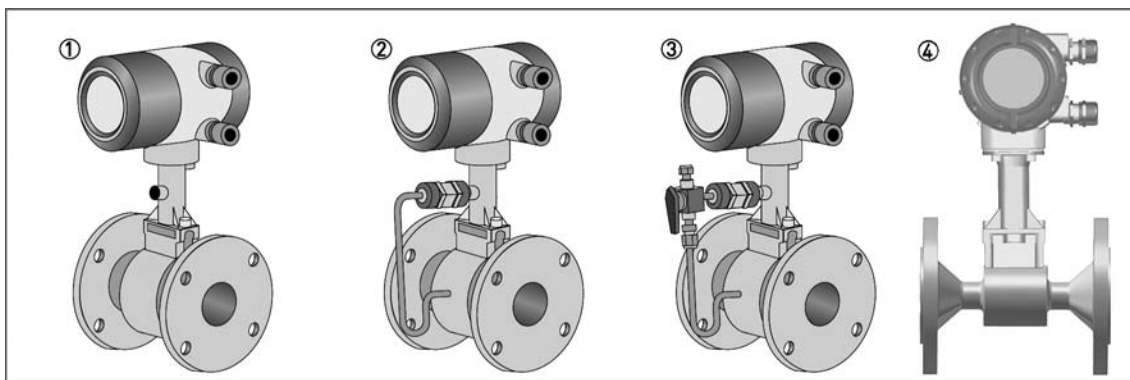
Рисунок 2-2: Приборы фланцевого исполнения с индикатором
