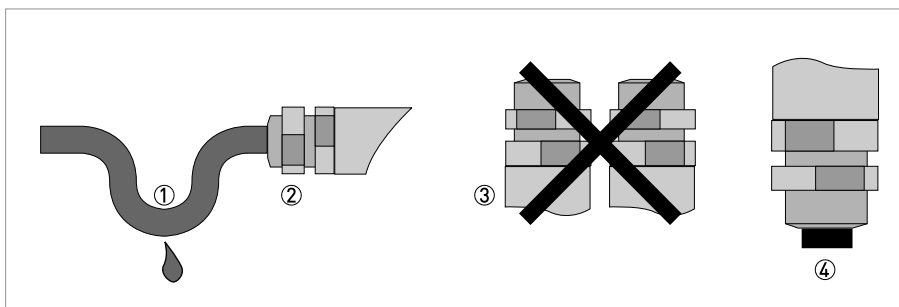
Рисунок 4-5: Кабельный ввод
