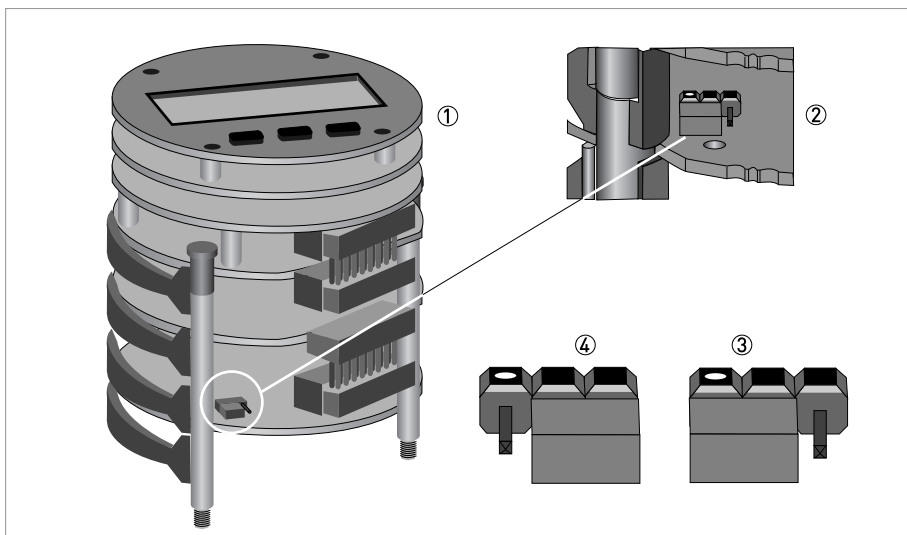
Рисунок 4-4: Положения перемычки импульсного выхода
