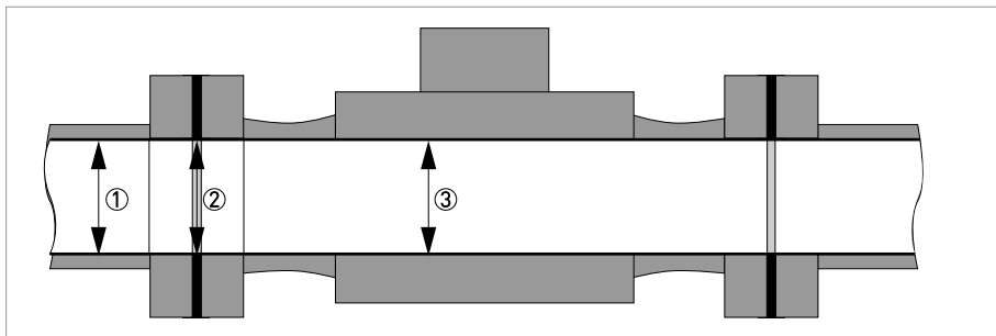
Рисунок 3-11: Внутренний диаметр
