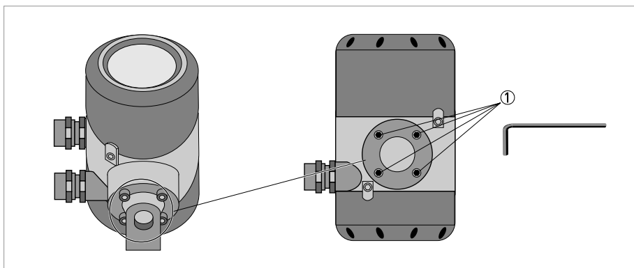
Рисунок 3-5: Винты с внутренним шестигранником на корпусе конвертера
