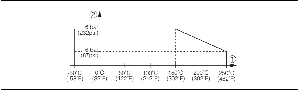
Рис. 14: Давление процесса - Температура продукта
