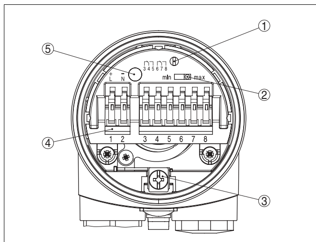
Рис. 12: Блок электроники VB 60R - релейный выход
