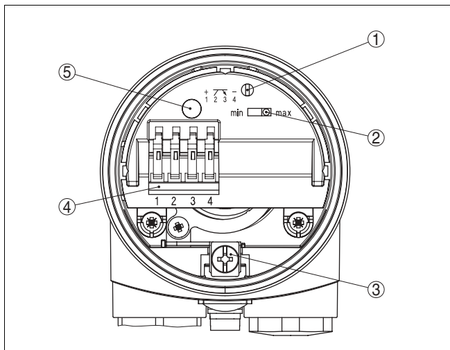
Рис. 14: Блок электроники VB 60T - транзисторный выход
