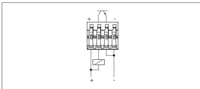
Рис. 12: Состояние NPN
