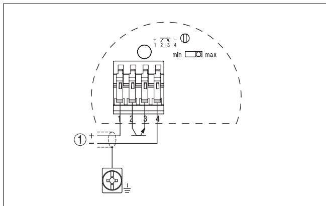
Рис. 11: Схема подключения
