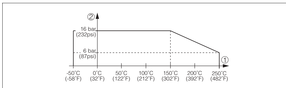
Рис. 17: Давление процесса - Температура продукта
