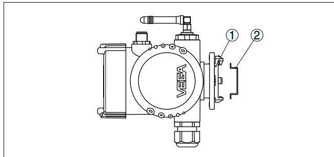
Рис. 3: PLICSMOBILE T61 для монтажа на несущей рейке
