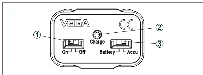
Рис. 8: Индикатор и элементы настройки аккумуляторного блока PLICSMOBILE
