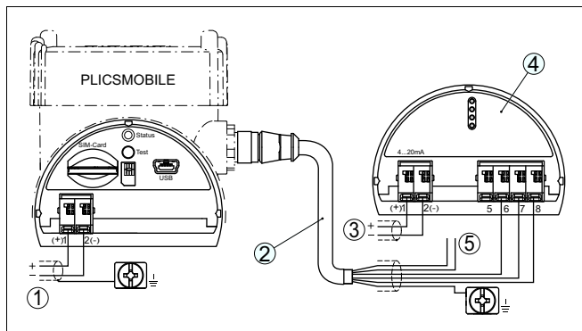
Рис. 7: Подключение источника питания в корпусе электроники
