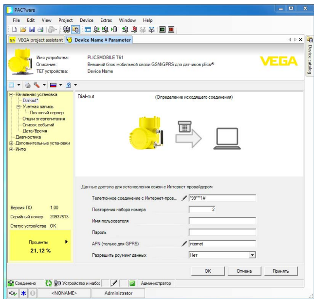
Рис. 13: Ввод данных доступа к Интернету
