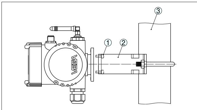
Рис. 4: PLICSMOBILE T61 для монтажа на стене
