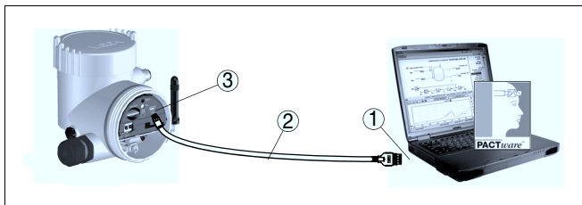
Рис. 11: Подключение ПК через USB
