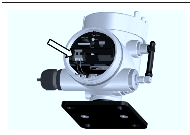
Рис. 5: Подключение: шаги 4 и 5
