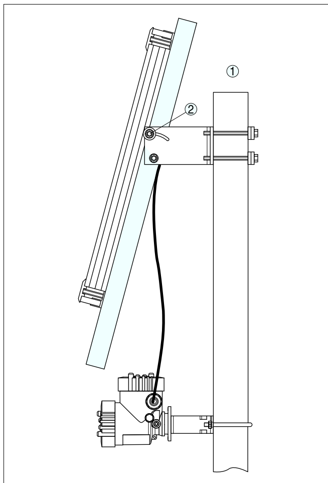
Рис. 9: Монтаж PLICSMOBILE на трубе, с солнечным модулем
