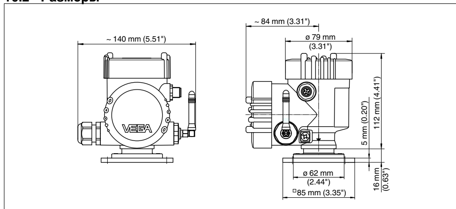
Рис. 15: Размеры PLICSMOBILE T61 с пластиковым корпусом
