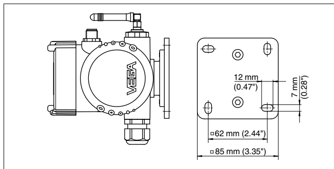
Рис. 2: PLICSMOBILE T61 для монтажа на стене. Монтажная панель - вид снизу.
