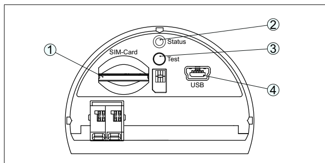
Рис. 10: Элементы индикации и настройки
