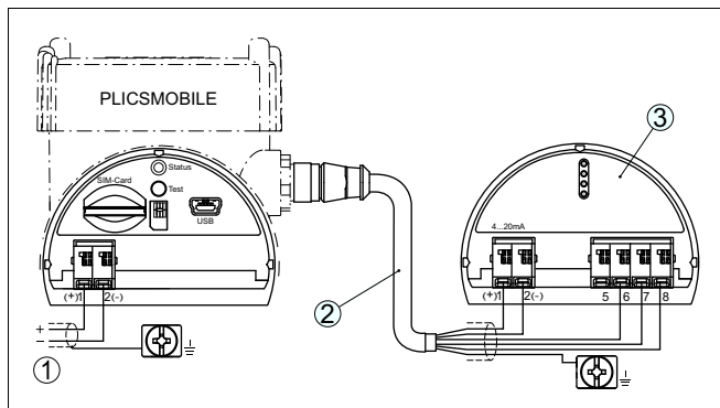
Рис. 6: Подключение источника питания в корпусе электроники
