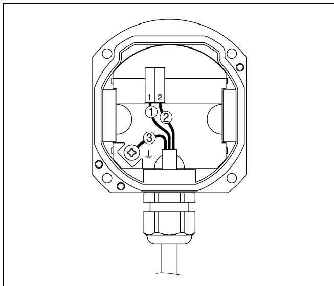
Рис. 10: Подключение выхода 4 ... 20 мА в цоколе корпуса
