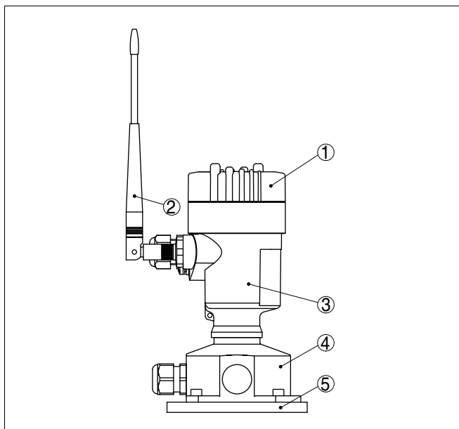
Рис. 1: PLICSRADIO R61
