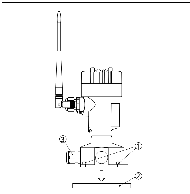
Рис. 7: Снятие монтажной пластины с цоколя корпуса
