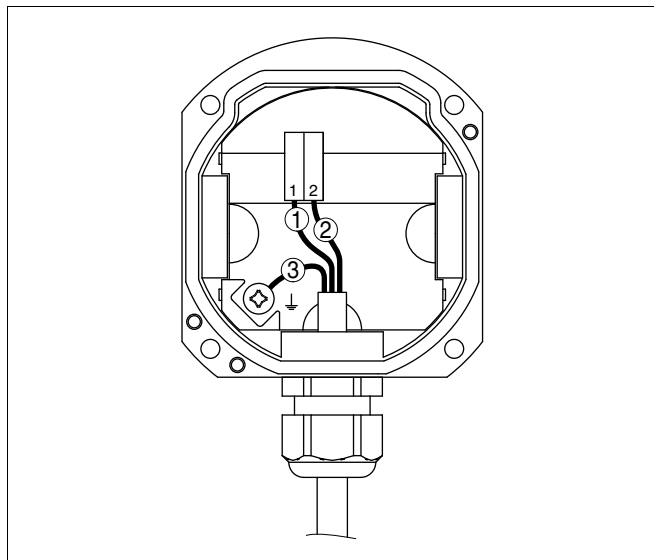
Рис. 10: Подключение соединения с C62 в цоколе корпуса
