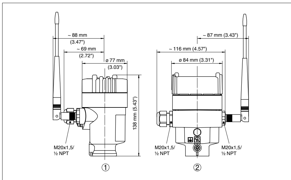
Рис. 15: Корпус с электроникой: с установленным модулем PLICSCOM пластиковый корпус выше на 11 мм (0.43 in), а алюминиевый - на 9 мм (0.35 in)
