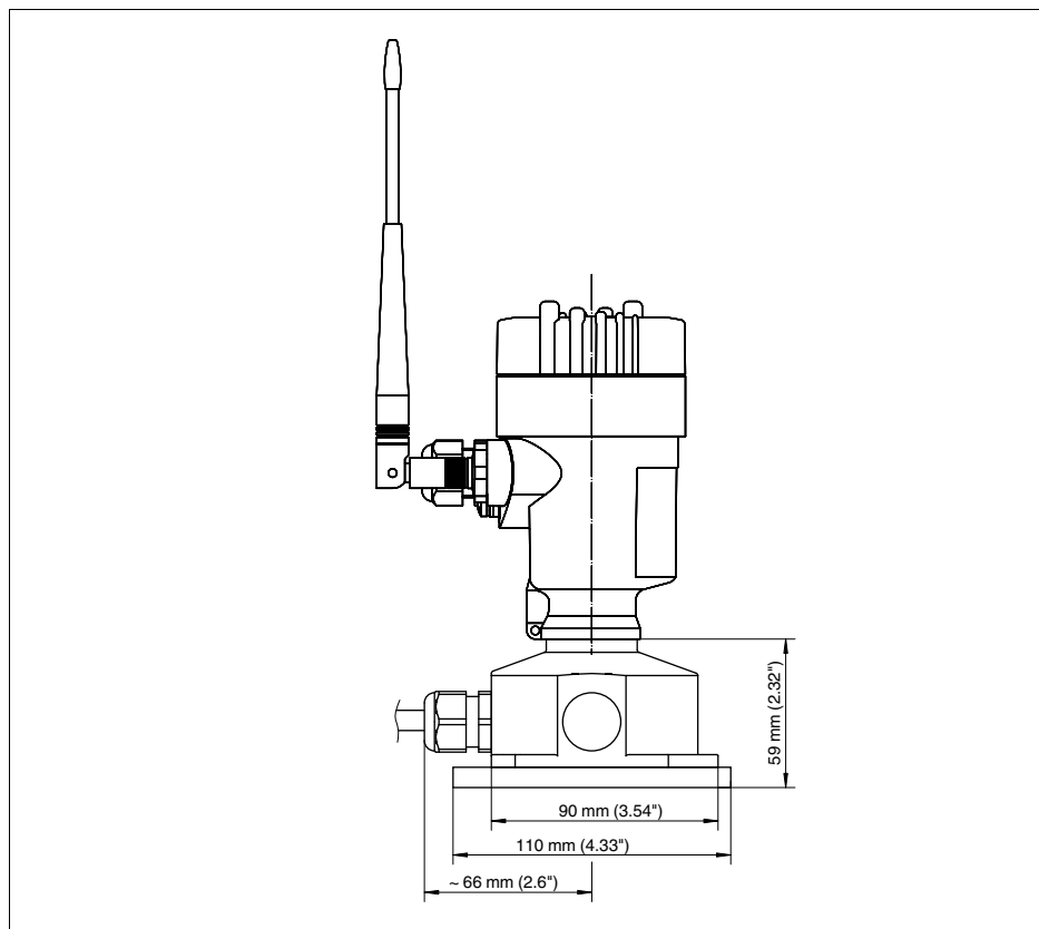
Рис. 16: Цоколь корпуса с отсеком подключения
