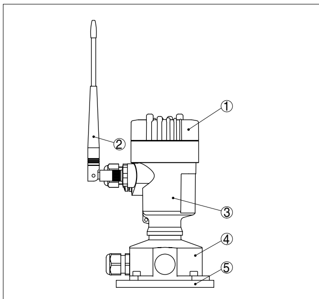
Рис. 1: PLICSRADIO R62
