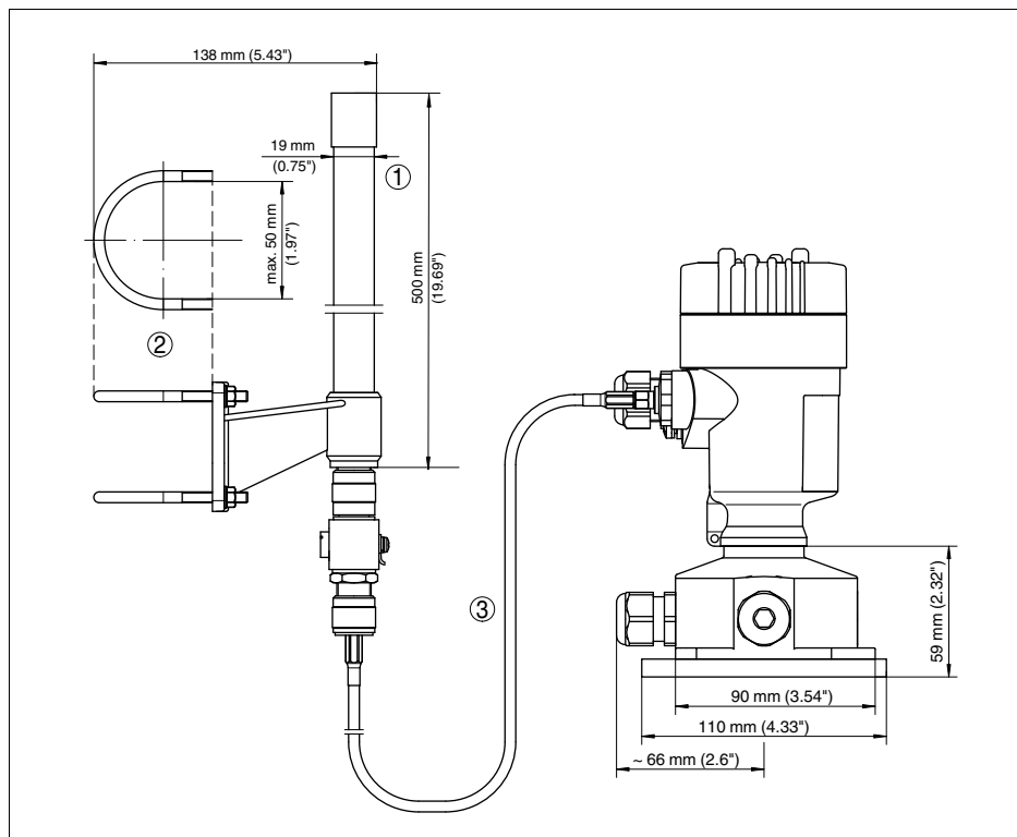
Рис. 17: Выносная антенна
