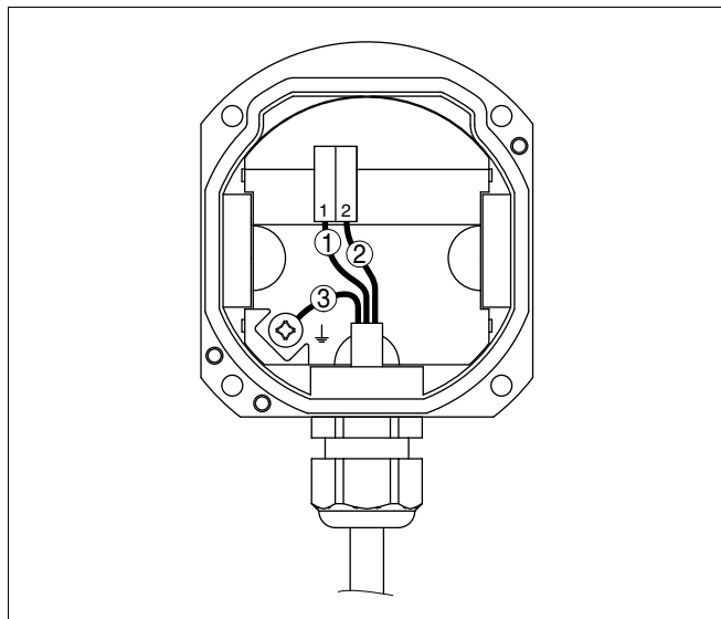
Рис. 10: Подключение датчика в цоколе выносного корпуса
