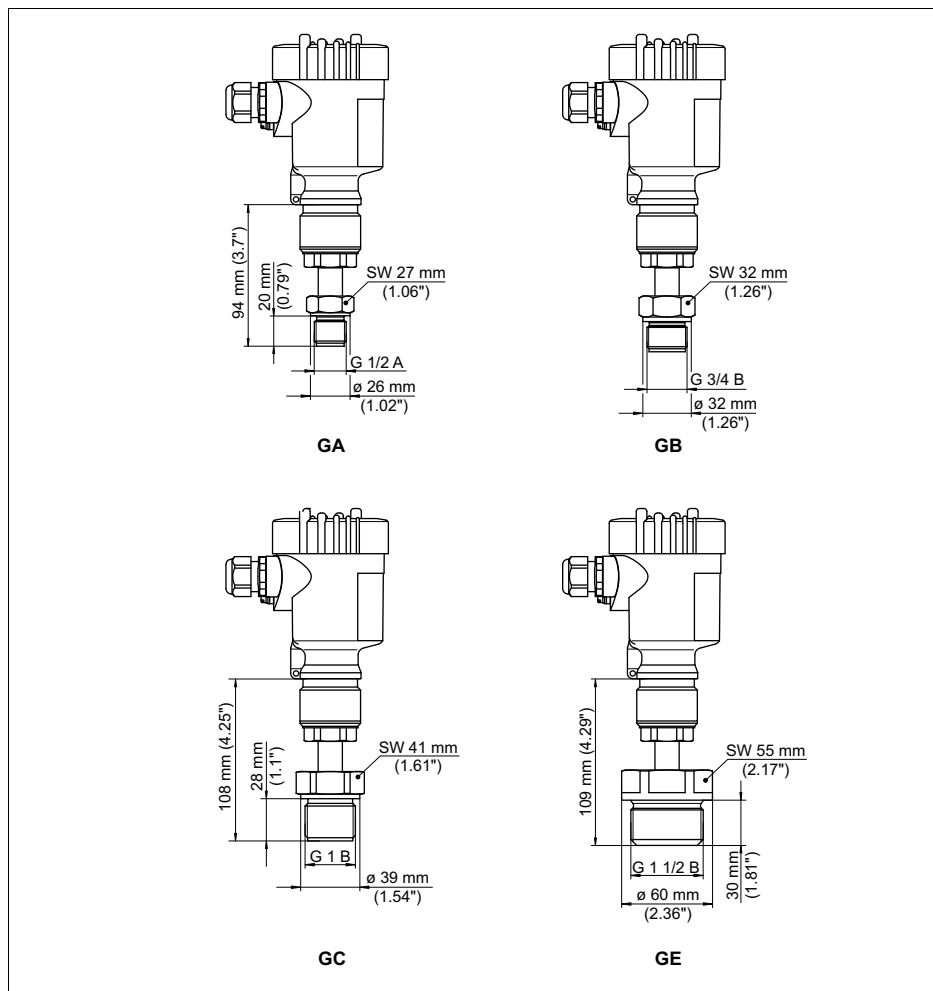
Рис. 44: VEGABAR 51 - резьбовое исполнение, GA = G 1/2 A по ISO 228-1, GB = G 3/4 A по DIN 3852-E, GC = G 1 A по DIN 3852-E, GD = G 1 1/2 A по DIN 3852-A
