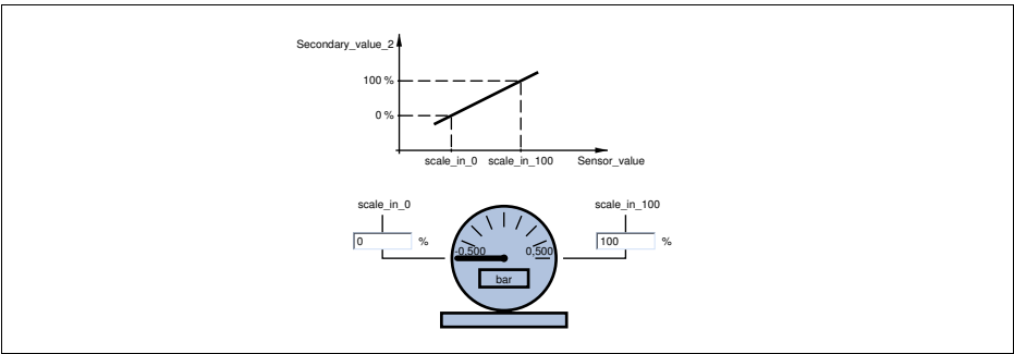
Рис. 29: Установка VEGABAR 51
