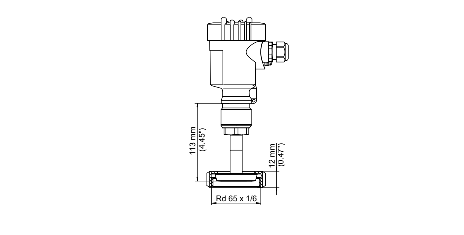
Рис. 41: VEGABAR 51 - Накидная гайка соотв. DIN 11851
