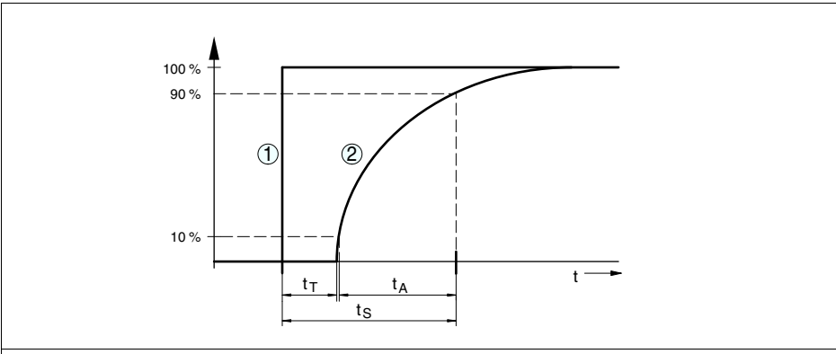
Рис. 26: Скачкообразное изменение параметров процесса, время нечувствительности t_T , время нарастания t_A и время реакции на скачок t_S
