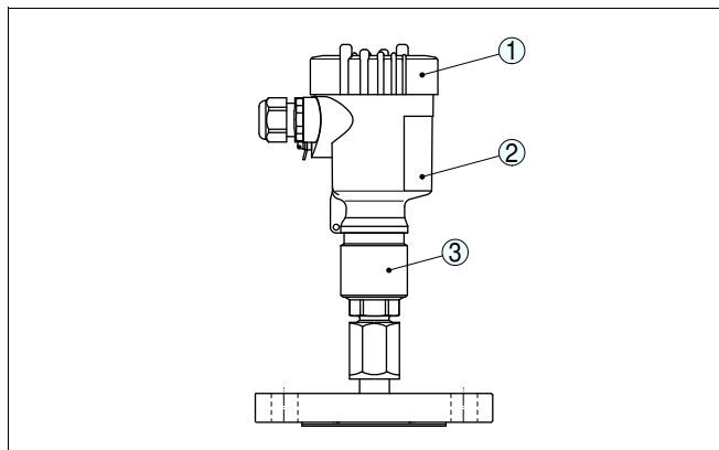
Рис. 1: VEGABAR 51 с фланцевым присоединением DN 50 PN 40 и пластиковым корпусом
