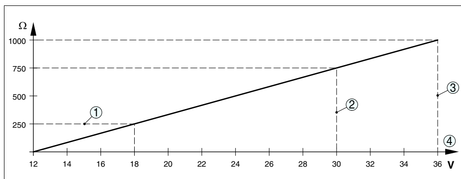
Рис. 29: Диаграмма напряжения
