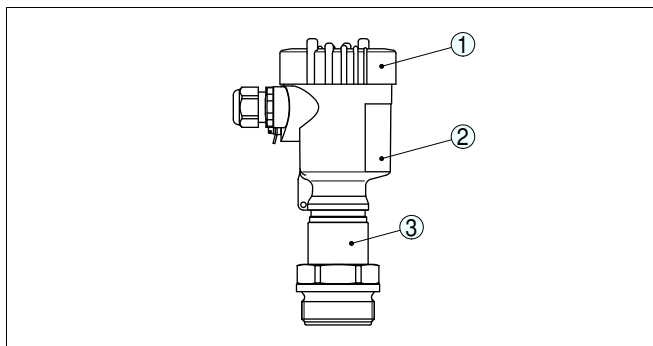
Рис. 1: VEGABAR 55 с резьбовым присоединением G1½ А и пластиковым корпусом
