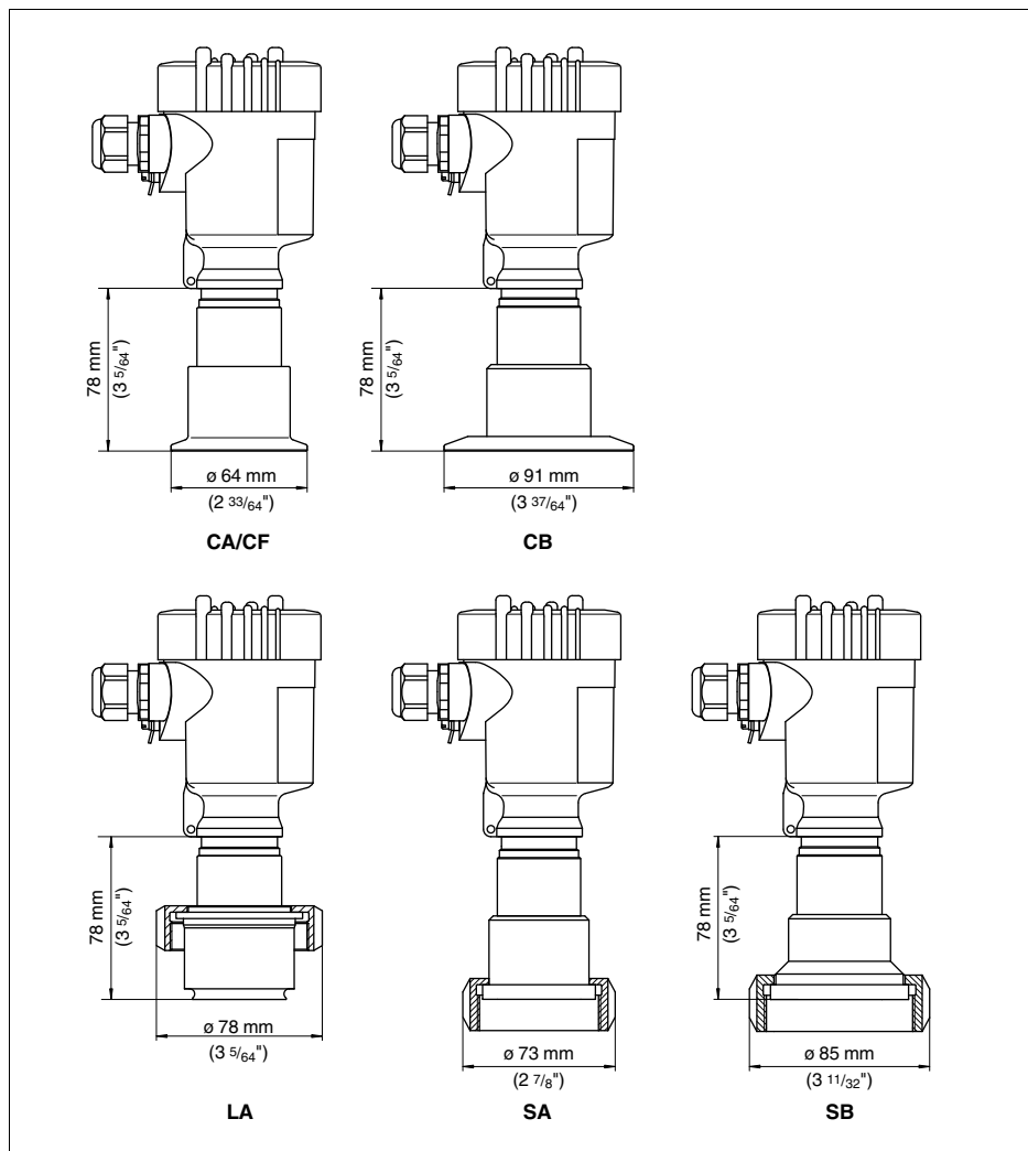
Рис. 37: VEGABAR 55, гигиеническое присоединение: CA/CF = зажим 2"/зажим 2 1/2" по DIN 32676, ISO 2852/316L CB = зажим 3", LA = гигиеническое присоединение со шлицевой накидной гайкой F40, SA = SMS DN 38, SB = SMS DN 51
