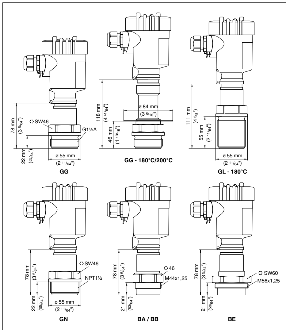
Рис. 27: VEGABAR 55, с резьбовым присоединением: GG = G1 1/2 A, GL = G1 1/2 A длина резьбы 55 мм, GN = 1 1/2 NPT, BA/BB = M44 x 1,25, BE = M56 x 1,25
