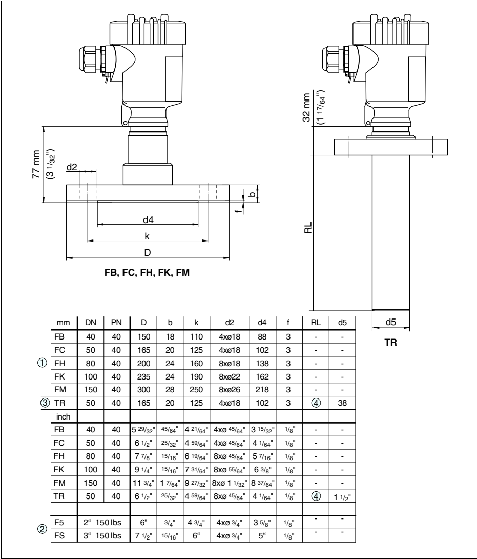
Рис. 30: VEGABAR 55 с фланцевым присоединением
