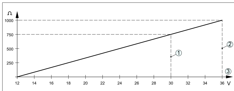
Рис. 20: Диаграмма напряжения
