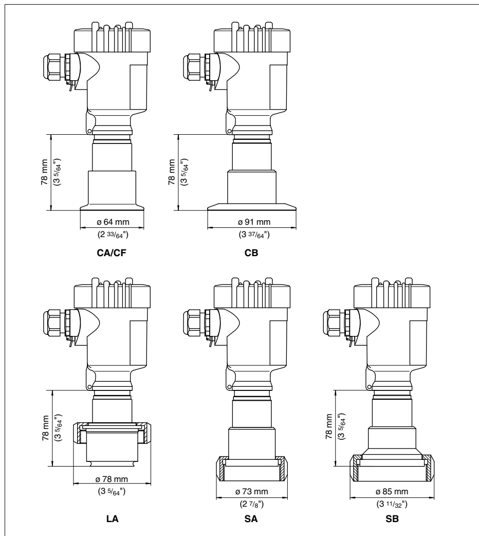
Рис. 28: VEGABAR 55, гигиеническое присоединение: CA/CF = зажим 2"/зажим 2 1/2" по DIN 32676, ISO 2852/316L CB = зажим 3", LA = гигиеническое присоединение со шлицевой накидной гайкой F40, SA = SMS DN 38, SB = SMS DN 51
