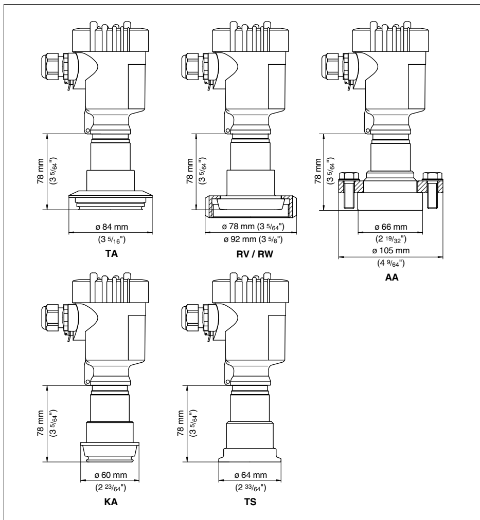
Рис. 29: VEGABAR 55, с гигиеническим присоединением: TA = Tuchenhausen Varivent DN 32, RV/RW = накидная гайка DN 40/DN 50 по DIN 11851, AA = DRD, KA = конус DN 40, TS = зажимный штуцер соотв. DIN 11864-3 форма A DN40/PN40
