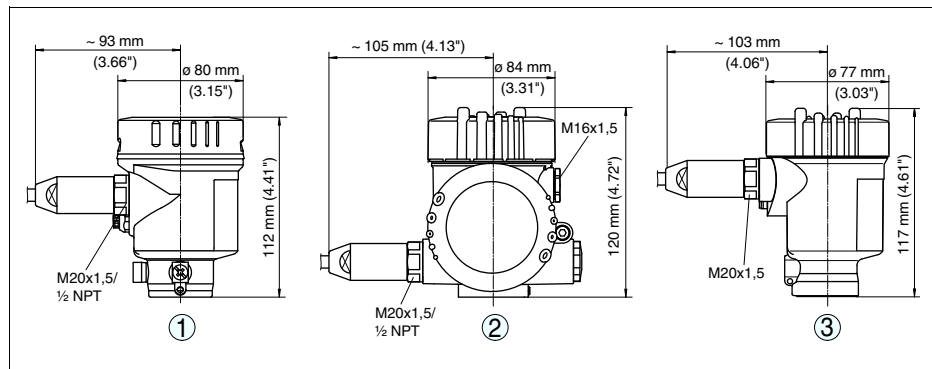
Рис. 25: Корпуса в исполнении IP 66/IP 68 (1 bar) - с установленным модулем индикации и настройки корпус выше на 9 mm/0.35 in
