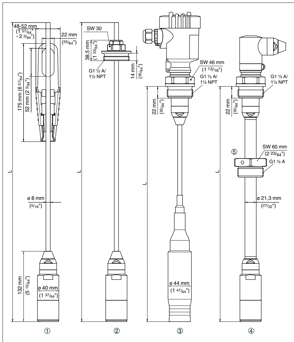
Рис. 41: VEGABAR 66 в стандартном исполнении
