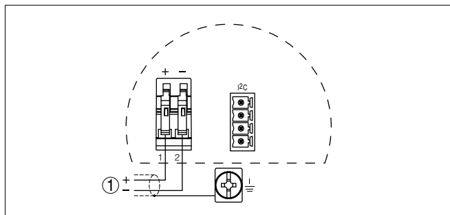
Рис. 18: Схема подключения (двухкамерный корпус)
