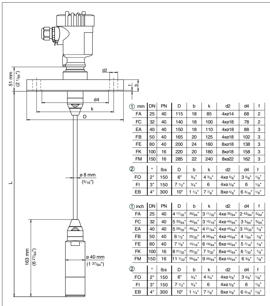
Рис. 42: VEGABAR 67 - фланцевое присоединение
