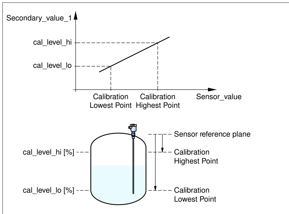
Рис. 26: Установка VEGACAL 63
