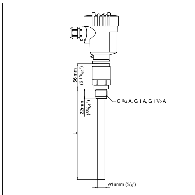
Рис. 29: VEGACAL 63 - Резьбовое исполнение G1 A (ISO 228 T1)
