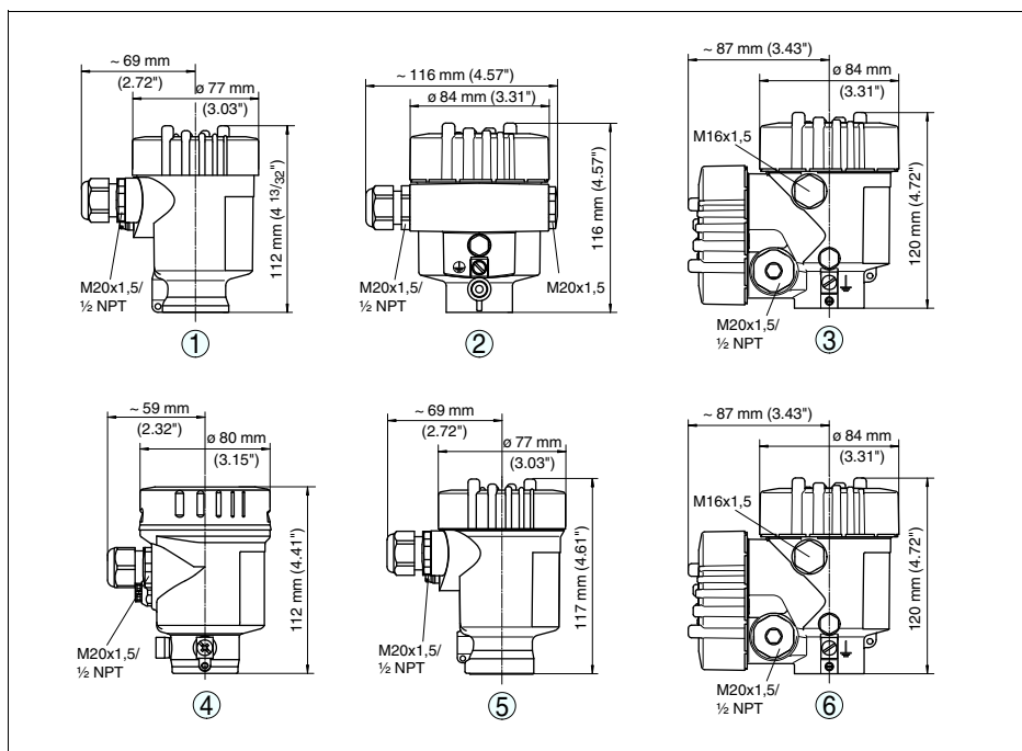
Рис. 27: Корпуса в исполнении IP 66/IP 68 (0,2 bar) - с установленным модулем индикации и настройки корпус выше на 9 мм/0.35 in
