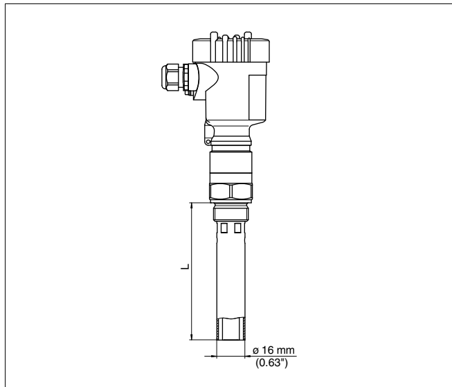
Рис. 19: VEGACAL 63 с концентрической трубой (например, при малом значении диэлектрической постоянной или для линеаризации)
