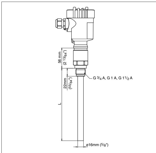
Рис. 17: VEGACAL 63 - Резьбовое исполнение G1 A (ISO 228 T1)
