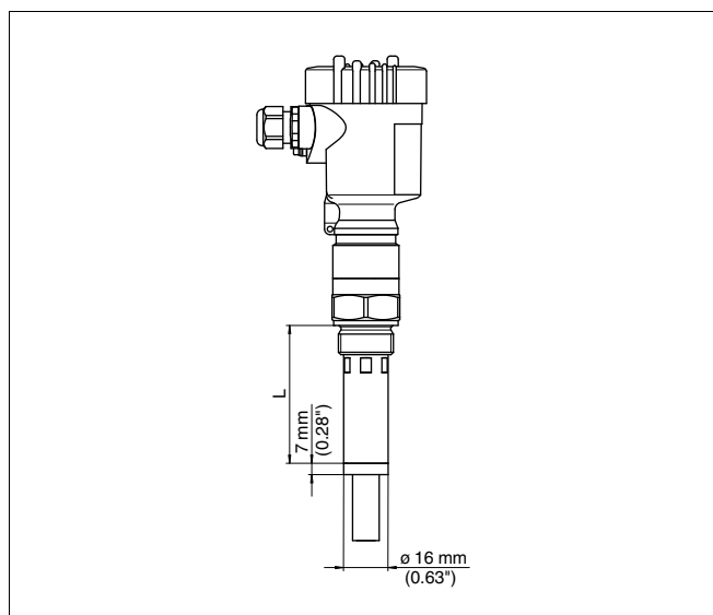
Рис. 33: VEGACAL 65 с экранирующей трубой (например, для защиты от конденсата)
