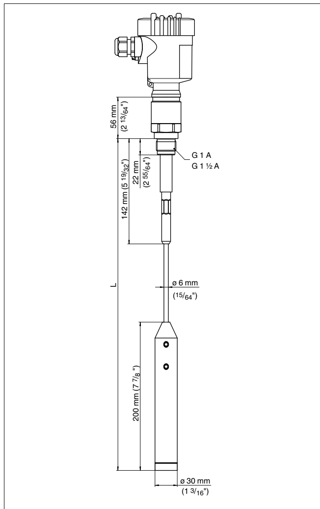
Рис. 30: VEGACAL 65 - тросовое исполнение \varnothing 6 мм, резьба G1 A (ISO 228 T1)
