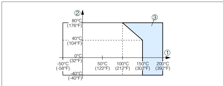
Рис. 25: Температура окружающей среды - Температура процесса
