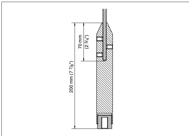
Рис. 24: При укорачивании троса следует учитывать наличие натяжного груза.
