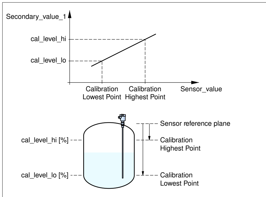
Рис. 27: Установка VEGACAL 65
