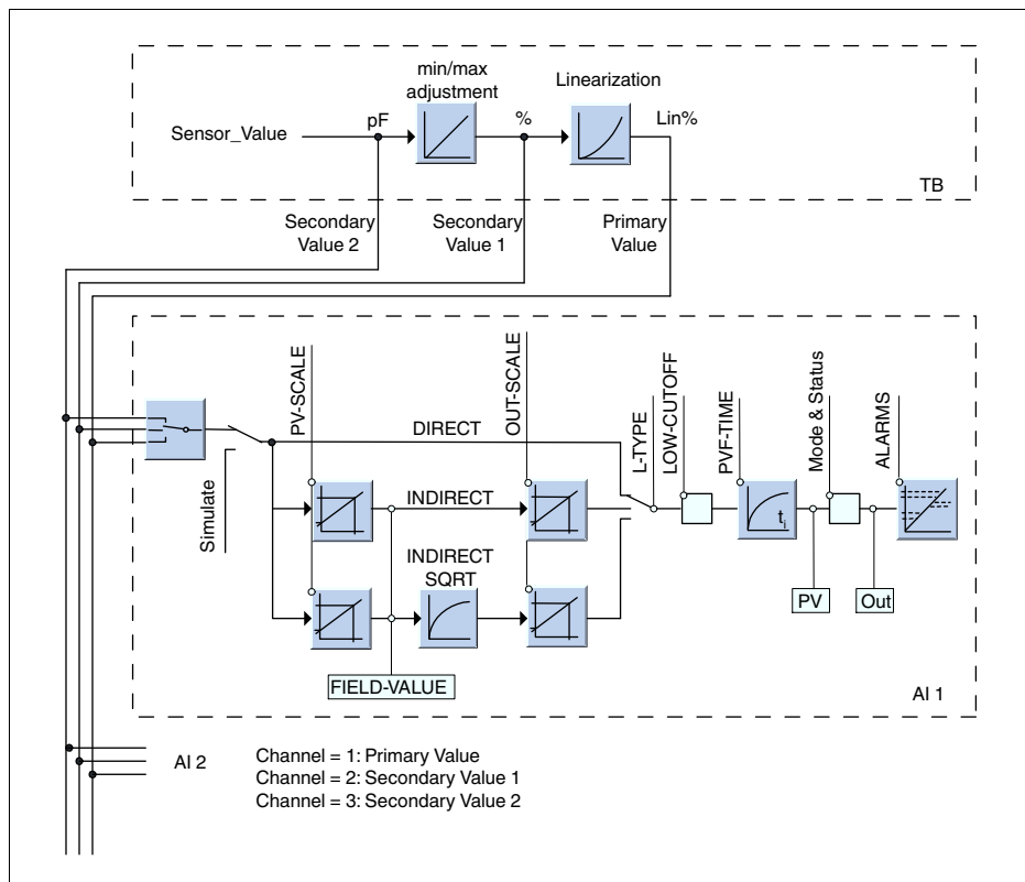
Рис. 26: Обработка измеренных значений VEGACAL 65
