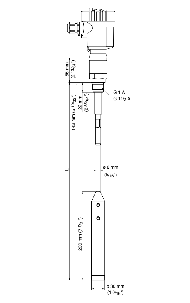
Рис. 31: VEGACAL 65 - тросовое исполнение \varnothing 8 мм, резьба G 1 A (ISO 228 T1)
