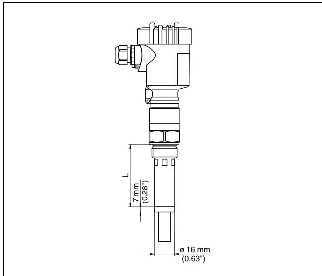
Рис. 36: VEGACAL 65 с экранирующей трубой (например, для защиты от конденсата)
