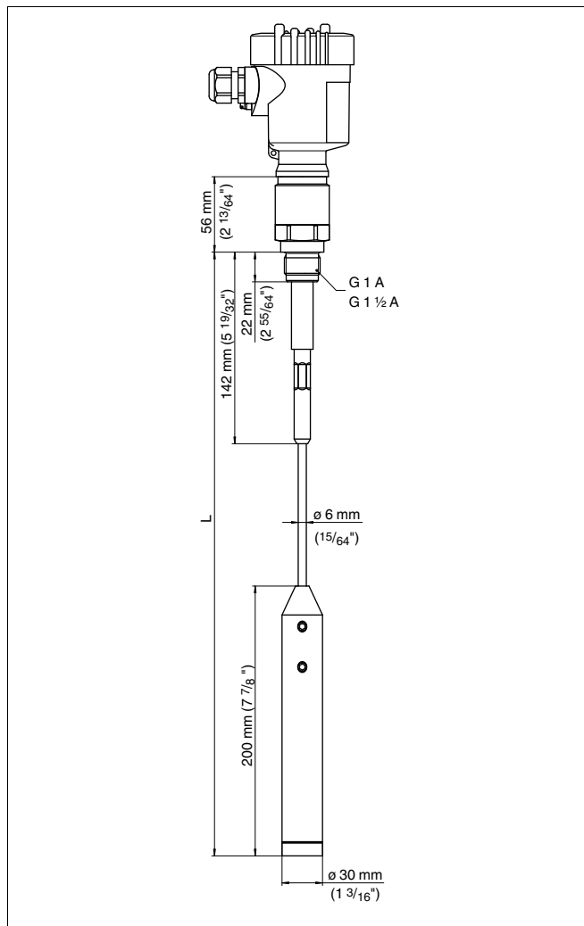
Рис. 33: VEGACAL 65 - тросовое исполнение \varnothing 6 мм, резьба G1 A (ISO 228 T1)
