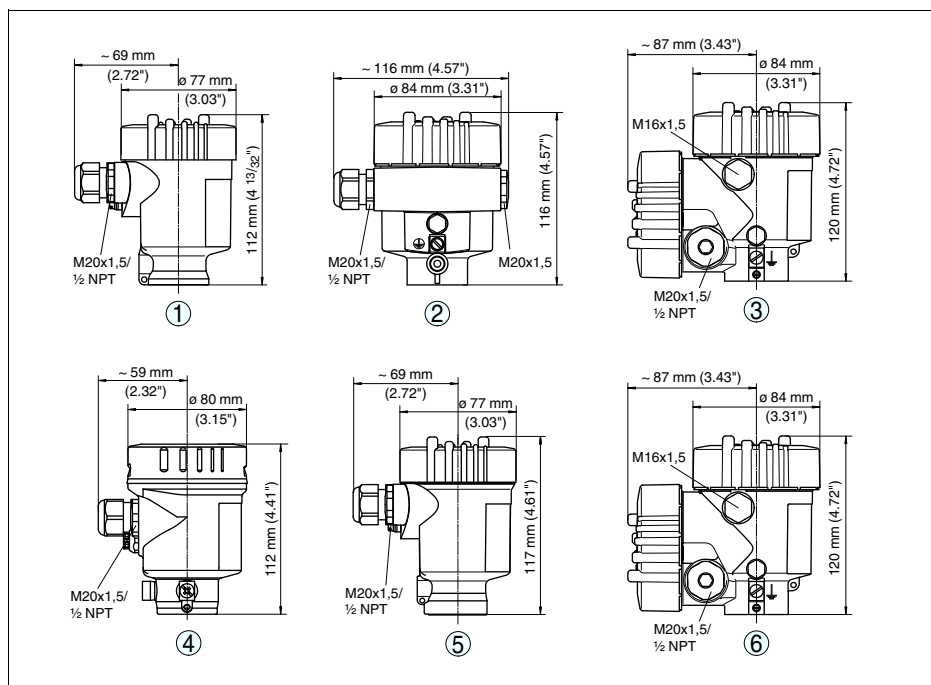
Рис. 31: Корпуса в исполнении IP 66/IP 68 (0,2 bar) - с установленным модулем индикации и настройки корпус выше на 9 mm/0.35 in
