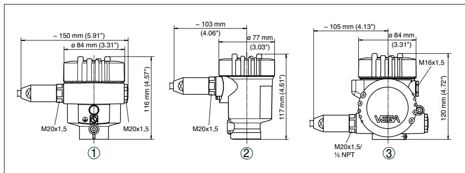
Рис. 32: Корпуса в исполнении IP 66/IP 68 (1 bar) - с установленным модулем индикации и настройки корпус выше на 9 mm/0.35 in
