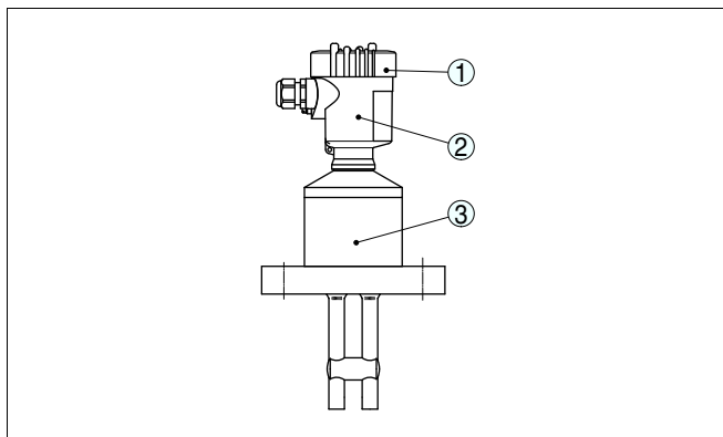
Рис. 1: VEGACAP 69 - с пластиковым корпусом
