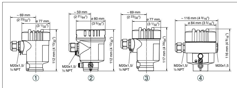
Рис. 31: Исполнения корпуса
