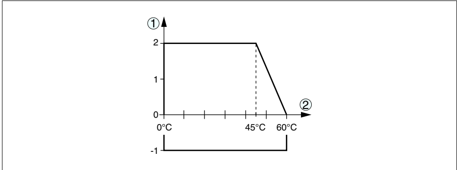
Рис. 30: Давление процесса - Температура процесса (фланец PP)
