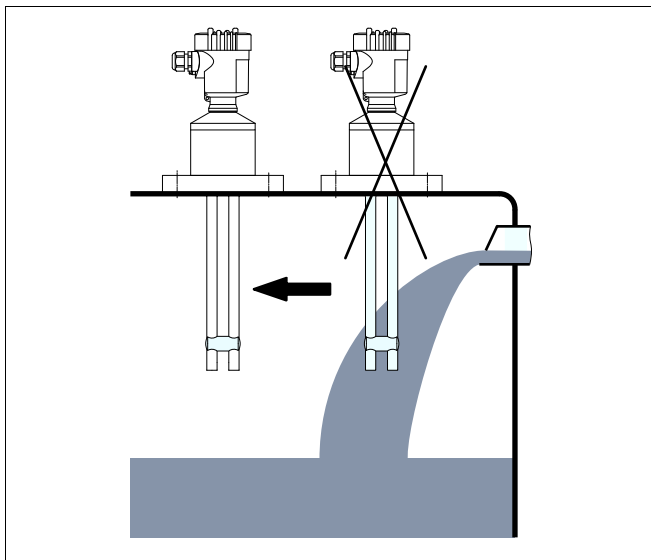
Рис. 4: Втекающий продукт
