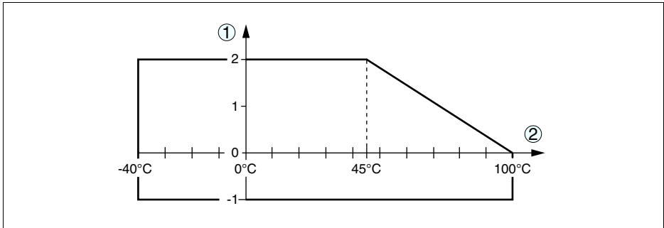
Рис. 29: Давление процесса - Температура процесса (фланец PTFE)
