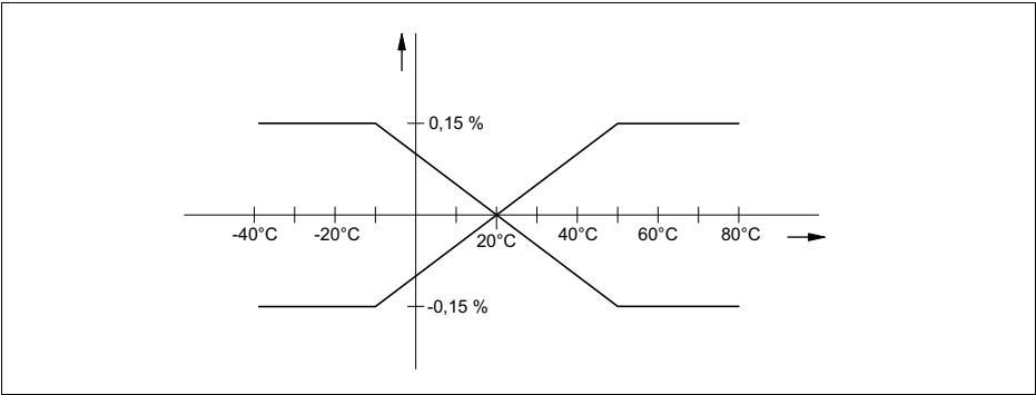
Рис. 59: Термическое изменение токового выхода
