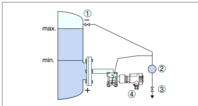
Рис. 23: Схема для измерения уровня в закрытой емкости
