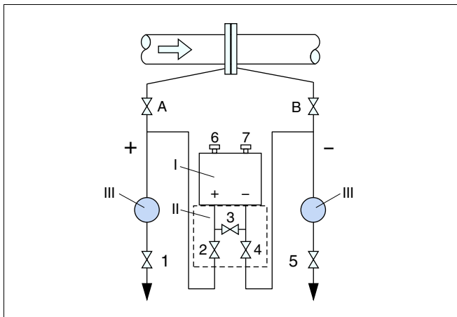
Рис. 52: Предпочтительная схема установки для измерения на жидкостях
