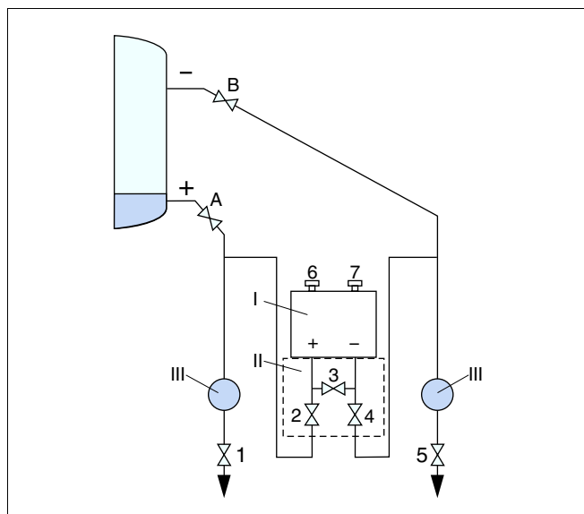
Рис. 54: Предпочтительная схема установки для измерения в закрытой емкости
