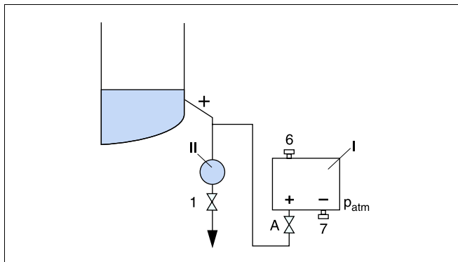
Рис. 53: Предпочтительная схема установки для измерения в открытой емкости
