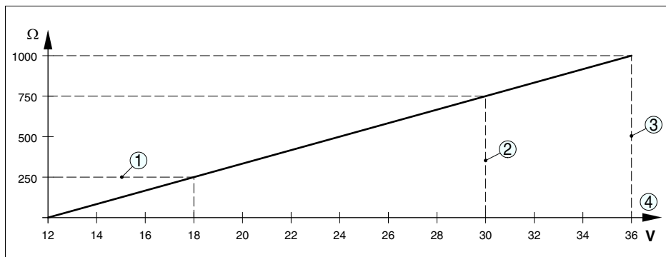
Рис. 60: Диаграмма напряжения
