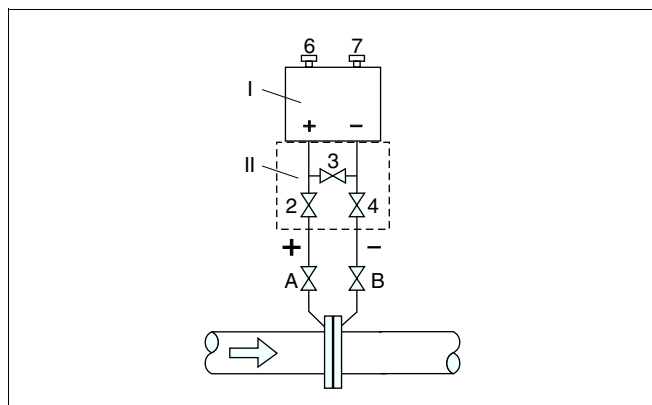
Рис. 50: Предпочтительная схема установки для измерения на газах
