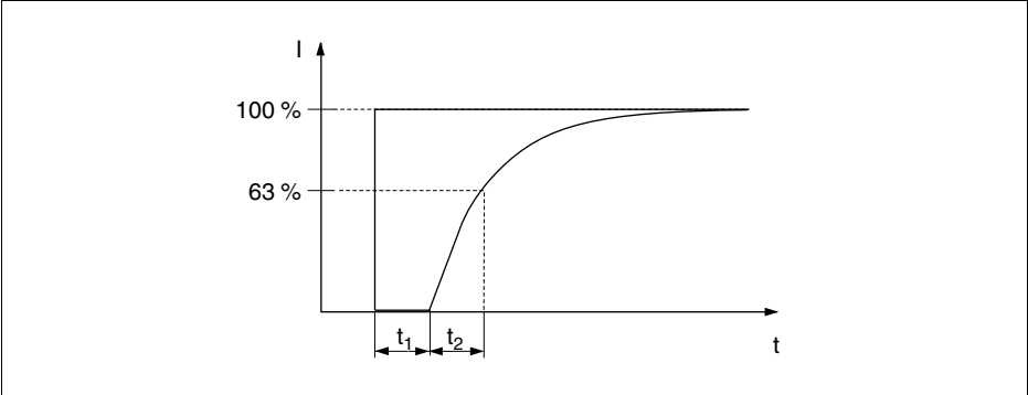
Рис. 58: Время нечувствительности t_1 и постоянная времени t_2
