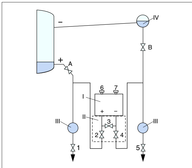
Рис. 55: Предпочтительная схема установки для измерения в закрытых емкостях с наличием парового слоя
