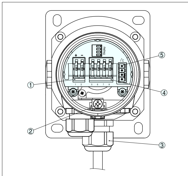
Рис. 42: Отсек электроники и подключения
