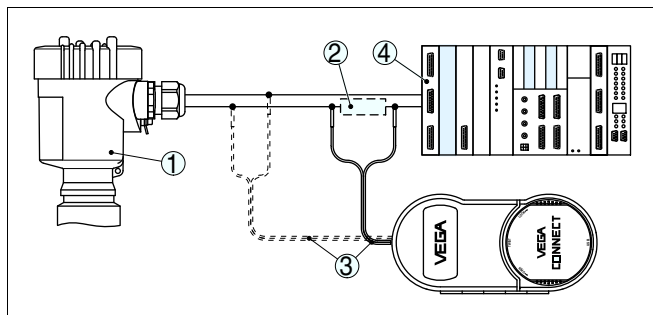
Рис. 49: Подключение ПК к сигнальному кабелю через HART
