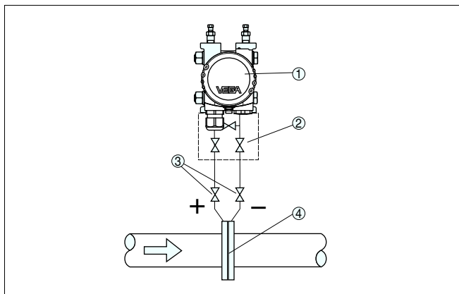
Рис. 16: Схема установки для измерения расхода на газах, подключение через 3-вентильный блок
