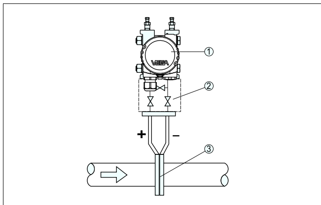
Рис. 17: Схема установки для измерения расхода на газах, подключение через 3-вентильный блок с фланцевым присоединением с обеих сторон
