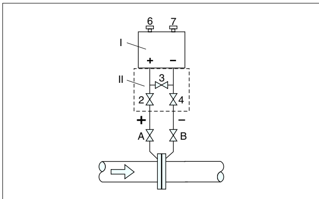
Рис. 56: Предпочтительная схема установки для измерения на газах
