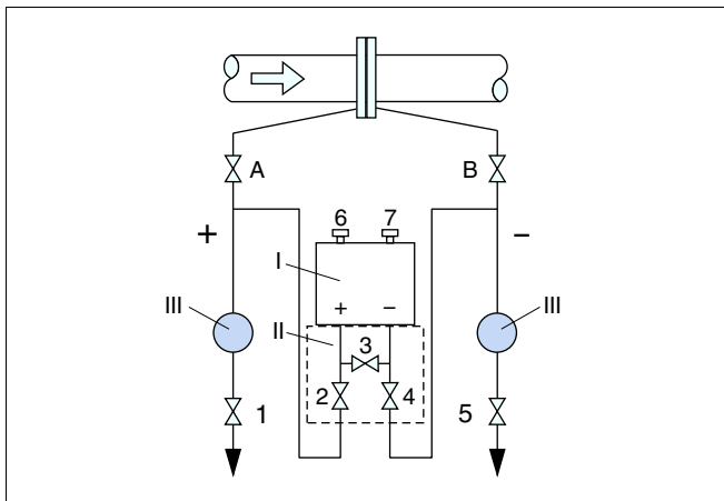
Рис. 57: Предпочтительная схема установки для измерения на жидкостях
