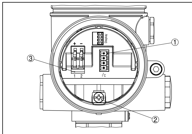
Рис. 26: Отсек подключения (двухкамерный корпус)
