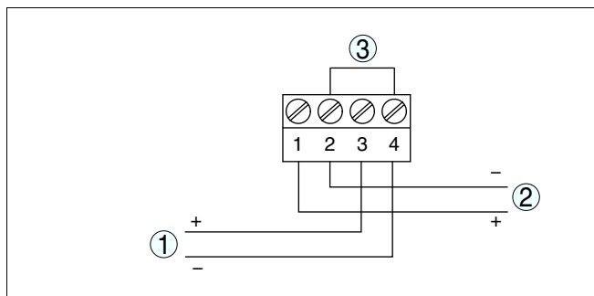
Рис. 4: Схема подключения VEGADIS 175 к пассивным датчикам
