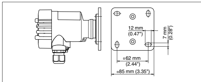
Рис. 6: VEGADIS 61 для монтажа на стене. Монтажная панель - вид снизу.
