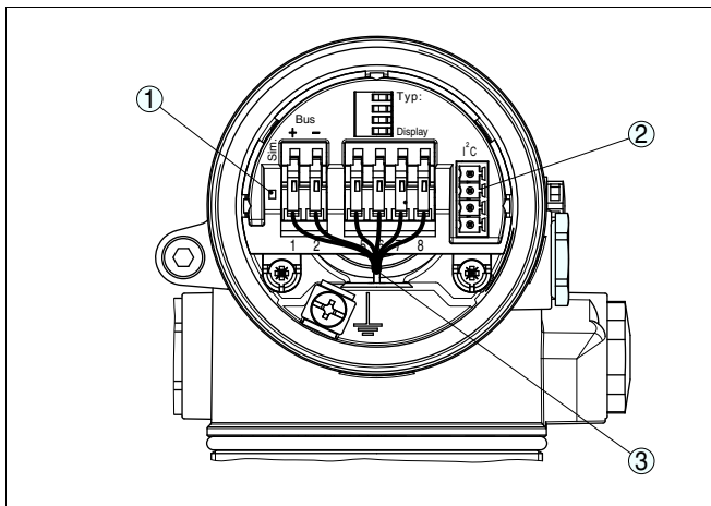
Рис. 10: Отсек электроники в двухкамерном корпусе
