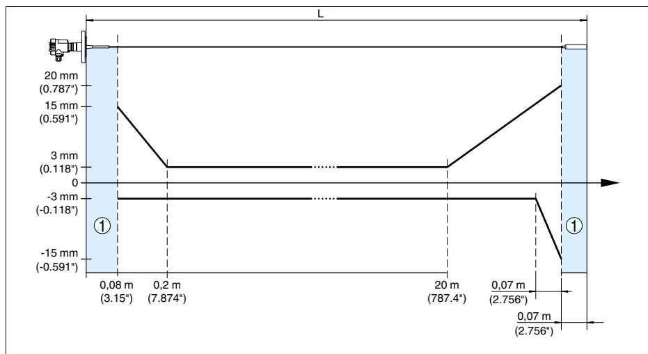
Рис. 23: Погрешность измерения VEGAFLEX 63 в тросовом исполнении, длина зонда L > 20 м (продукт - вода)
