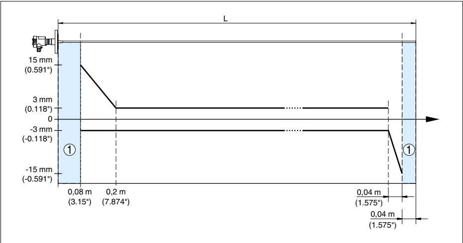
Рис. 19: Погрешность измерения VEGAFLEX 63 в стержневом исполнении (продукт - вода)
