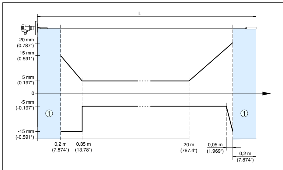
Рис. 24: Погрешность измерения VEGAFLEX 63 в тросовом исполнении, длина зонда L > 20 м (продукт - масло)
