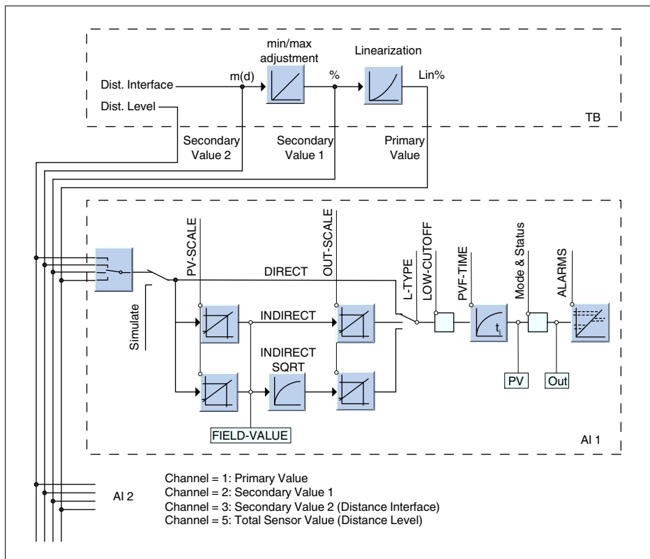
Рис. 26: Обработка измеренных значений VEGAFLEX 63
