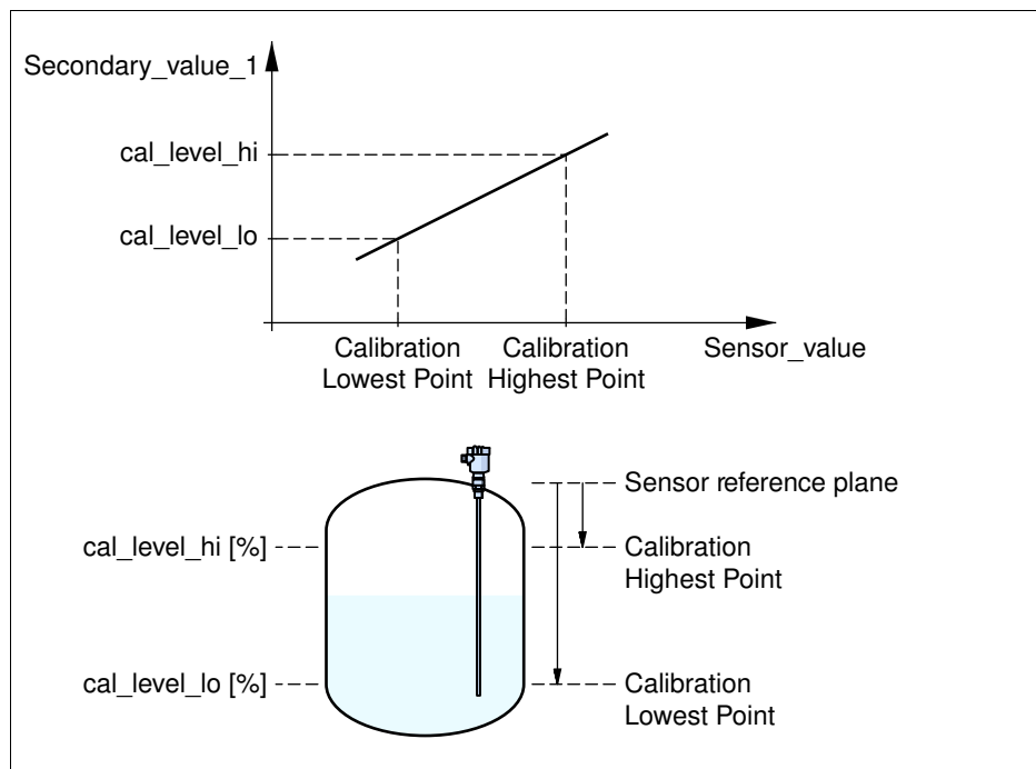
Рис. 27: Установка VEGAFLEX 63
