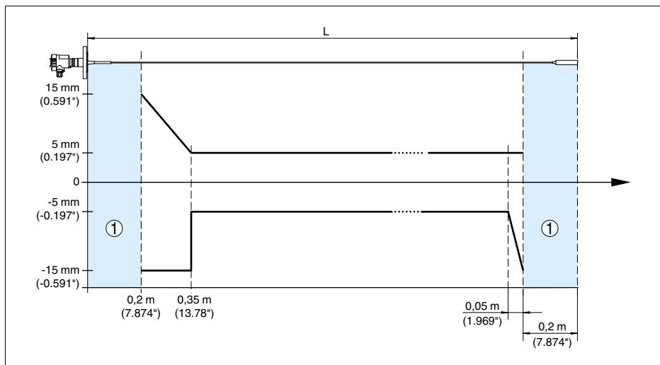
Рис. 22: Погрешность измерения VEGAFLEX 63 в тросовом исполнении, длина зонда L < 20 м (продукт - масло)
