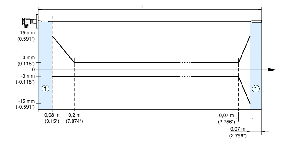
Рис. 21: Погрешность измерения VEGAFLEX 63 в тросовом исполнении, длина зонда L < 20 м (продукт - вода)
