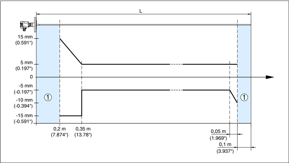
Рис. 20: Погрешность измерения VEGAFLEX 63 в стержневом исполнении (продукт - масло)
