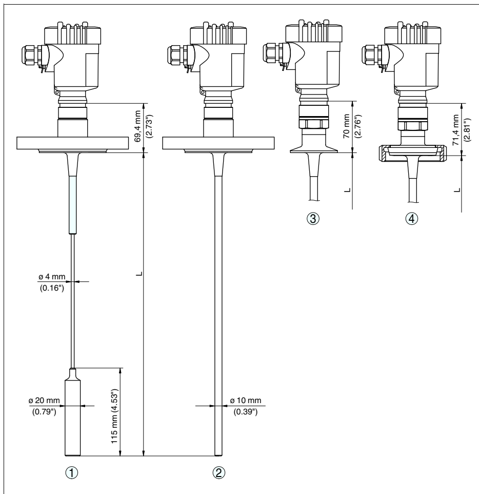
Рис. 32: VEGAFLEX 63 во фланцевом исполнении
