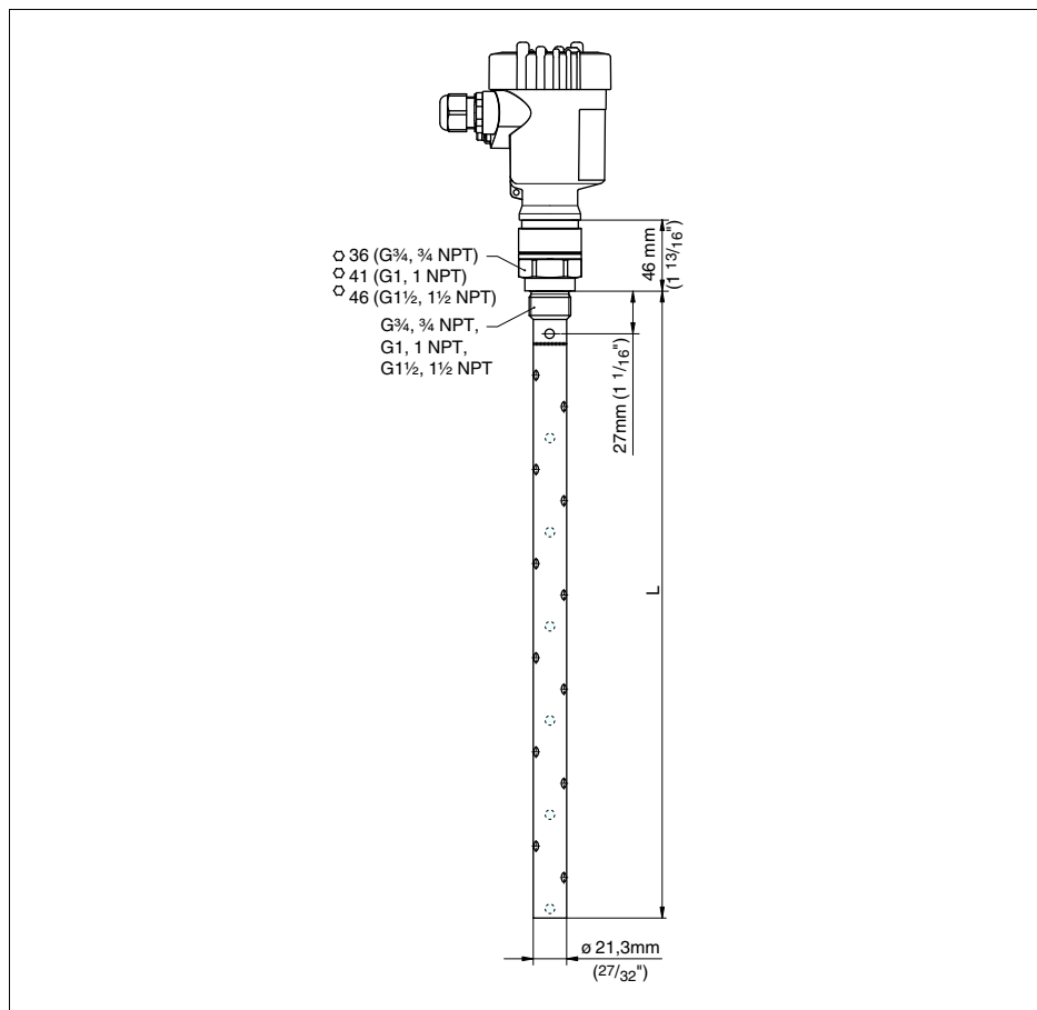
Рис. 26: VEGAFLEX 65, резьбовое исполнение
