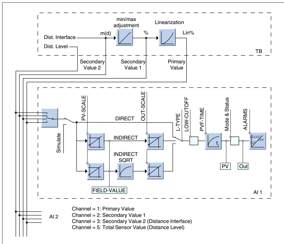
Рис. 20: Обработка измеренных значений VEGAFLEX 65
