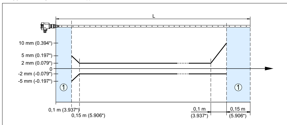
Рис. 18: Погрешность измерения VEGAFLEX 65 в коаксиальном исполнении (продукт - масло)
