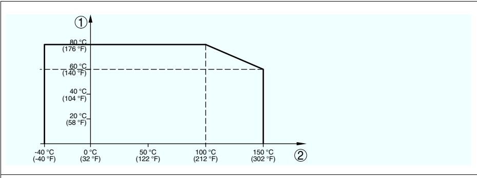
Рис. 19: Температура окружающей среды - Температура процесса 1 Температура окружающей среды 2 Температура процесса (в зависимости от материала уплотнения)
