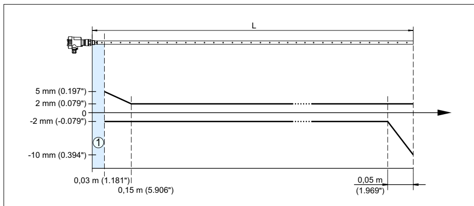
Рис. 17: Погрешность измерения VEGAFLEX 65 в коаксиальном исполнении (продукт - вода)
