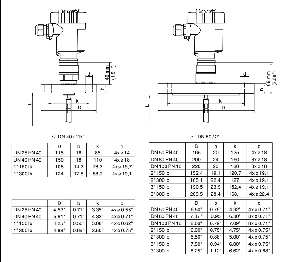
Рис. 27: VEGAFLEX 65, фланцевое исполнение L Длина датчика, см. "Технические данные"
