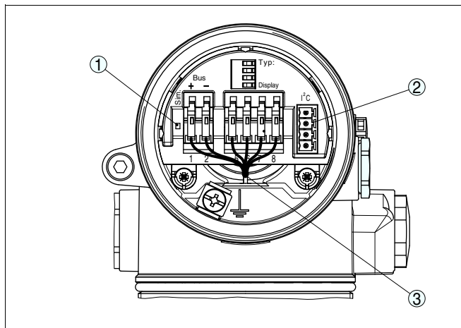
Рис. 8: Отсек электроники (двухкамерный корпус)
