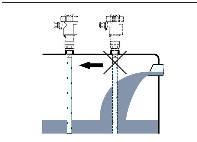
Рис. 4: Боковая нагрузка
