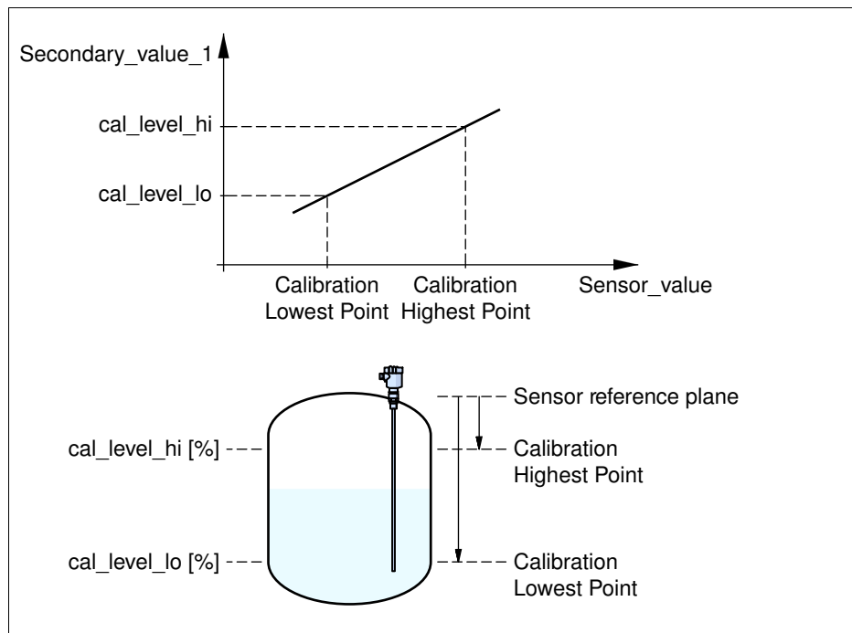
Рис. 21: Установка VEGAFLEX 65
