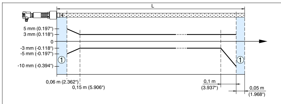
Рис. 31: Погрешность измерения VEGAFLEX 66 в коаксиальном исполнении (продукт - вода)
