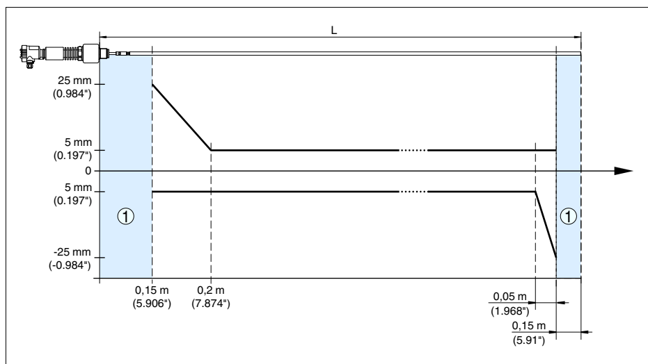
Рис. 26: Погрешность измерения VEGAFLEX 66 в стержневом исполнении (продукт - масло)
