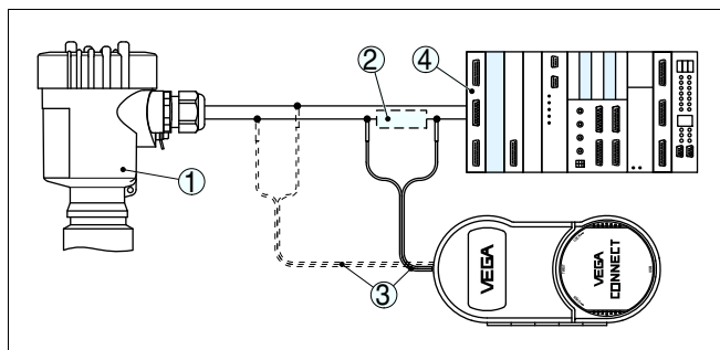
Рис. 22: Подключение ПК к сигнальному кабелю через HART
