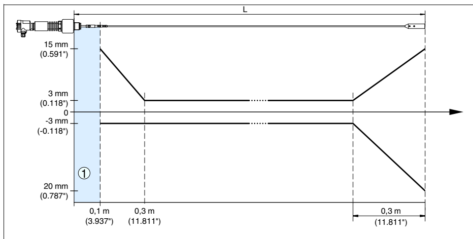
Рис. 27: Погрешность измерения VEGAFLEX 66 в тросовом исполнении, длина зонда L < 20 м (продукт - вода)
