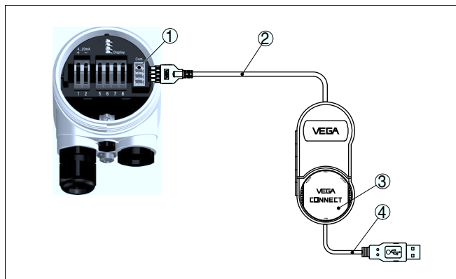
Рис. 21: Подключение через подключенный внешне VEGACONNECT
