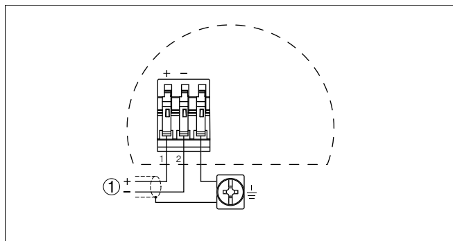
Рис. 16: Схема подключения для двухкамерного корпуса Ex d
