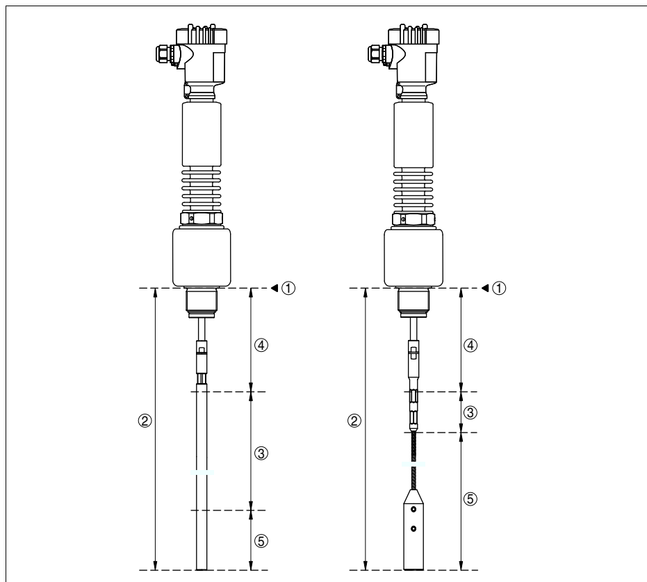
Рис. 24: Диапазон измерения VEGAFLEX 66 (исполнение с тросом или стержнем)
