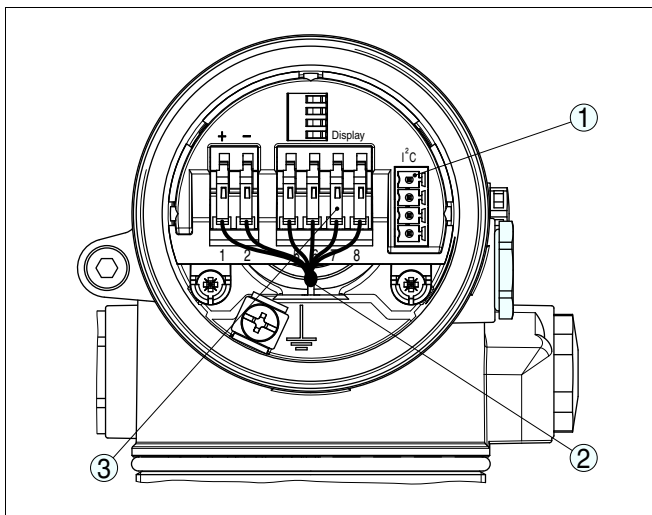
Рис. 14: Отсек электроники в двухкамерном корпусе
