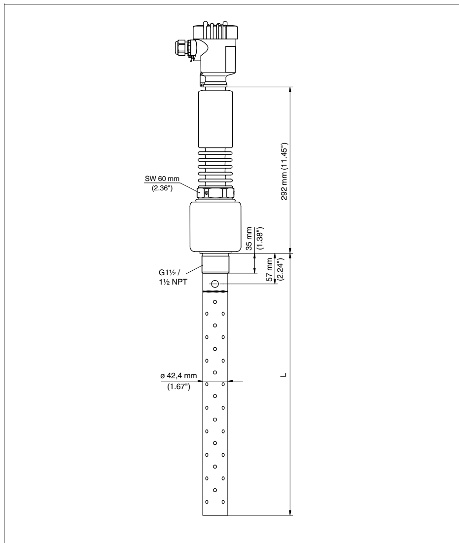
Рис. 41: VEGAFLEX 66 - коаксиальное исполнение с резьбовым присоединением (-200 ... +400 °C/-328 ... +752 °F)
