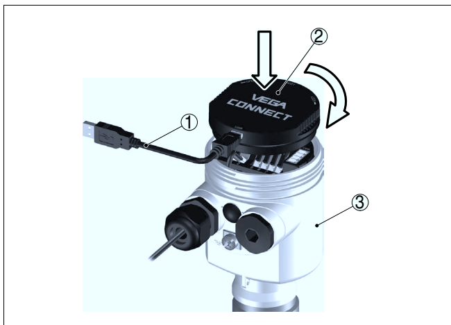
Рис. 20: Подключение ПК через VEGACONNECT прямо на датчике
