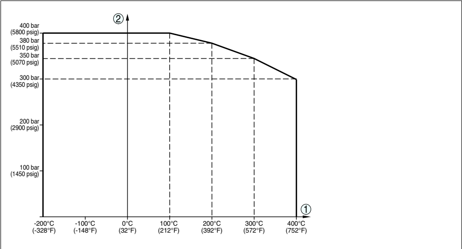
Рис. 33: Исполнение для высоких температур: давление процесса - температура процесса
