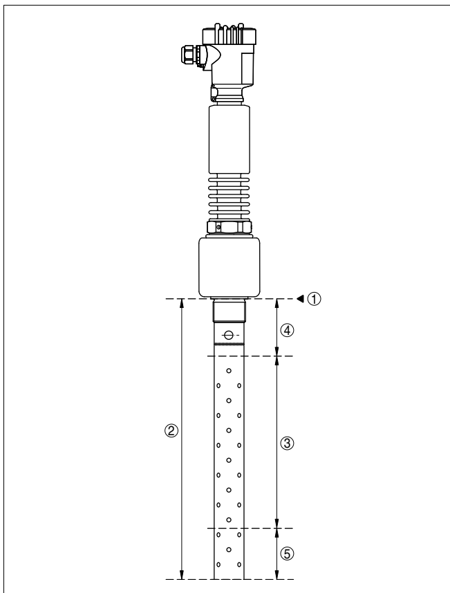
Рис. 23: Диапазон измерения VEGAFLEX 66 - коаксиальное исполнение
