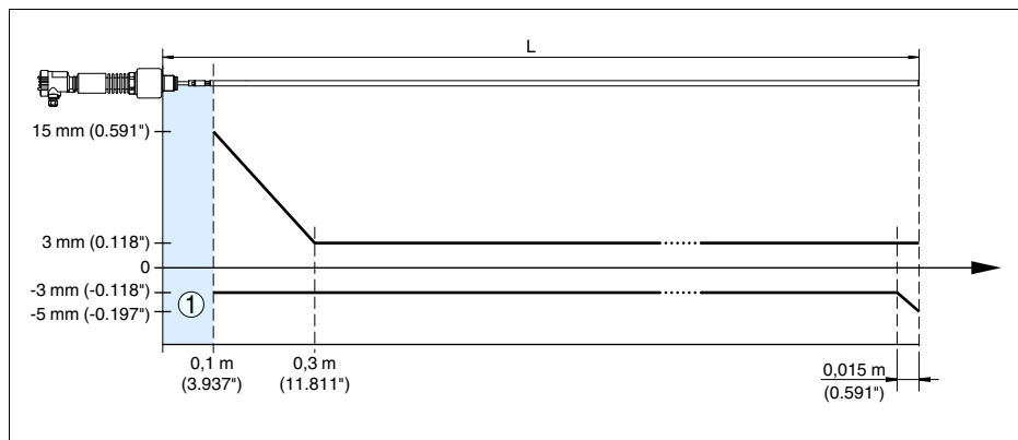
Рис. 25: Погрешность измерения VEGAFLEX 66 в стержневом исполнении (продукт - вода)
