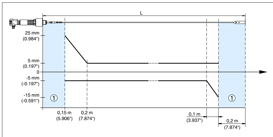
Рис. 28: Погрешность измерения VEGAFLEX 66 в тросовом исполнении, длина зонда L < 20 м (продукт - масло)
