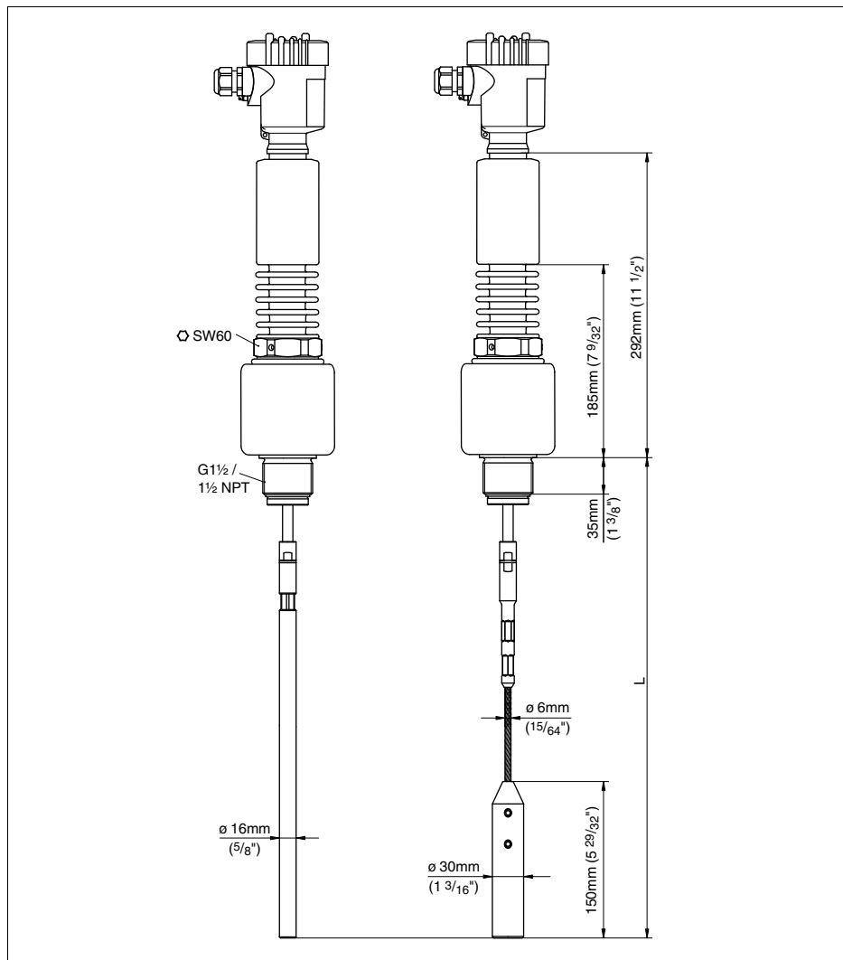
Рис. 40: VEGAFLEX 66 - исполнение с тросом или стержнем, с резьбовым присоединением (-200 ... +400 °C/-328 ... +752 °F)
