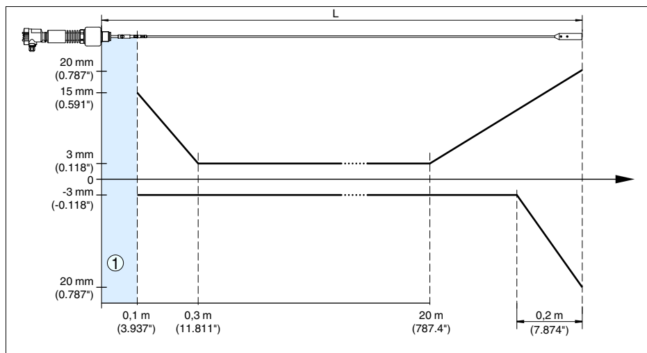
Рис. 29: Погрешность измерения VEGAFLEX 66 в тросовом исполнении, длина зонда L > 20 м (продукт - вода)
