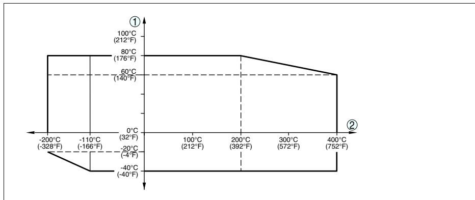
Рис. 34: Температура окружающей среды - температура процесса (исполнение -200 ... +400 °C/-328 ... +752 °F)
