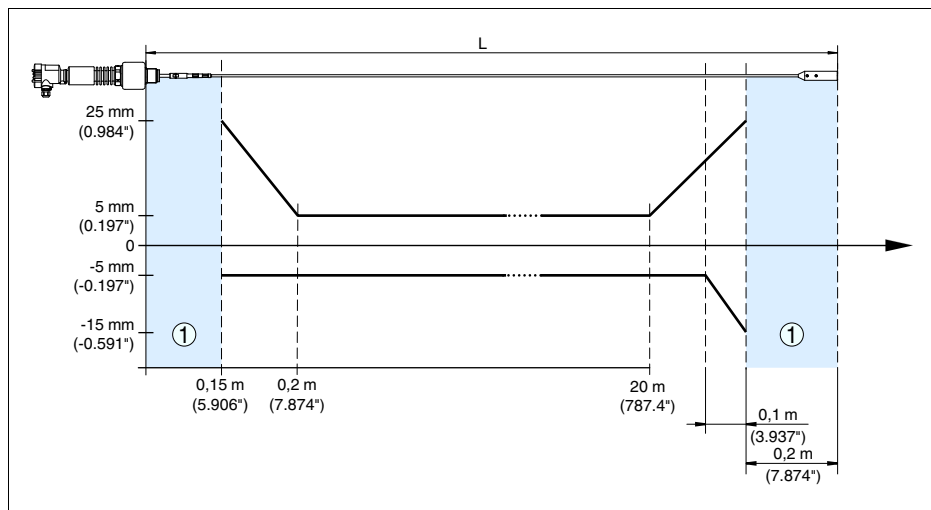
Рис. 30: Погрешность измерения VEGAFLEX 66 в тросовом исполнении, длина зонда L > 20 м (продукт - масло)
