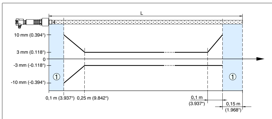
Рис. 32: Погрешность измерения VEGAFLEX 66 в коаксиальном исполнении (продукт - масло)
