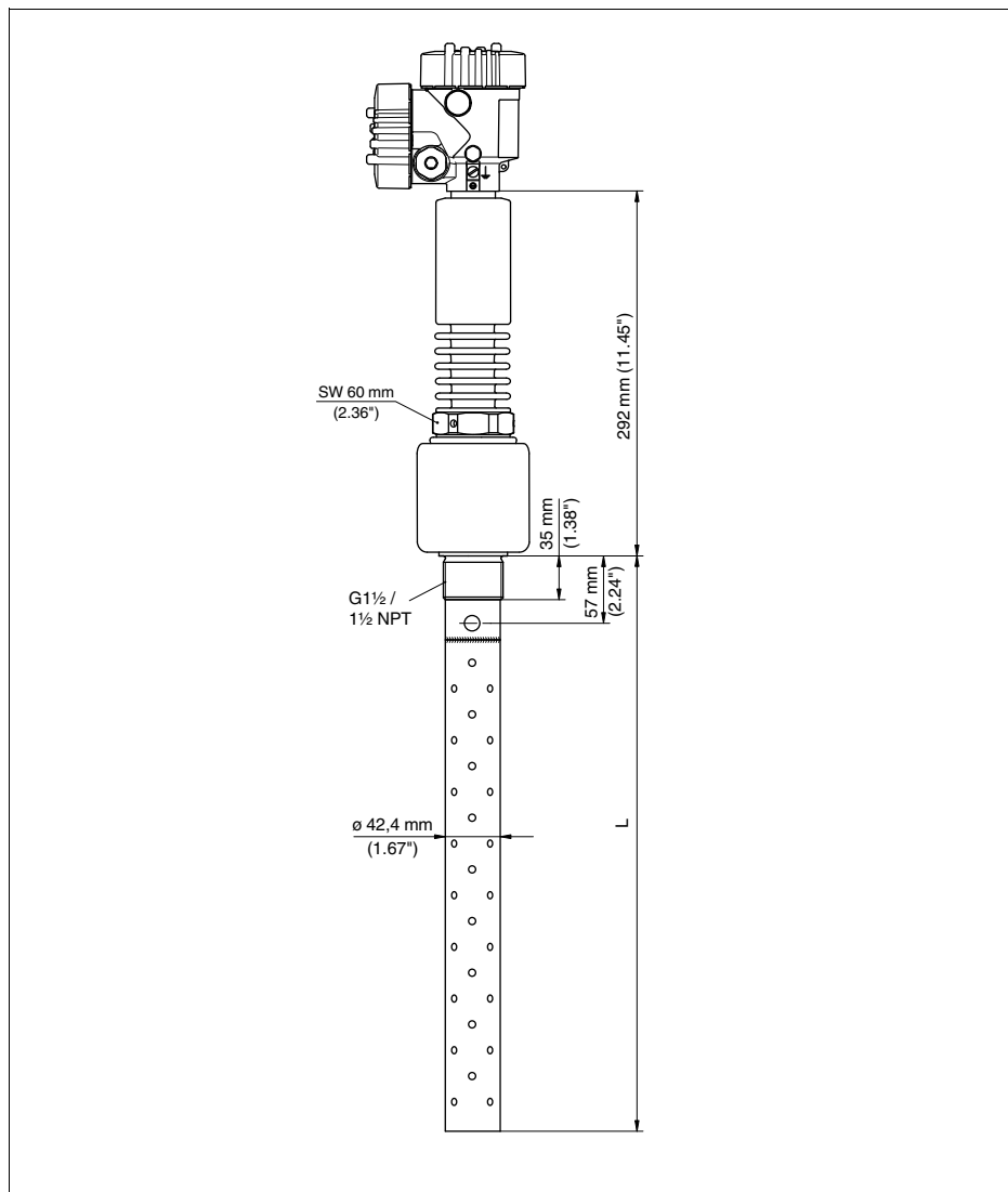
Рис. 31: VEGAFLEX 66 - коаксиальное исполнение с резьбовым присоединением (-200 ... +400 °C/-328 ... +752 °F)
