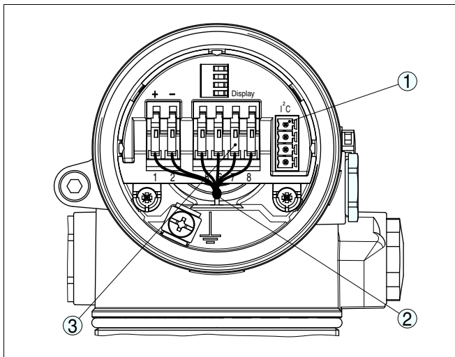
Рис. 9: Отсек электроники в двухкамерном корпусе
