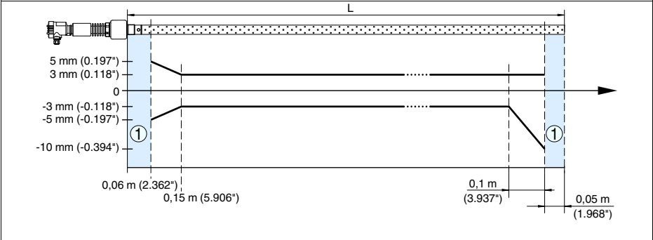
Рис. 25: Погрешность измерения VEGAFLEX 66 в коаксиальном исполнении (продукт - вода)
