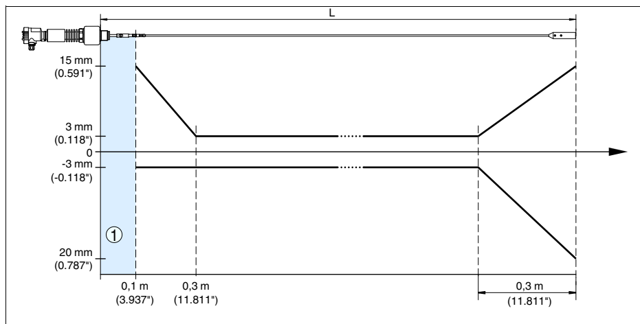
Рис. 21: Погрешность измерения VEGAFLEX 66 в тросовом исполнении, длина зонда L < 20 м (продукт - вода)
