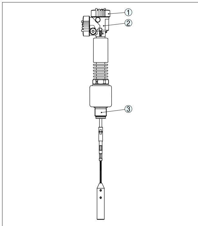
Рис. 1: VEGAFLEX 66 в исполнении с тросом и двухкамерным корпусом
