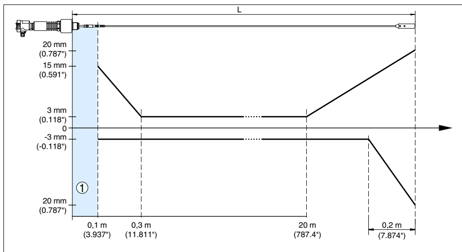
Рис. 23: Погрешность измерения VEGAFLEX 66 в тросовом исполнении, длина зонда L > 20 м (продукт - вода)
