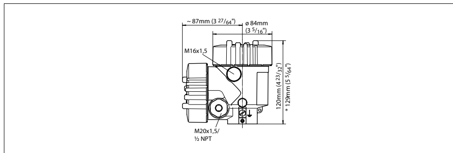
Рис. 29: Двухкамерный корпус (с установленным модулем индикации и настройки крышка корпуса выше на 9 мм)
