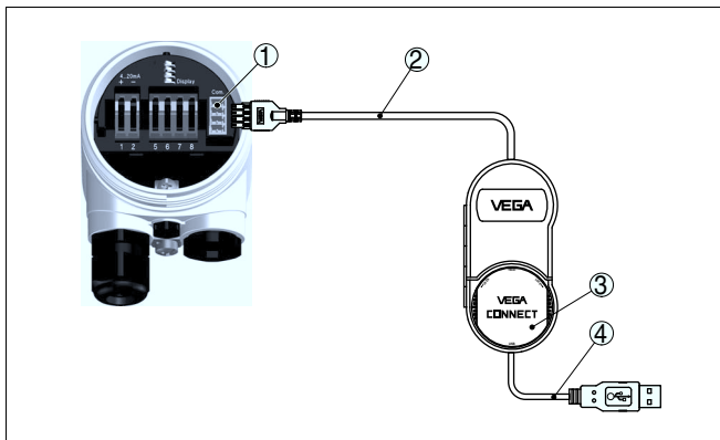
Рис. 15: Подключение через подключенный внешне VEGACONNECT
