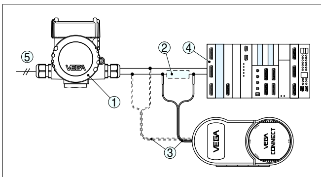
Рис. 16: Подключение ПК к сигнальному кабелю через HART
