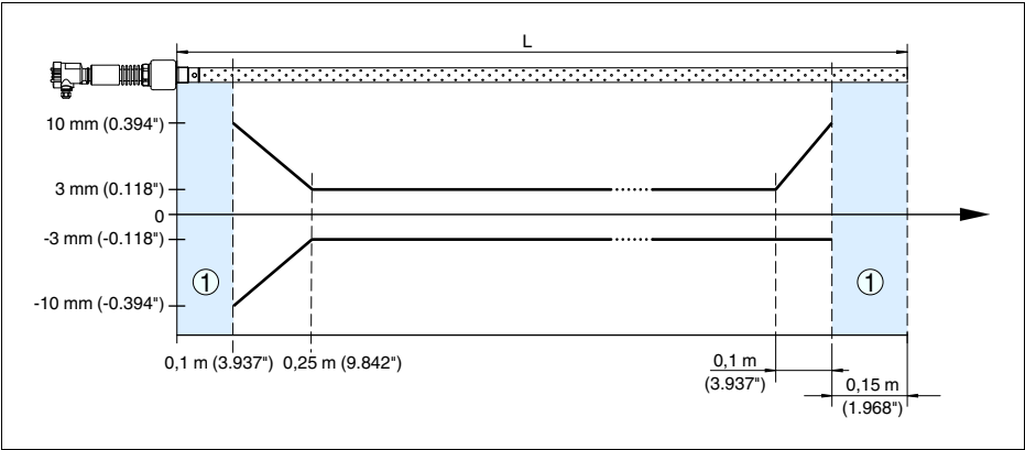
Рис. 26: Погрешность измерения VEGAFLEX 66 в коаксиальном исполнении (продукт - масло)
