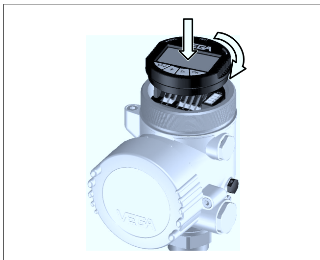
Рис. 12: Установка модуля индикации и настройки
