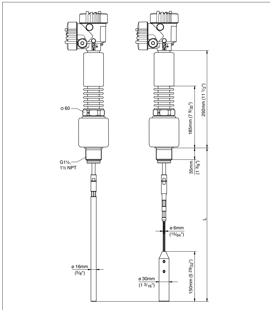
Рис. 30: VEGAFLEX 66 - исполнение с тросом или стержнем, с резьбовым присоединением (-200 ... +400 °C/-328 ... +752 °F)
