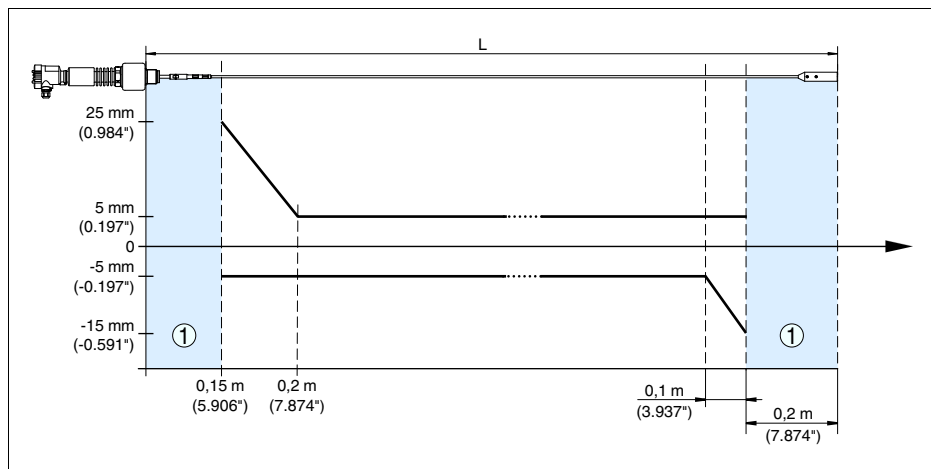
Рис. 22: Погрешность измерения VEGAFLEX 66 в тросовом исполнении, длина зонда L < 20 м (продукт - масло)
