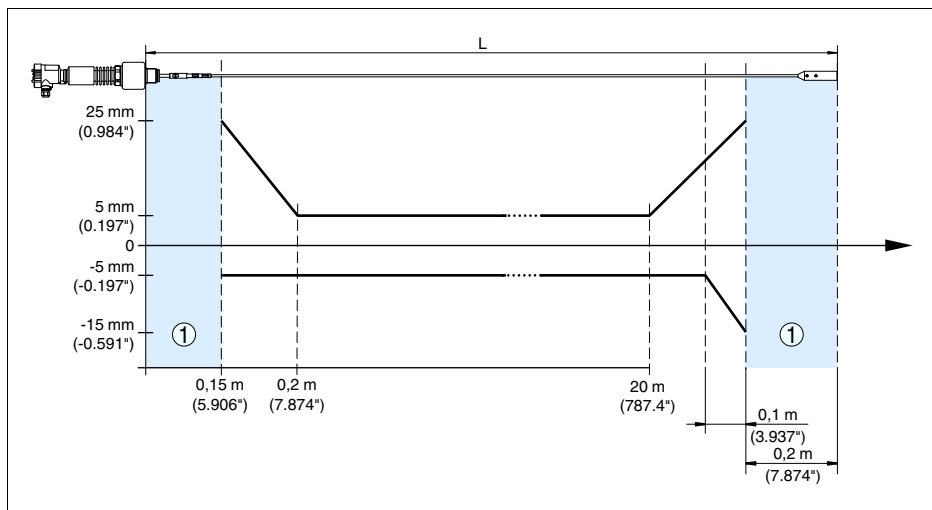
Рис. 24: Погрешность измерения VEGAFLEX 66 в тросовом исполнении, длина зонда L > 20 м (продукт - масло)
