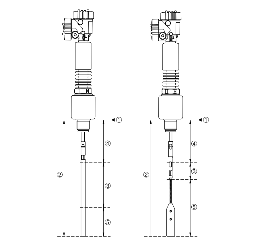
Рис. 18: Диапазон измерения VEGAFLEX 66 (исполнение с тросом или стержнем)
