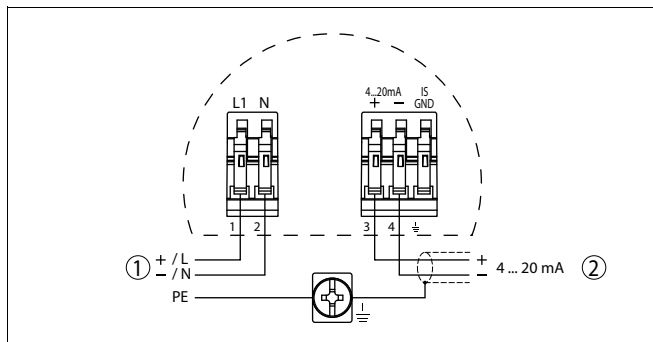
Рис. 11: Схема подключения (двухкамерный корпус)
