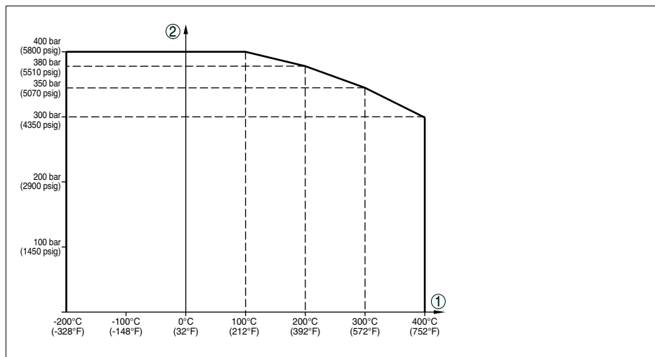
Рис. 27: Исполнение для высоких температур: давление процесса - температура процесса
