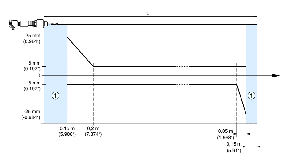
Рис. 20: Погрешность измерения VEGAFLEX 66 в стержневом исполнении (продукт - масло)
