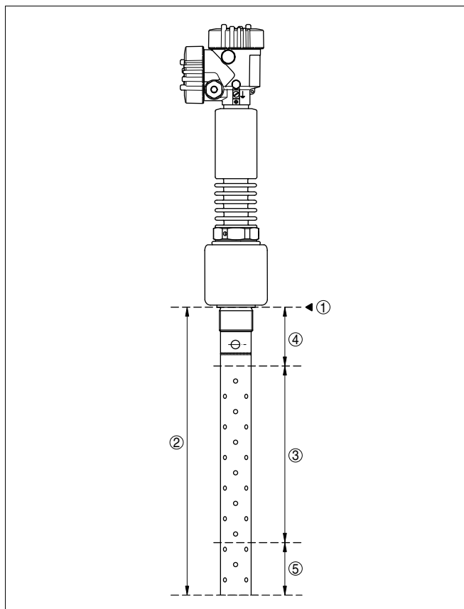
Рис. 17: Диапазон измерения VEGAFLEX 66 - коаксиальное исполнение
