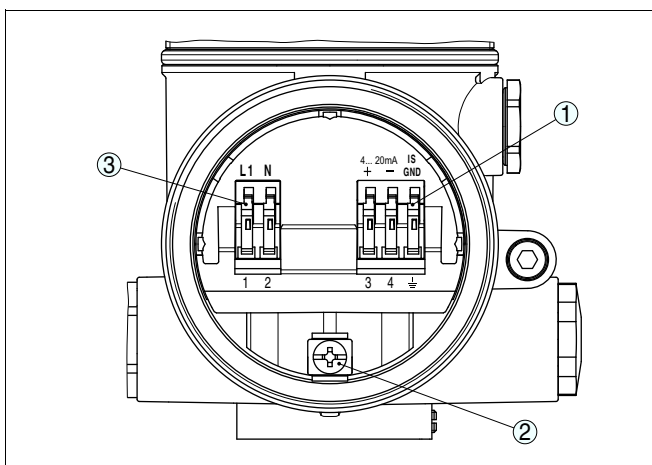
Рис. 10: Отсек подключения в двухкамерном корпусе
