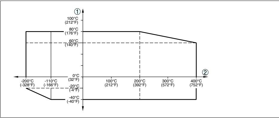
Рис. 28: Температура окружающей среды - температура процесса (исполнение -200 ... +400 °C/-328 ... +752 °F)
