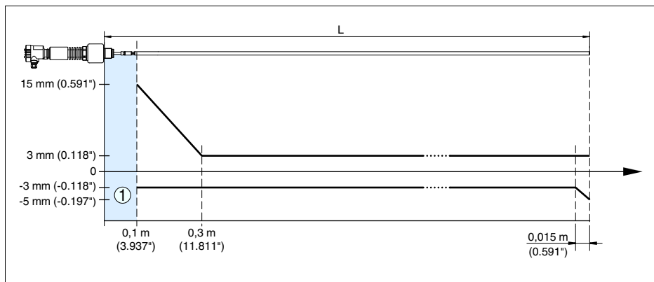
Рис. 19: Погрешность измерения VEGAFLEX 66 в стержневом исполнении (продукт - вода)
