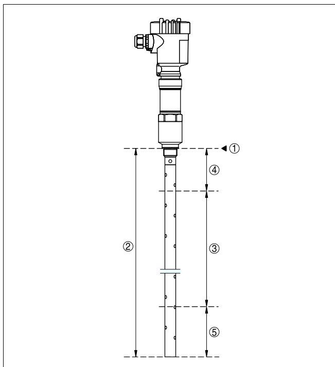
Рис. 18: Диапазон измерения VEGAFLEX 66 - коаксиальное исполнение
