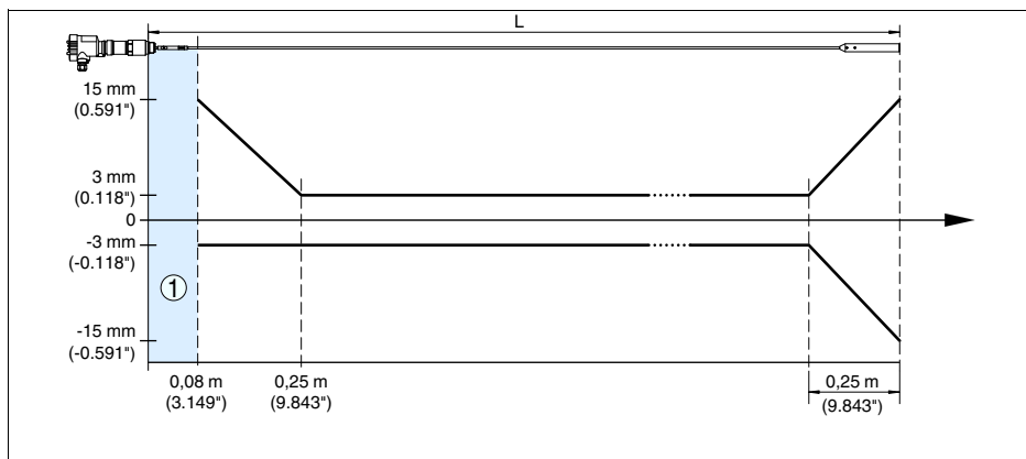
Рис. 22: Погрешность измерения VEGAFLEX 66 в тросовом исполнении, длина зонда L < 20 м (продукт - вода)
