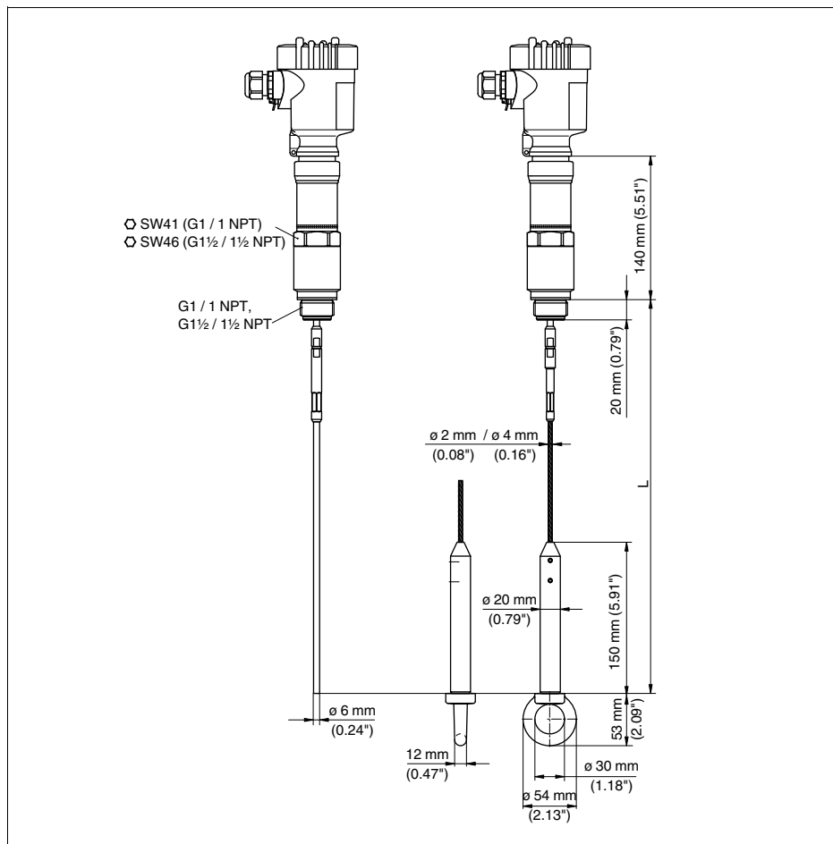
Рис. 33: VEGAFLEX 66 - исполнение с тросом или стержнем, с резьбовым присоединением (-20 ... +250 °C/-4 ... +482 °F)
