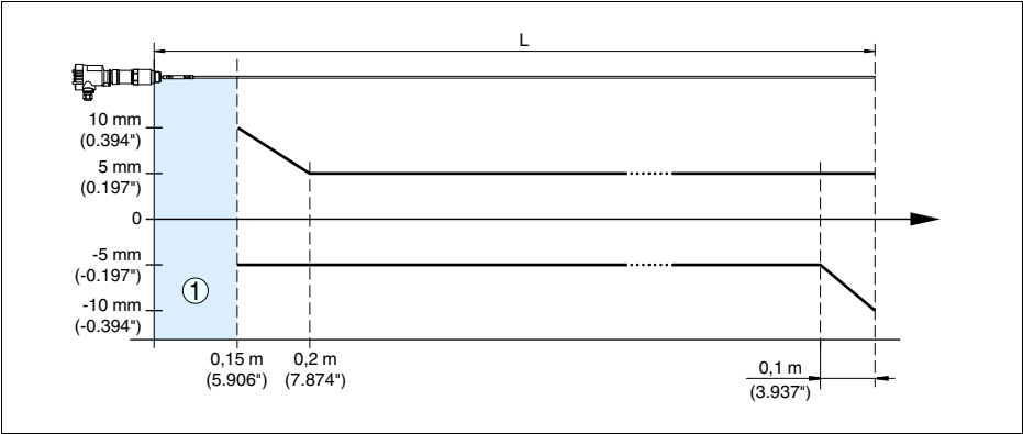
Рис. 21: Погрешность измерения VEGAFLEX 66 в стержневом исполнении (продукт - масло)
