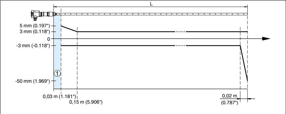
Рис. 24: Погрешность измерения VEGAFLEX 66 в коаксиальном исполнении (продукт - вода)
