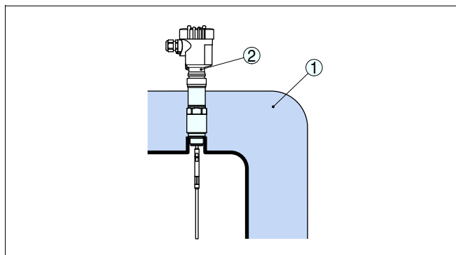
Рис. 6: Емкость с температурной изоляцией
