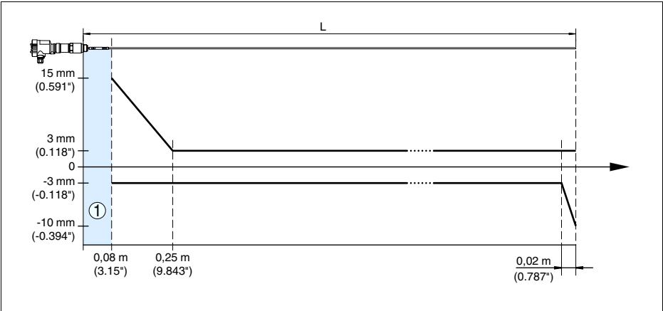
Рис. 20: Погрешность измерения VEGAFLEX 66 в стержневом исполнении (продукт - вода)
