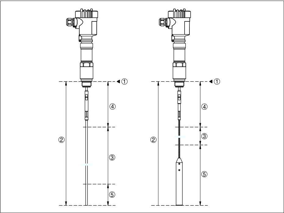
Рис. 19: Диапазон измерения VEGAFLEX 66 (исполнение с тросом или стержнем)
