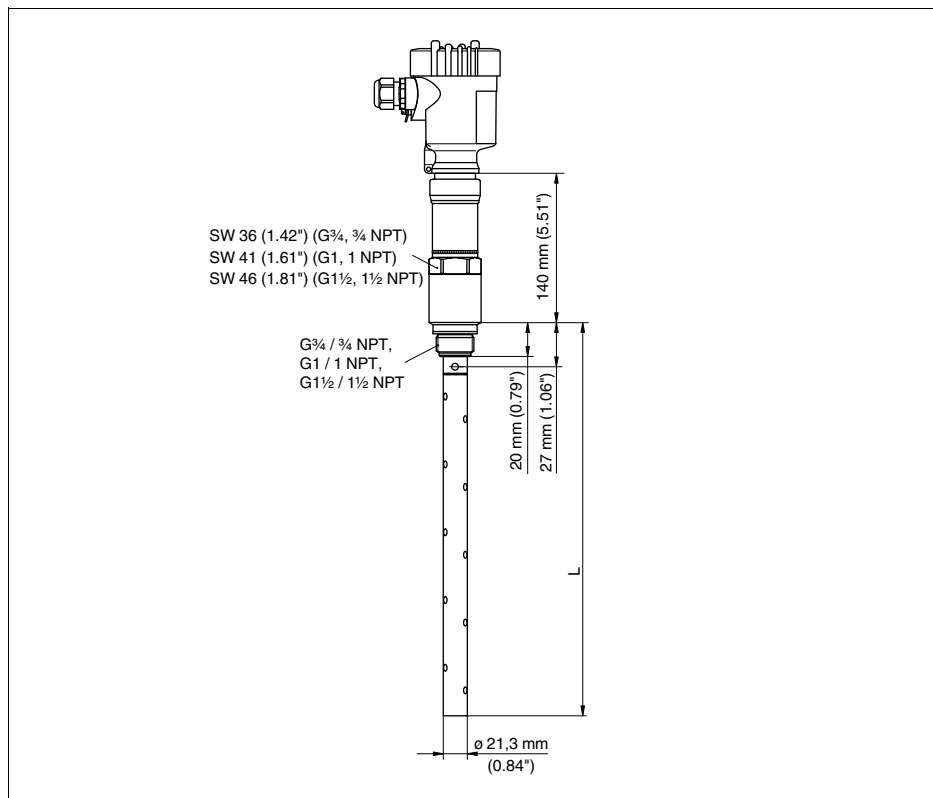
Рис. 34: VEGAFLEX 66, коаксиальное исполнение с резьбовым присоединением (-20 ... +250 °C/-4 ... +482 °F)
