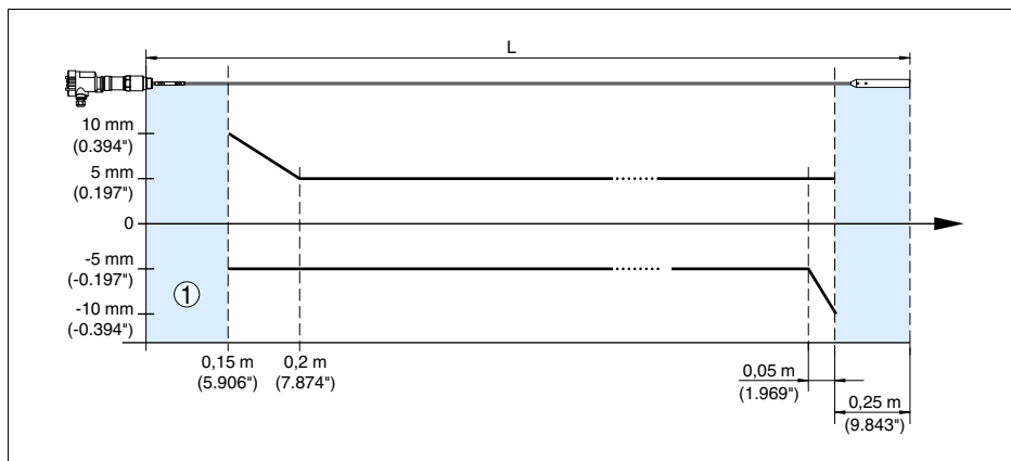
Рис. 23: Погрешность измерения VEGAFLEX 66 в тросовом исполнении, длина зонда L < 20 м (продукт - масло)
