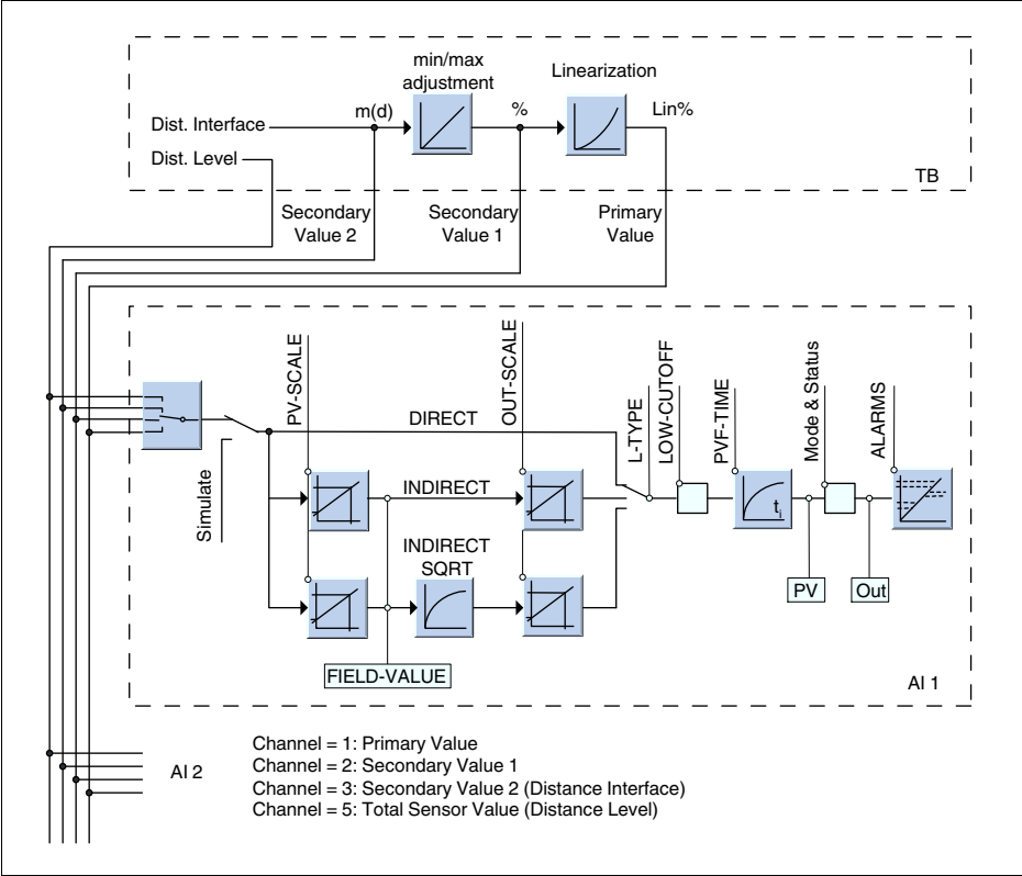
Рис. 27: Обработка измеренных значений VEGAFLEX 66
