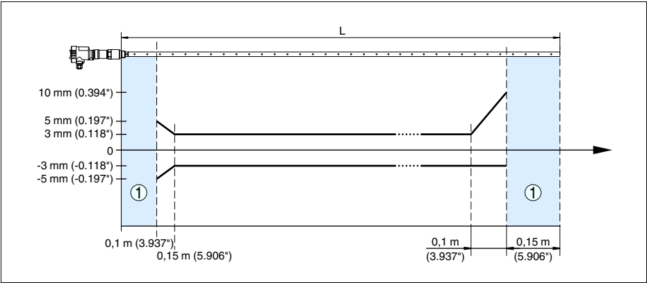
Рис. 25: Погрешность измерения VEGAFLEX 66 в коаксиальном исполнении (продукт - масло)
