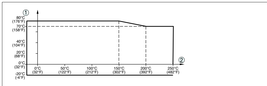
Рис. 26: Температура окружающей среды - температура процесса (исполнение -20 ... +250 °C/-4 ... +482 °F)
