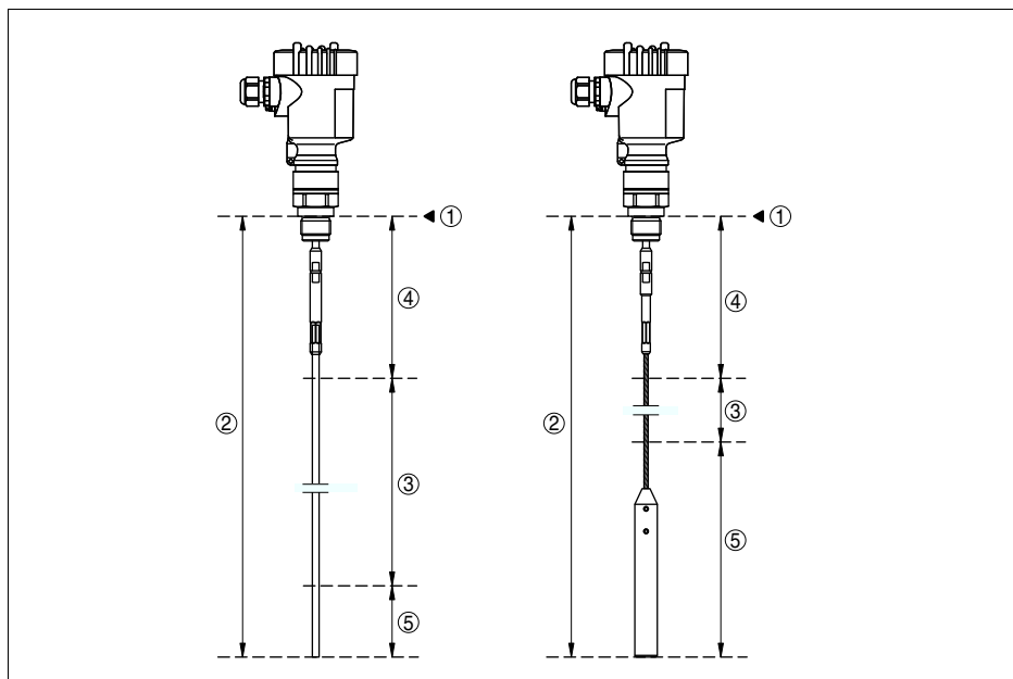
Рис. 22: Диапазон измерения VEGAFLEX 67 (исполнение с тросом или стержнем)
