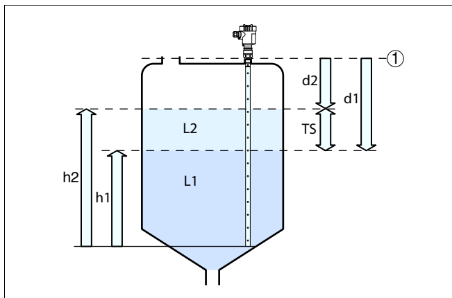
Рис. 24: Измерение межфазного уровня (раздел фаз находится между L1 и L2)
