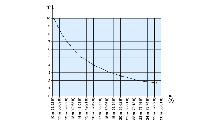
Рис. 23: Отношение диэлектрической постоянной ( \epsilon_r ) верхнего продукта к максимальной длине измерительного зонда
