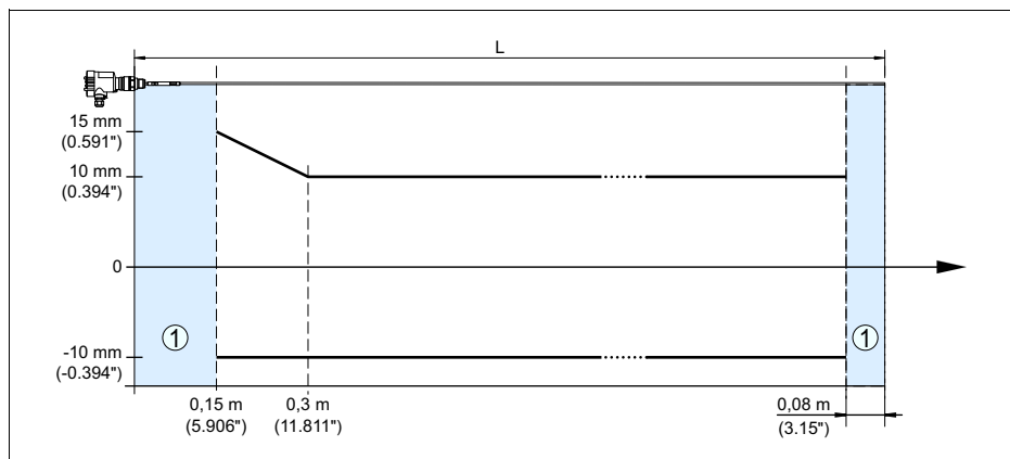
Рис. 25: Погрешность измерения VEGAFLEX 67 в стержневом исполнении
