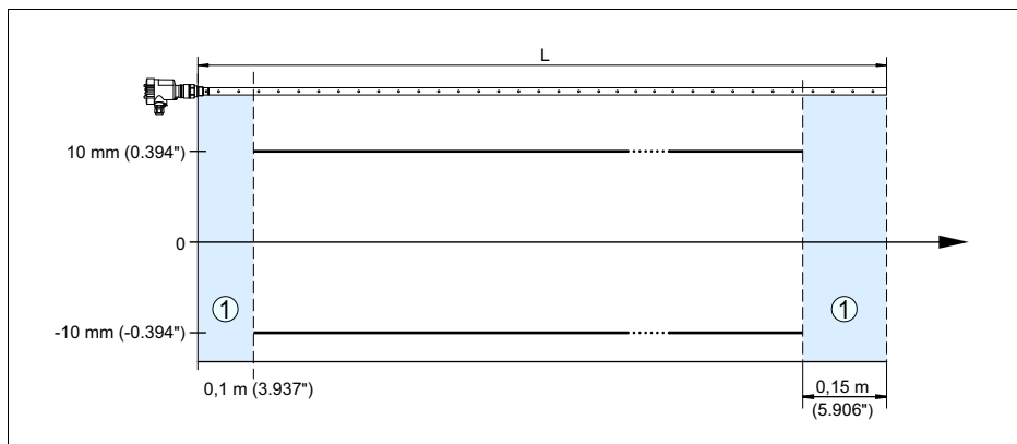
Рис. 27: Погрешность измерения VEGAFLEX 67 в коаксиальном исполнении
