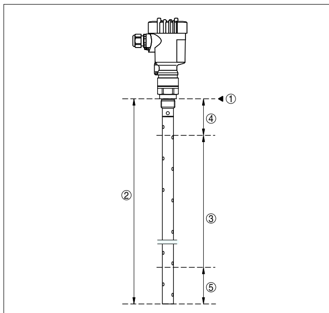
Рис. 21: Диапазон измерения VEGAFLEX 67 - коаксиальное исполнение
