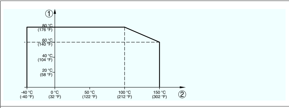
Рис. 28: Температура окружающей среды - Температура процесса
