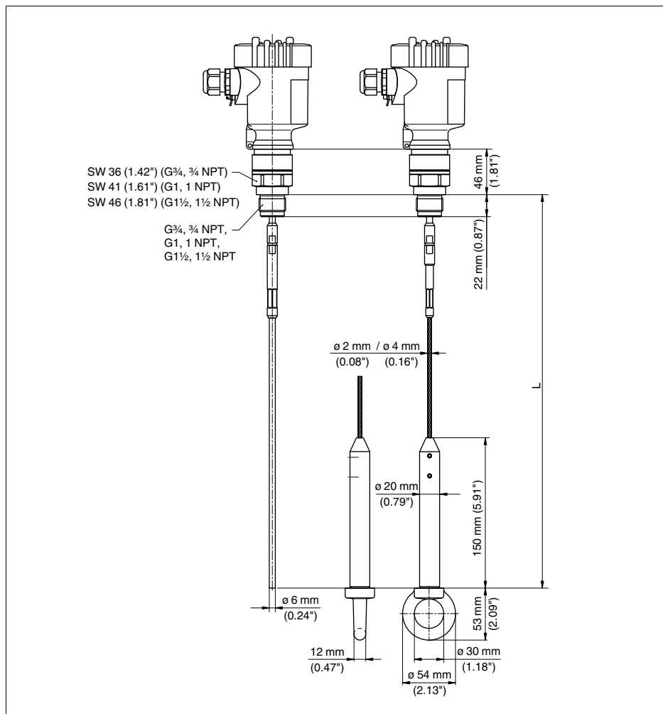
Рис. 34: VEGAFLEX 67, тросовое или стержневое исполнение, с резьбовым присоединением
