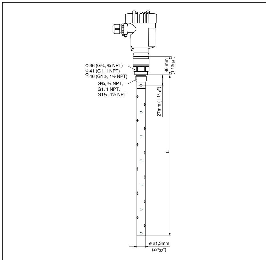
Рис. 35: VEGAFLEX 67, коаксиальное исполнение с резьбовым присоединением
