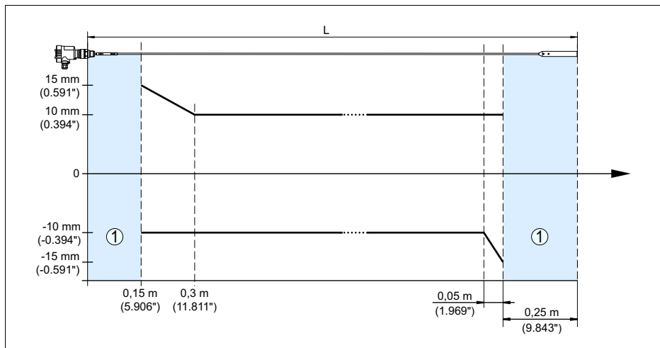
Рис. 26: Погрешность измерения VEGAFLEX 67 в тросовом исполнении
