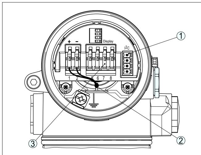
Рис. 7: Отсек электроники (двухкамерный корпус)
