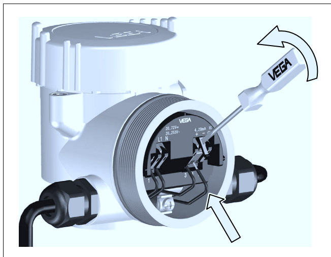
Рис. 6: Подключение: шаги 5 и 6
