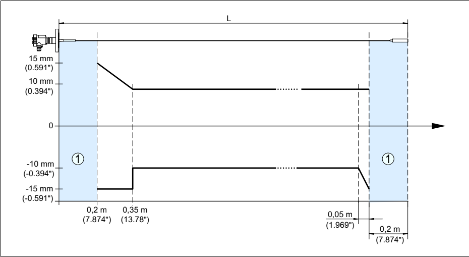
Рис. 19: Погрешность измерения VEGAFLEX 67 в тросовом исполнении
