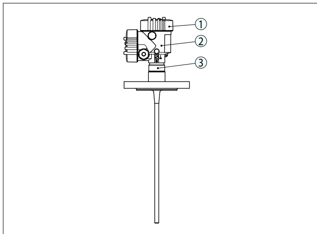
Рис. 1: VEGAFLEX 67 в исполнении со стержнем и двухкамерным корпусом
