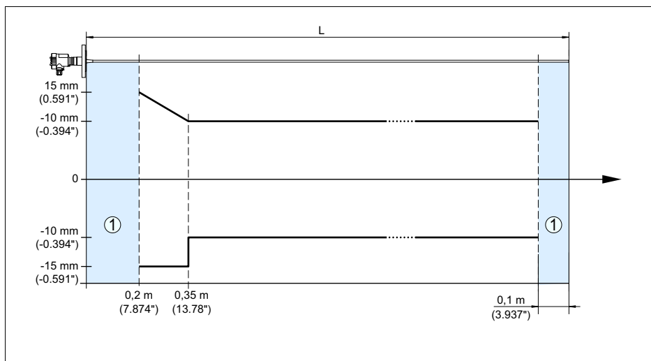
Рис. 18: Погрешность измерения VEGAFLEX 67 в стержневом исполнении
