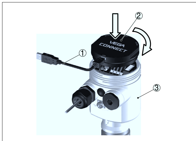
Рис. 12: Подключение ПК через VEGACONNECT прямо на датчике
