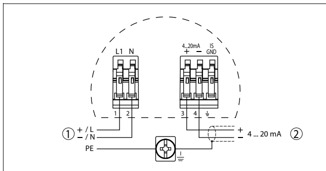
Рис. 9: Схема подключения (двухкамерный корпус)
