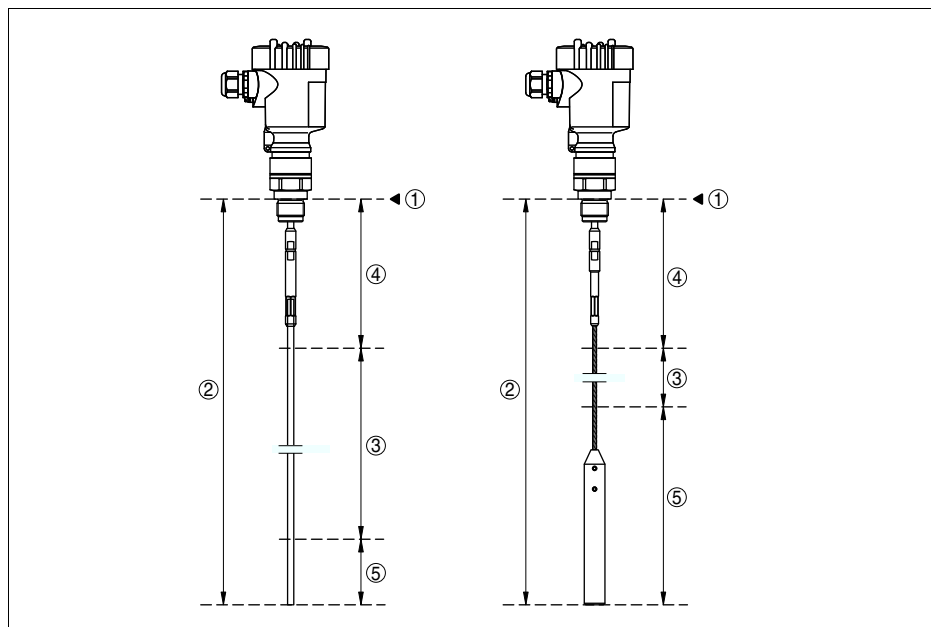
Рис. 15: Диапазон измерения VEGAFLEX 67 (исполнение с тросом или стержнем)
