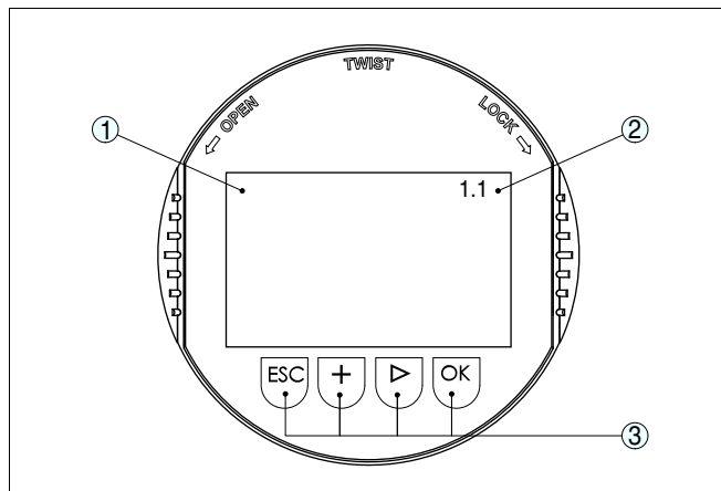
Рис. 11: Элементы индикации и настройки
