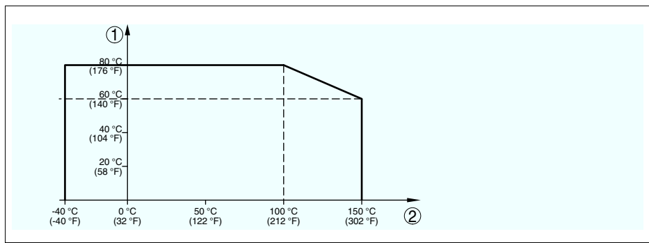
Рис. 20: Температура окружающей среды - Температура процесса
