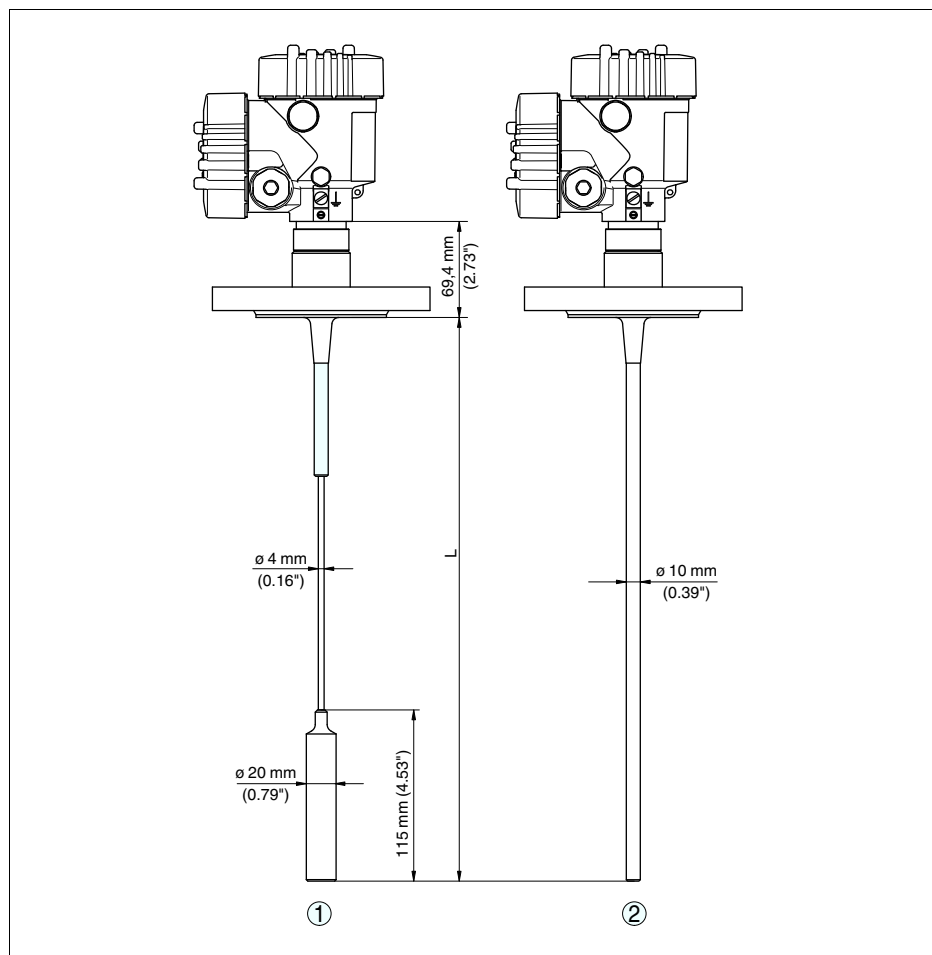
Рис. 22: VEGAFLEX 67, фланцевое исполнение
