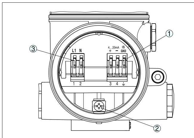
Рис. 8: Отсек подключения (двухкамерный корпус)
