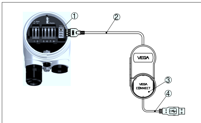
Рис. 13: Подключение через подключенный внешне VEGACONNECT
