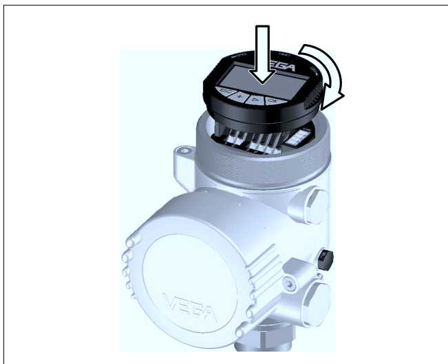
Рис. 10: Установка модуля индикации и настройки
