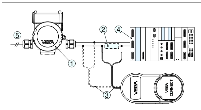
Рис. 14: Подключение ПК к сигнальному кабелю через HART
