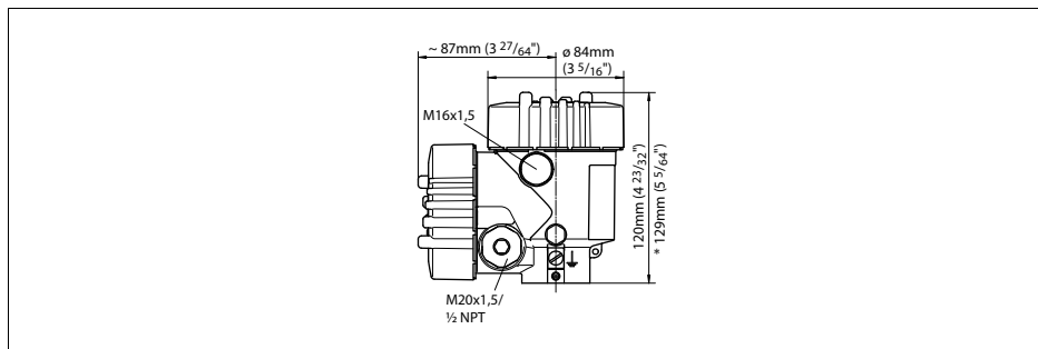
Рис. 21: Двухкамерный корпус (с установленным модулем индикации и настройки крышка корпуса выше на 9 мм)
