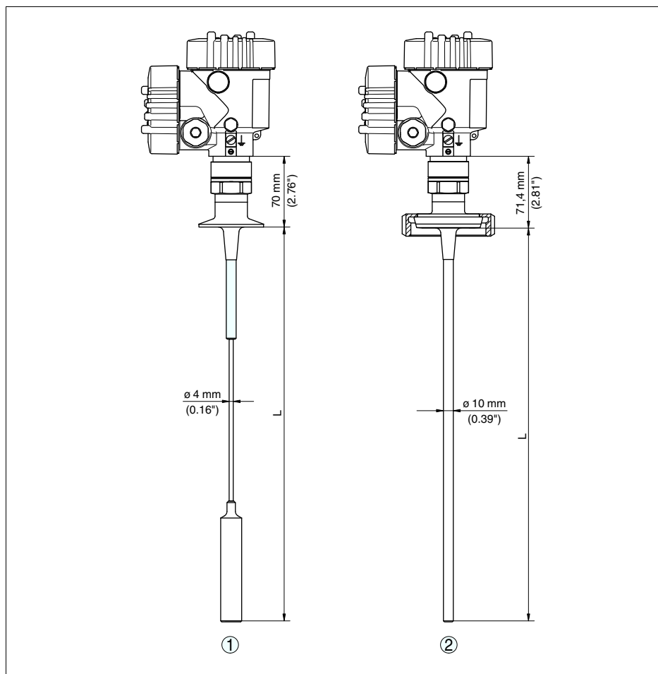
Рис. 23: VEGAFLEX 67, исполнения для пищевой промышленности
