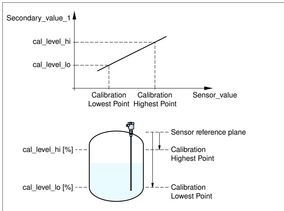
Рис. 27: Установка VEGAFLEX 67
