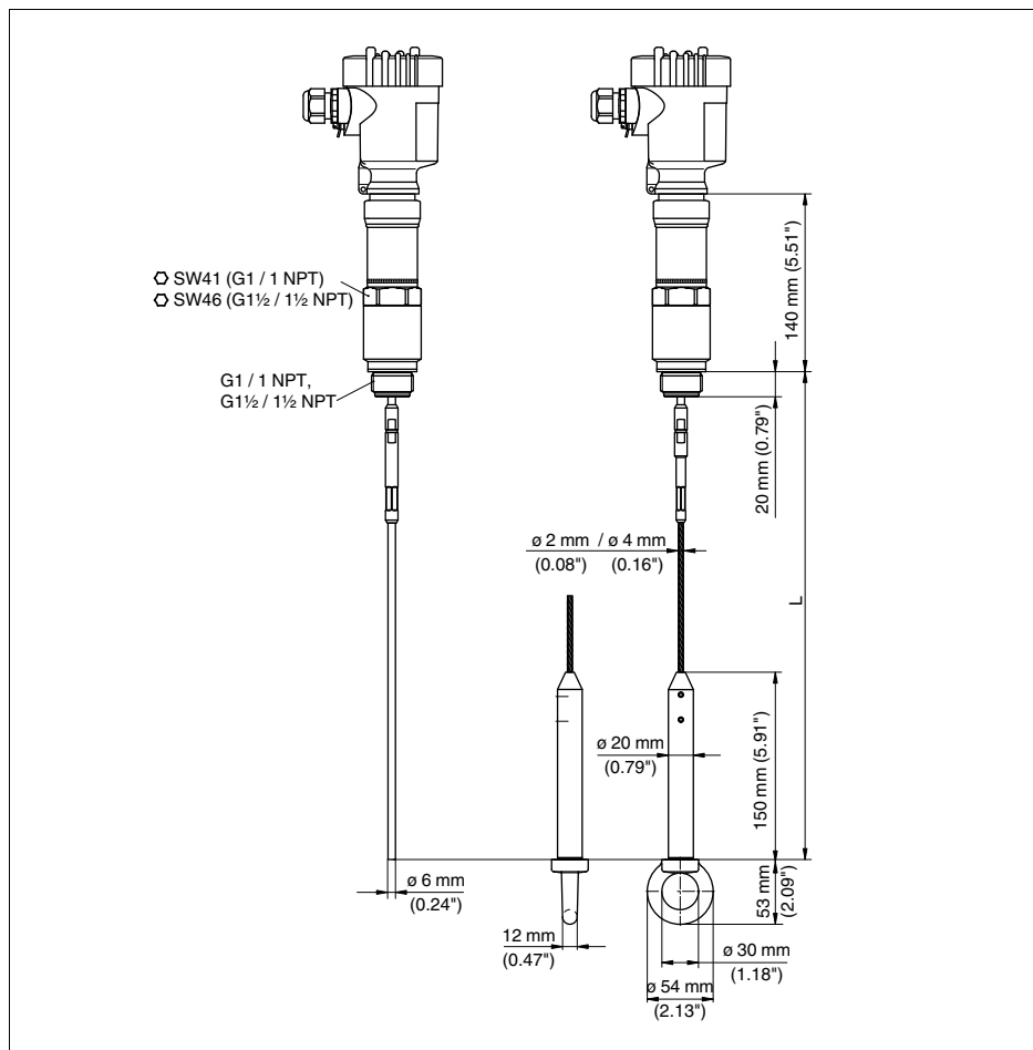
Рис. 32: VEGAFLEX 67, исполнение с тросом или стержнем, с резьбовым присоединением (-20 ... +250 °C/-4 ... +482 °F)
