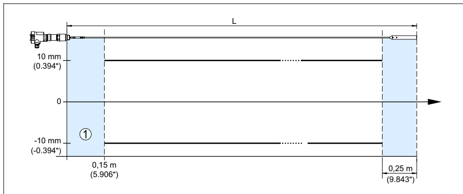
Рис. 23: Погрешность измерения VEGAFLEX 67 в тросовом исполнении
