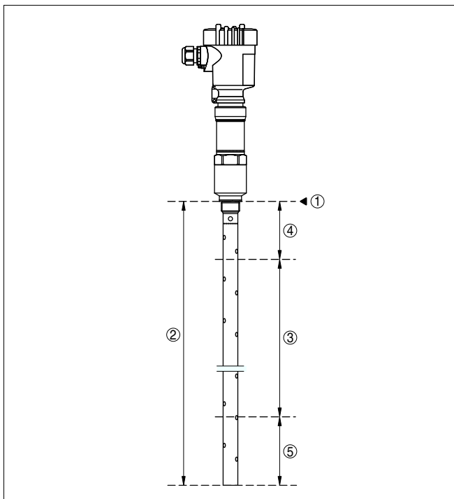
Рис. 18: Диапазон измерения VEGAFLEX 67 - коаксиальное исполнение
