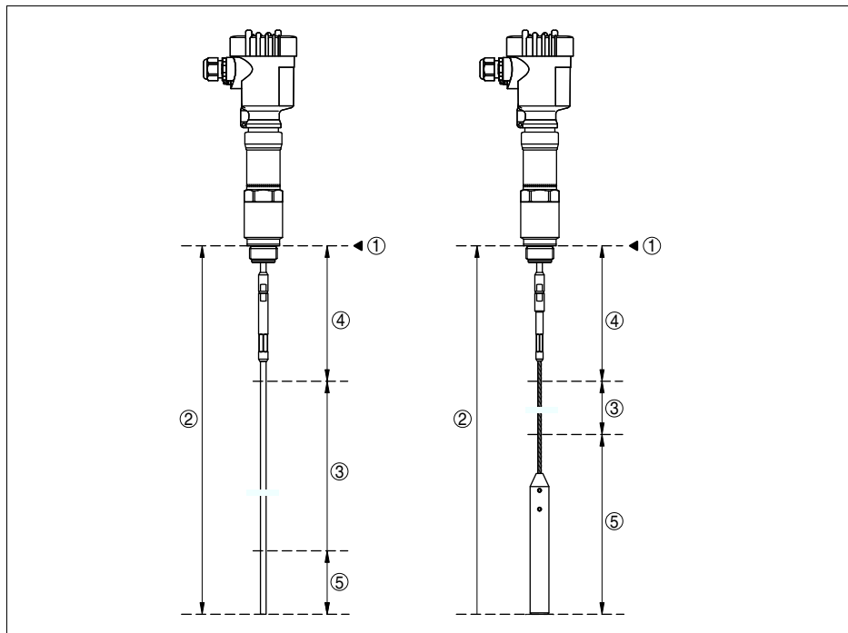
Рис. 19: Диапазон измерения VEGAFLEX 67 (исполнение с тросом или стержнем)
