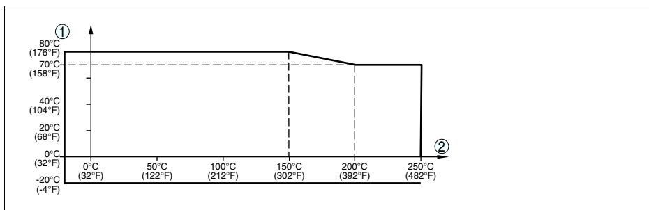
Рис. 25: Температура окружающей среды - температура процесса (исполнение -20 ... +250 °C/-4 ... +482 °F)
