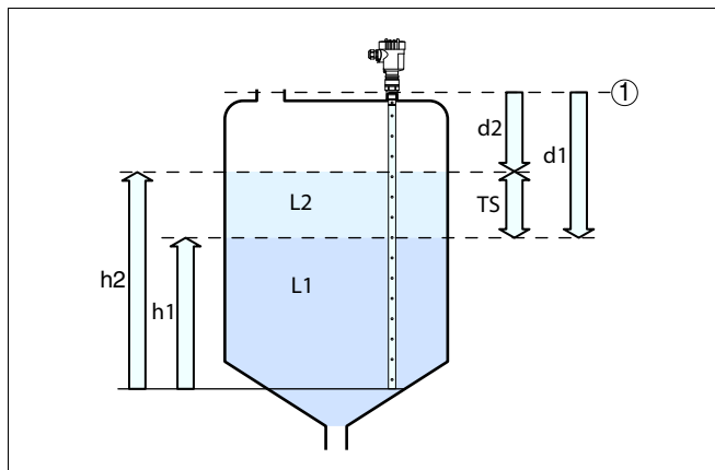
Рис. 2: Измерение межфазного уровня
