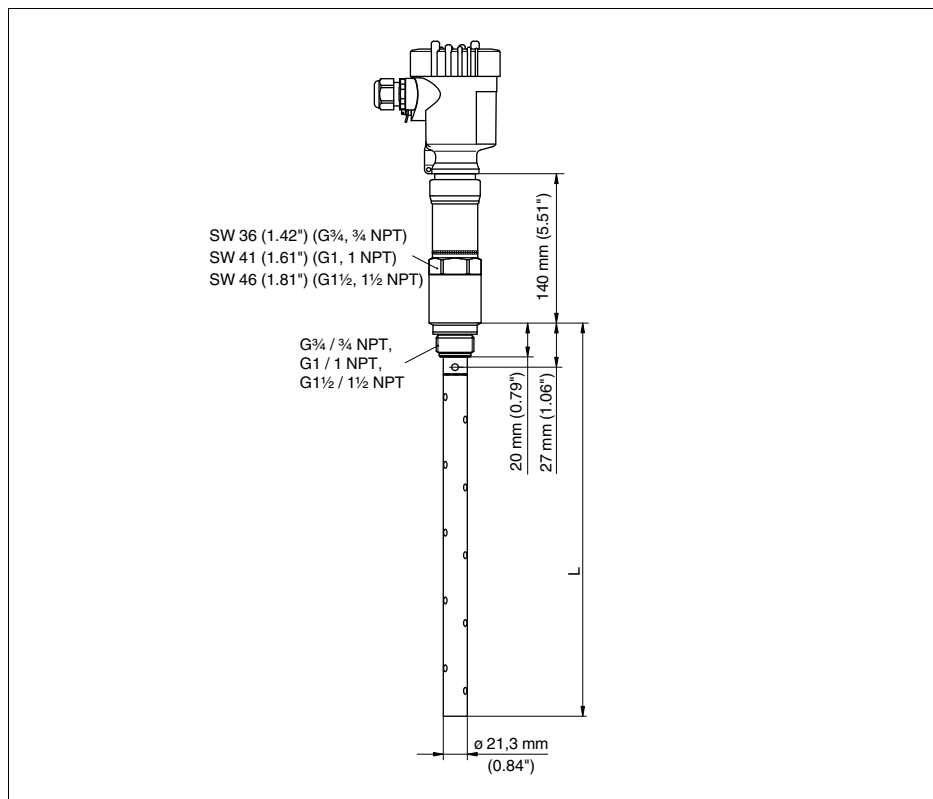
Рис. 33: VEGAFLEX 67, коаксиальное исполнение с резьбовым присоединением (-20 ... +250 °C/-4 ... +482 °F)
