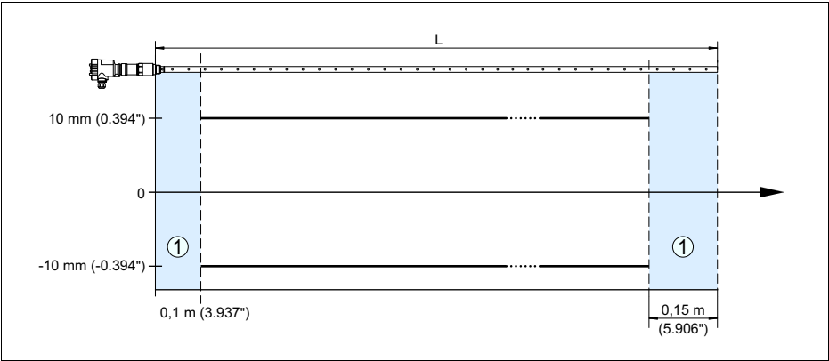
Рис. 24: Погрешность измерения VEGAFLEX 67 в коаксиальном исполнении
