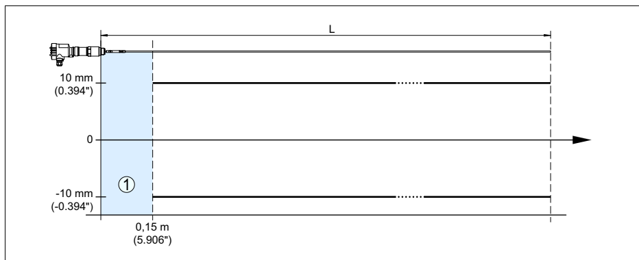
Рис. 22: Погрешность измерения VEGAFLEX 67 в стержневом исполнении
