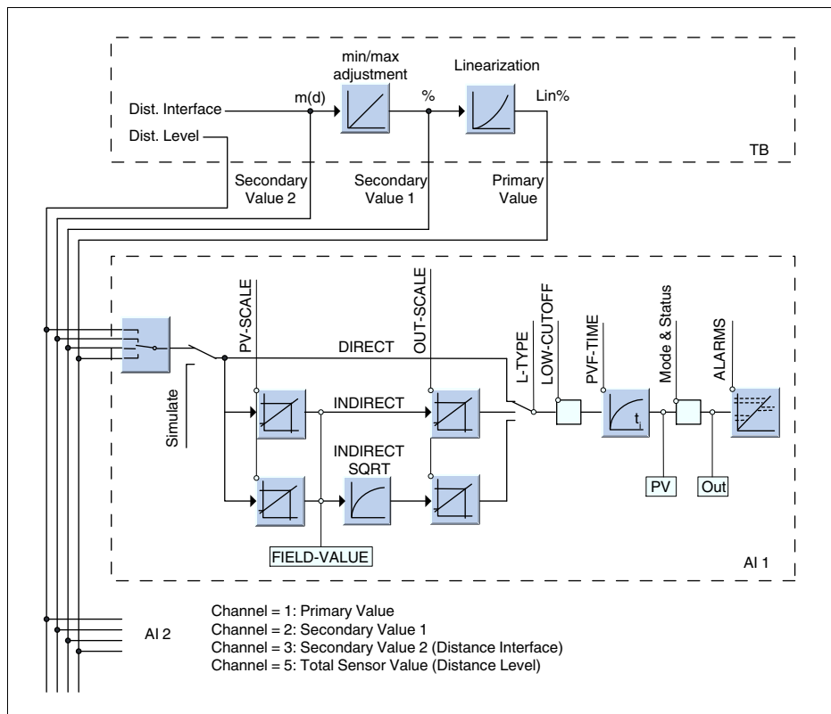
Рис. 26: Обработка измеренных значений VEGAFLEX 67
