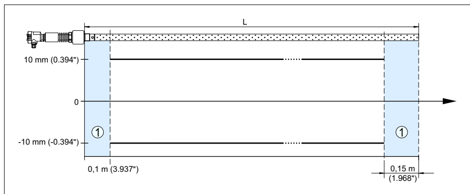
Рис. 24: Погрешность измерения VEGAFLEX 67 в коаксиальном исполнении
