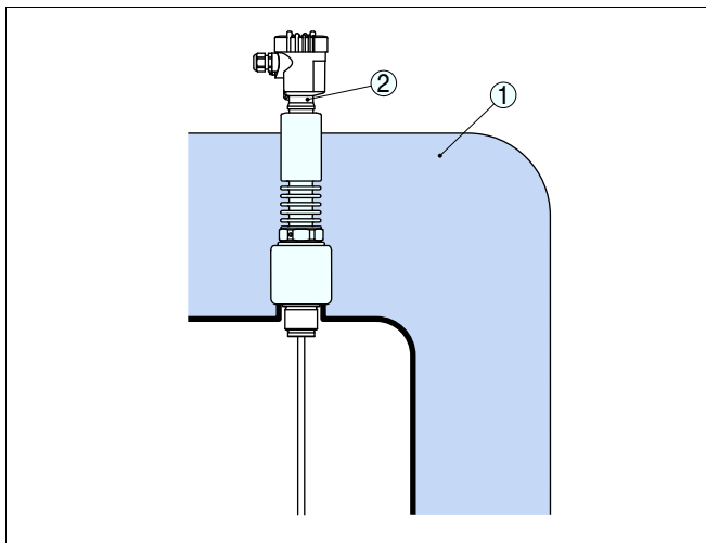
Рис. 6: Емкость с температурной изоляцией
