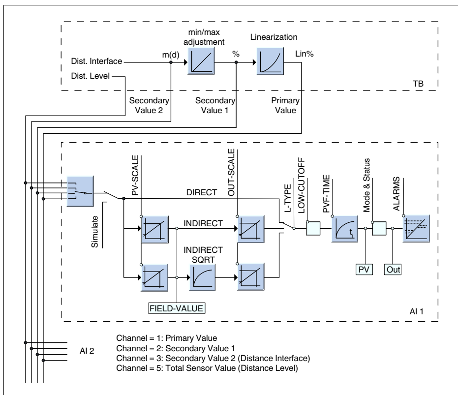
Рис. 27: Обработка измеренных значений VEGAFLEX 67
