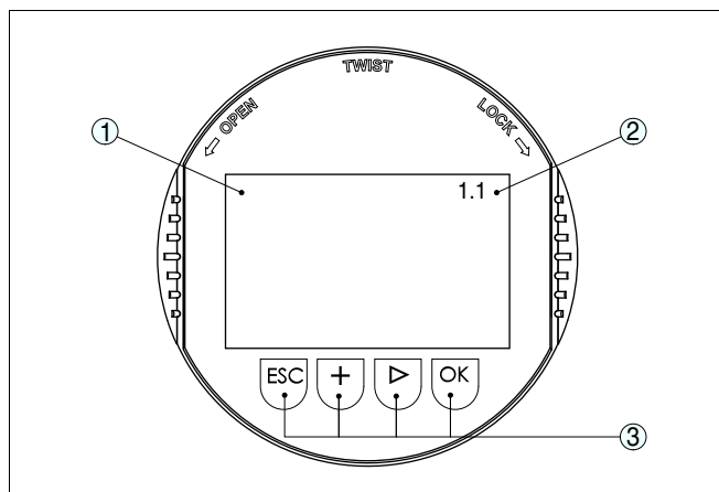
Рис. 15: Элементы индикации и настройки
