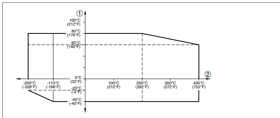
Рис. 26: Температура окружающей среды - температура процесса (исполнение -200 ... +400 °C/-328 ... +752 °F)
