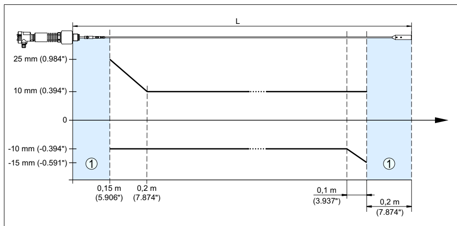
Рис. 23: Погрешность измерения VEGAFLEX 67 в тросовом исполнении
