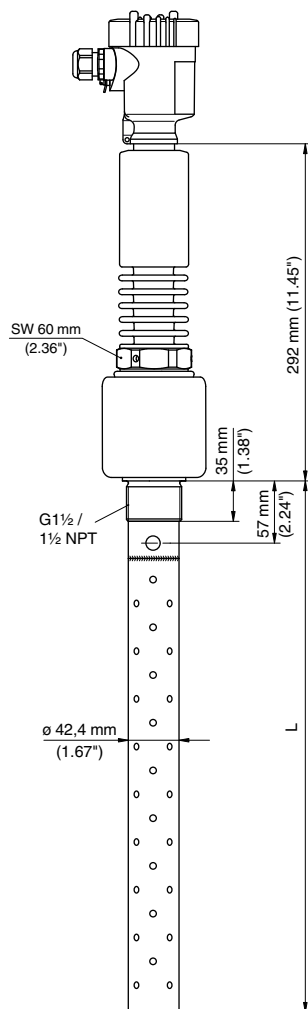
Рис. 34: VEGAFLEX 67, коаксиальное исполнение с резьбовым присоединением (-200 ... +400 °C/-328 ... +752 °F)
