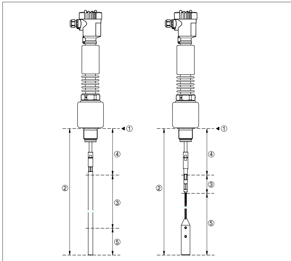
Рис. 19: Диапазон измерения VEGAFLEX 67 (исполнение с тросом или стержнем)
