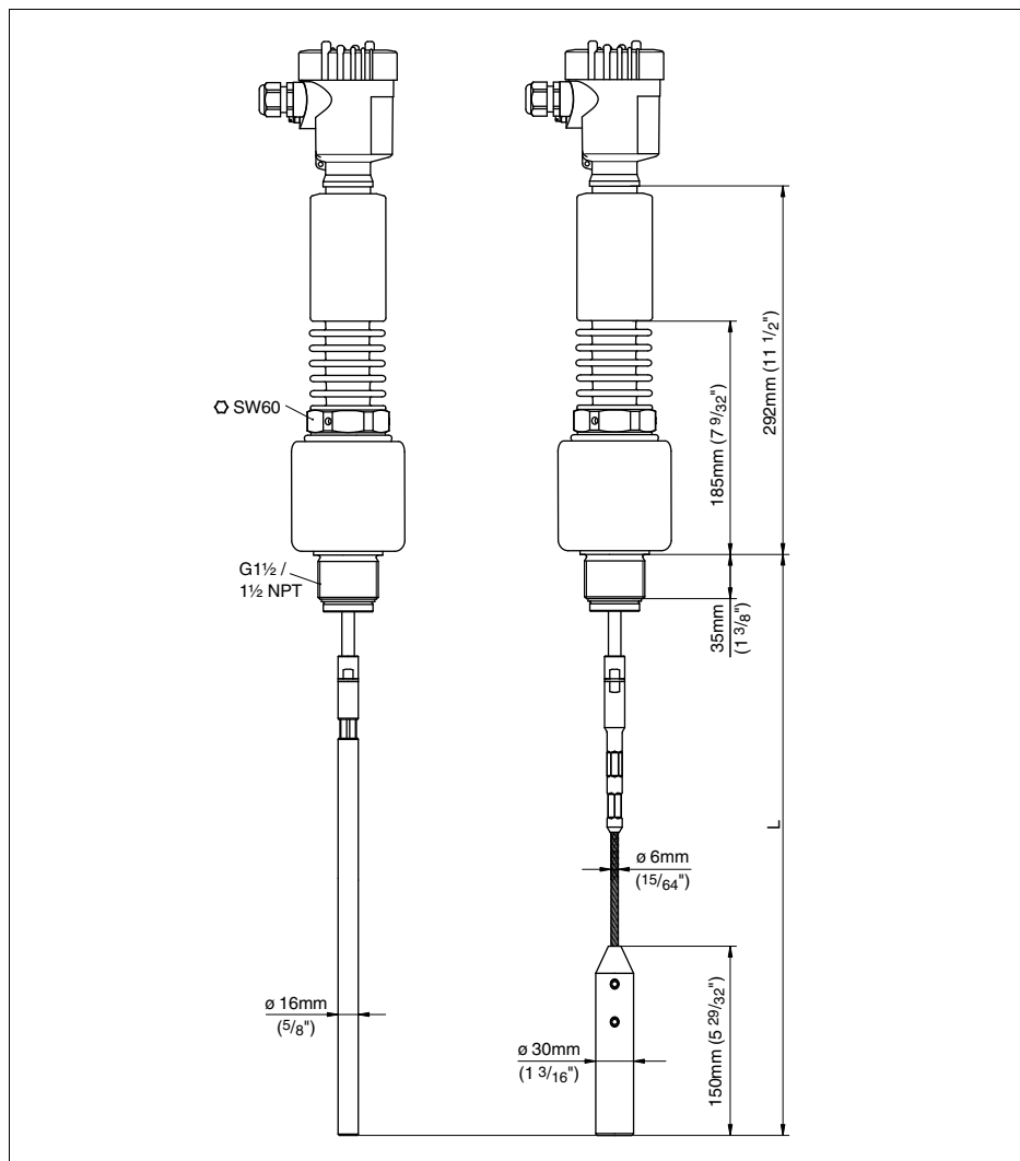
Рис. 33: VEGAFLEX 67, исполнение с тросом или стержнем, с резьбовым присоединением (-200 ... +400 °C/-328 ... +752 °F)
