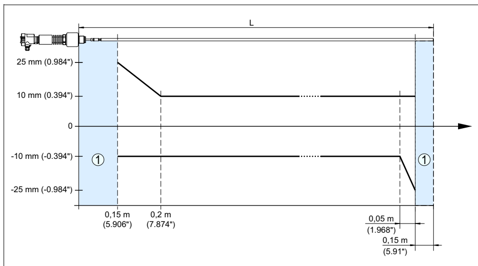
Рис. 22: Погрешность измерения VEGAFLEX 67 в стержневом исполнении
