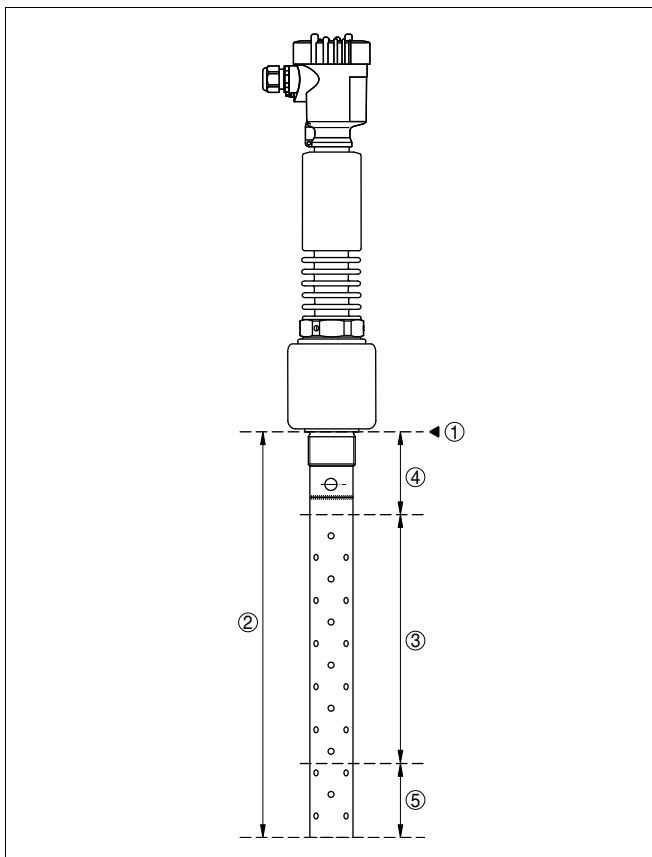
Рис. 18: Диапазон измерения VEGAFLEX 67 - коаксиальное исполнение
