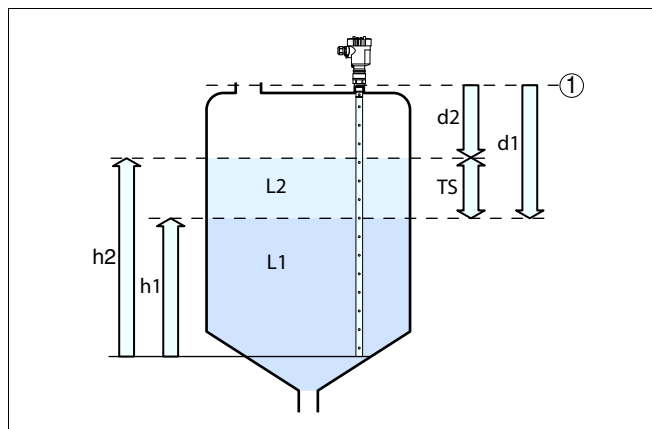
Рис. 21: Измерение межфазного уровня (раздел фаз находится между L1 и L2)
