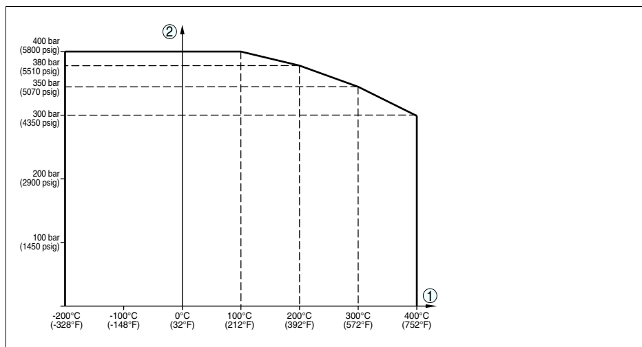
Рис. 25: Исполнение для высоких температур: давление процесса - температура процесса
