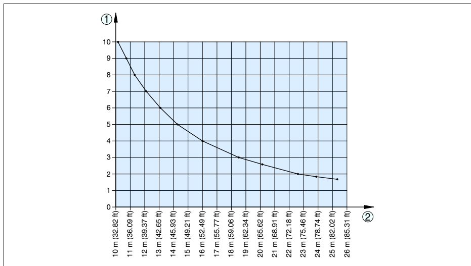
Рис. 20: Отношение диэлектрической постоянной ( \epsilon_r ) верхнего продукта к максимальной длине измерительного зонда
