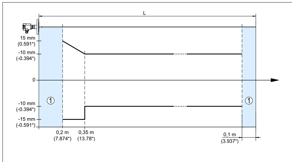
Рис. 20: Погрешность измерения VEGAFLEX 67 в стержневом исполнении
