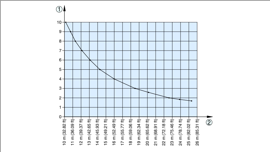
Рис. 18: Отношение диэлектрической постоянной ( \epsilon_r ) верхнего продукта к максимальной длине измерительного зонда
