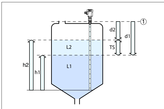
Рис. 19: Измерение межфазного уровня (раздел фаз находится между L1 и L2)
