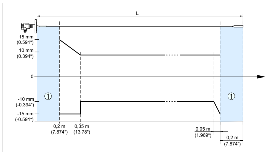
Рис. 21: Погрешность измерения VEGAFLEX 67 в тросовом исполнении
