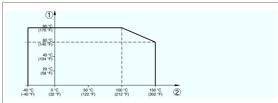
Рис. 22: Температура окружающей среды - Температура процесса
