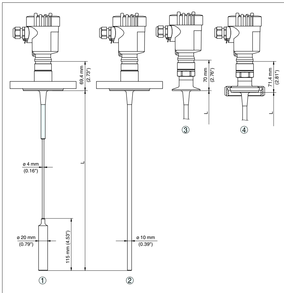
Рис. 29: VEGAFLEX 67, фланцевое исполнение
