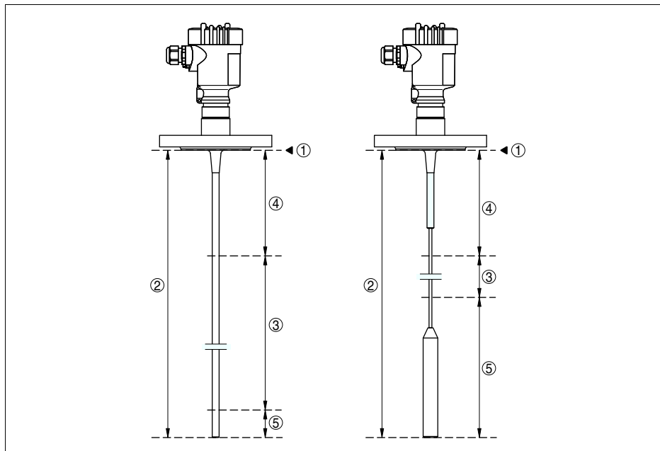
Рис. 17: Диапазон измерения VEGAFLEX 67 (исполнение с тросом или стержнем)
