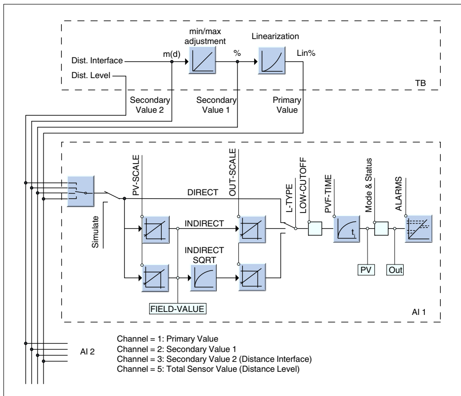
Рис. 23: Обработка измеренных значений VEGAFLEX 67
