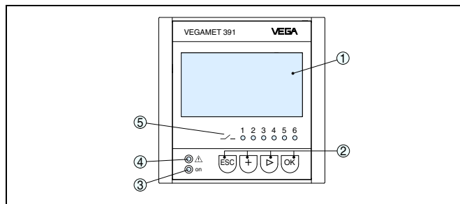
Рис. 19: Элементы индикации и настройки
