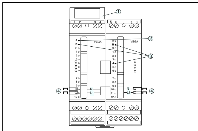
Рис. 10: Разъем VEGAMET
