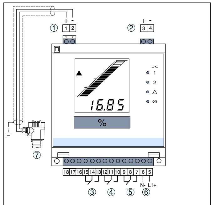
Рис. 12: Схема подключения с двухпроводным датчиком
