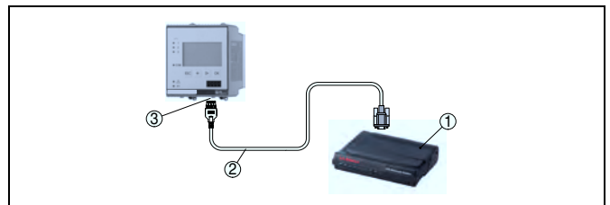
Рис. 25: Подключение модема через RS232
