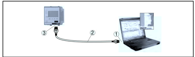
Рис. 23: Подключение ПК через Ethernet
