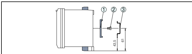
Рис. 6: Монтаж на несущей рейке
