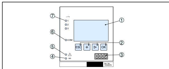
Рис. 20: Элементы индикации и настройки
