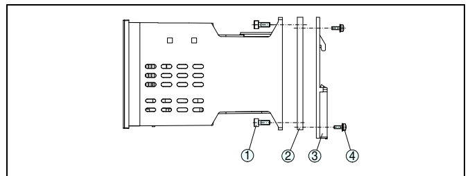
Рис. 9: Монтаж на несущей рейке
