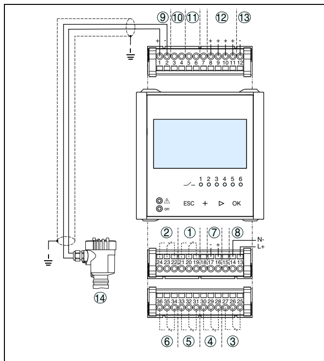
Рис. 14: Схема подключения с двухпроводным датчиком
