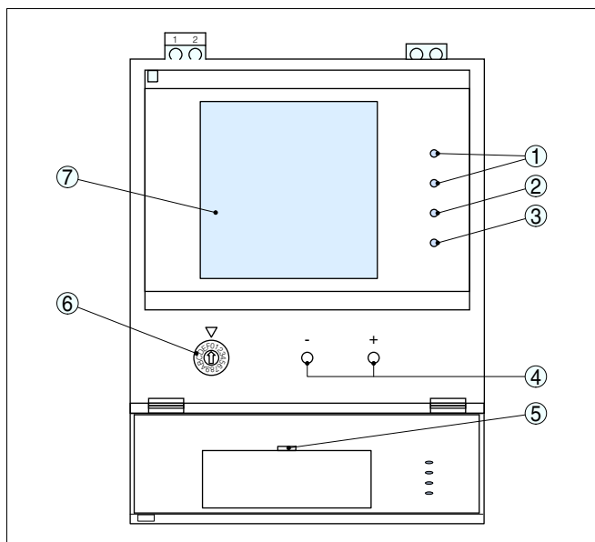
Рис. 1: VEGAMET 381 Ex
