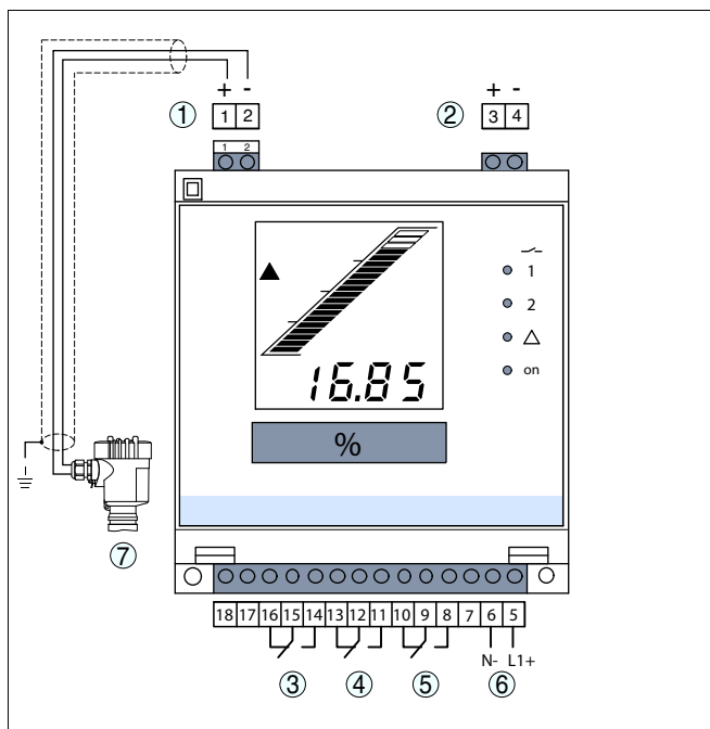
Рис. 6: Схема подключения и двухпроводного датчика
