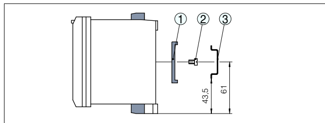
Рис. 4: Монтаж на несущей рейке
