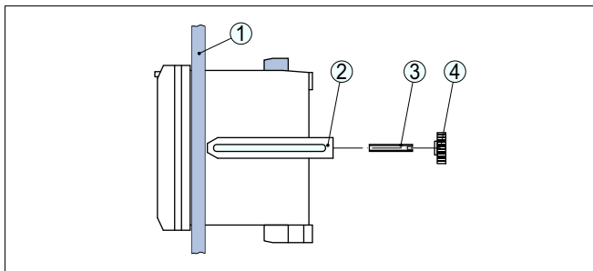
Рис. 2: Монтаж на панели
