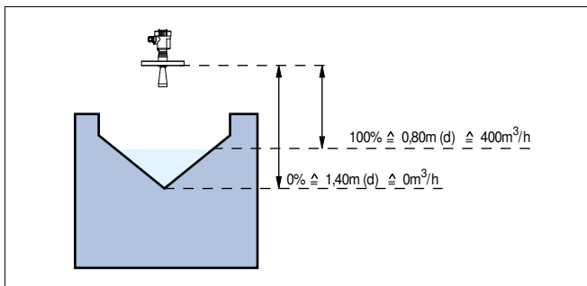
Рис. 13: Установка для измерения расхода с треугольным водосливом
