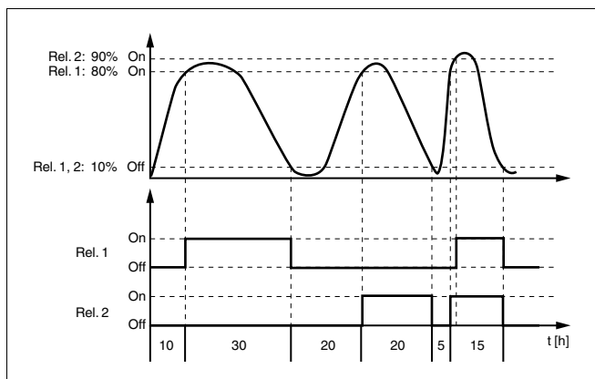
Рис. 10: Пример управления насосами 2
