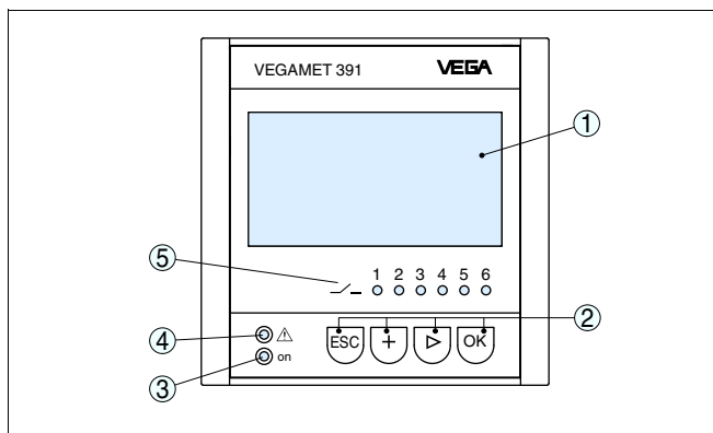
Рис. 7: Элементы индикации и настройки
