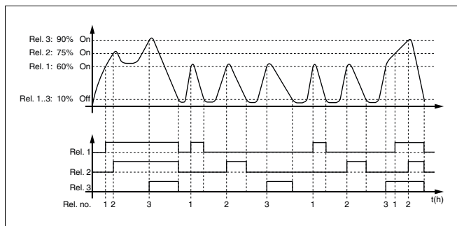
Рис. 11: Пример управления насосами 4
