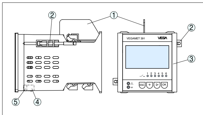
Рис. 1: VEGAMET 391
