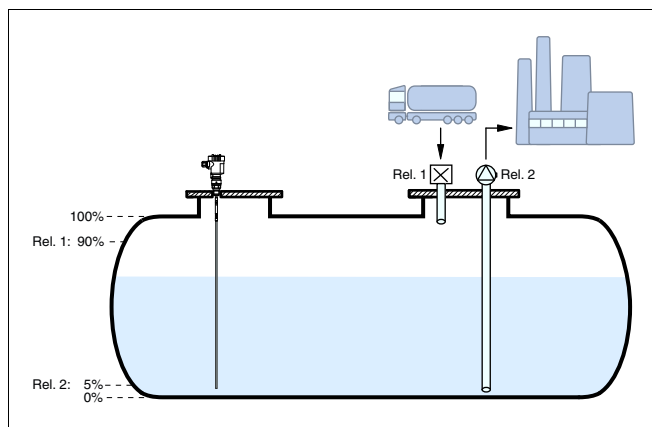
Рис. 9: Пример измерения уровня в горизонтальной цилиндрической емкости
