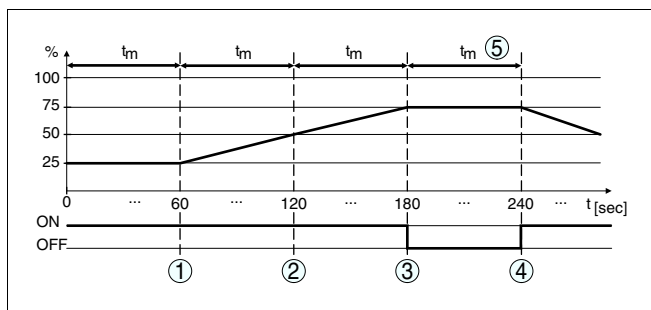
Рис. 12: Пример сигнализации тенденции
