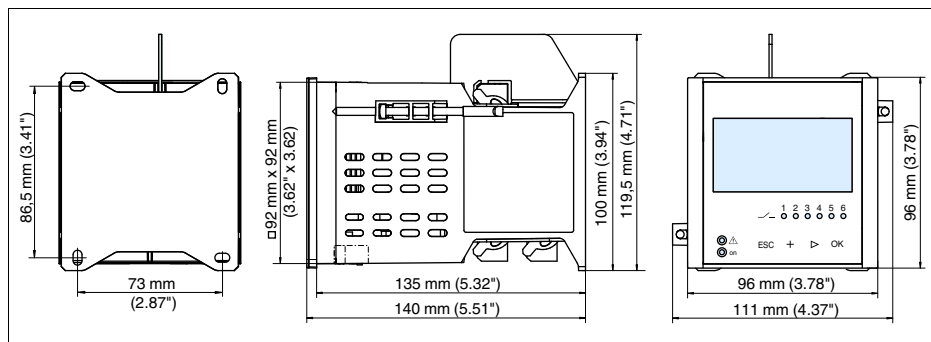
Рис. 14: Размеры VEGAMET 391
