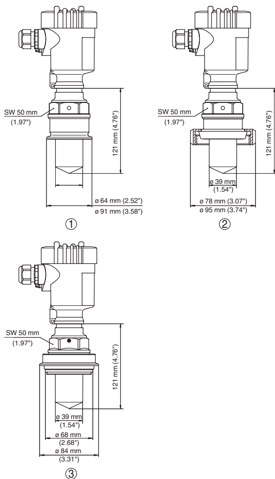
Рис. 65: VEGAPULS 61, гигиеническое присоединение
