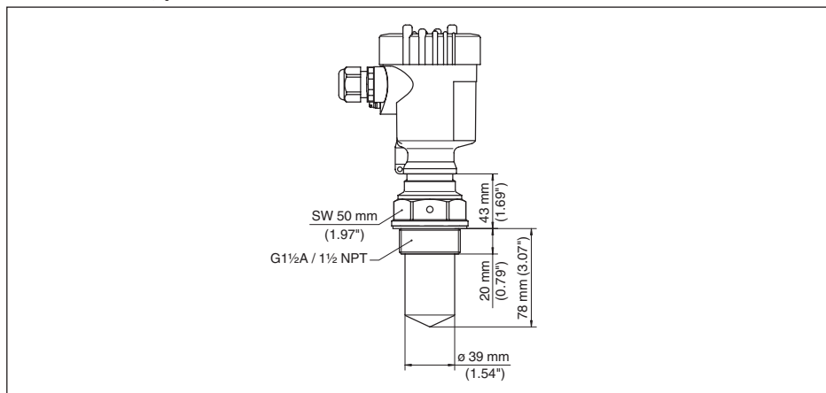
Рис. 64: VEGAPULS 61, резьбовое исполнение G1 1/2 и 1 1/2 NPT
