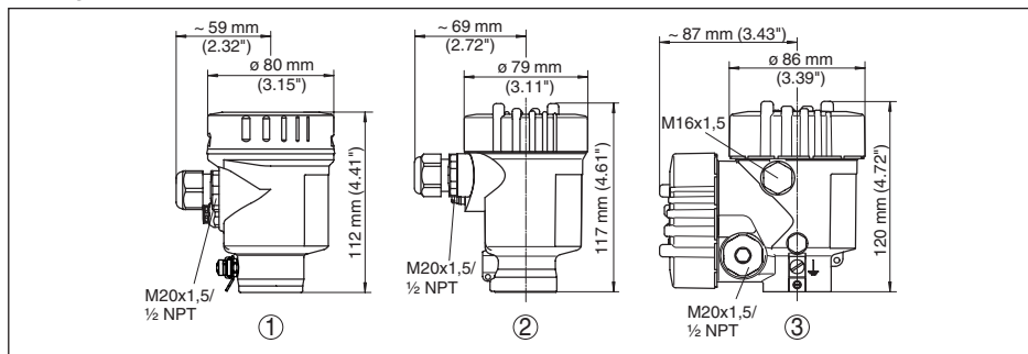
Рис. 62: Корпуса в исполнении IP 66/IP 68 (0,2 bar) - с установленным модулем индикации и настройки корпус выше на 9 mm/0.35 in
