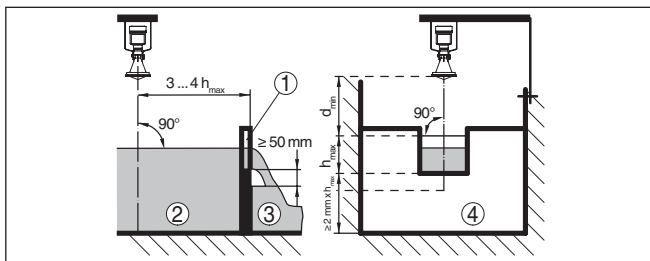
Рис. 22: Измерение расхода с прямоугольным водосливом: d_{min} = минимальное расстояние датчика (см. гл. "Технические данные"); h_{max} = max. заполнение прямоугольного водослива
