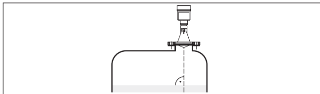
Рис. 17: Ориентация датчика на жидкостях
