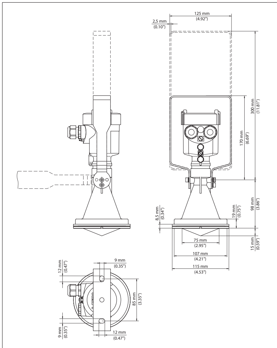
Рис. 66: VEGAPULS 61, монтажная скоба длиной 170 или 300 мм
