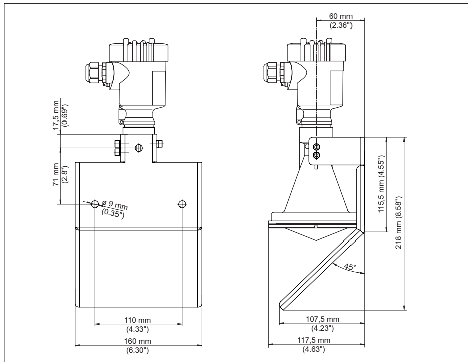
Рис. 74: VEGAPULS 61, монтажная скоба и отражатель
