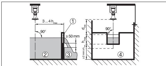
Рис. 22: Измерение расхода с прямоугольным водосливом: d_{min} = минимальное расстояние датчика (см. гл. "Технические данные"); h_{max} = максимальное заполнение прямоугольного водослива
