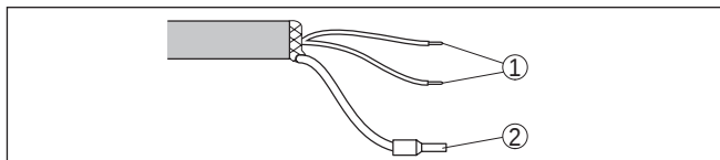
Рис. 32: Назначение проводов постоянно подключенного соединительного кабеля
