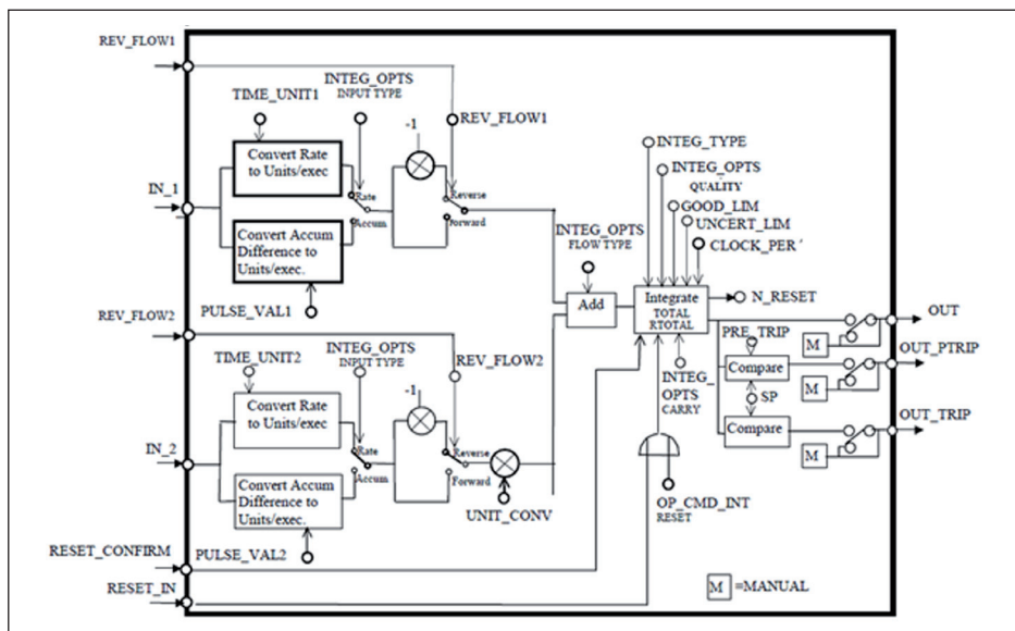
Рис. 63: Схема функционального блока Integrator
