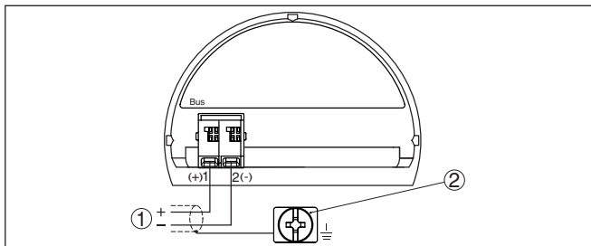
Рис. 30: Отсек подключения (двухкамерный корпус Ex d)
