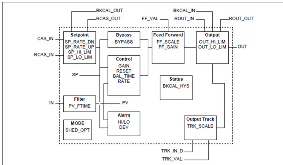
Рис. 60: Схема функционального блока PID Control
