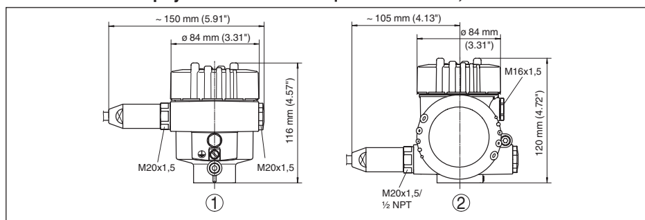
Рис. 68: Корпуса в исполнении IP 66/IP 68 (1 bar) - с установленным модулем индикации и настройки корпус выше на 9 mm/0.35 in
