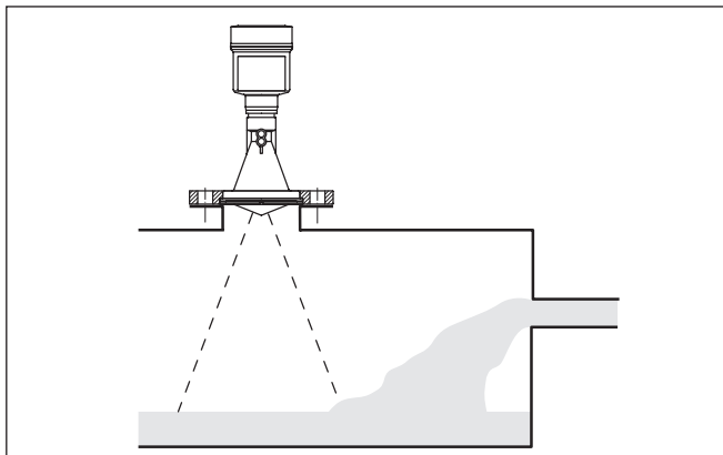
Рис. 11: Монтаж радарного датчика при втекающем продукте
