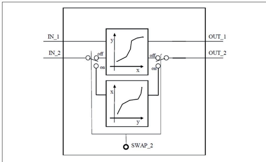
Рис. 62: Схема функционального блока Signal Characterizer
