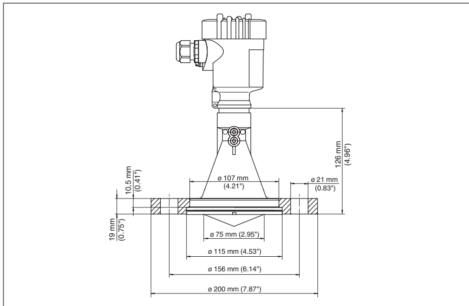
Рис. 75: VEGAPULS 61, накидной фланец для DN 80 PN 16/ ASME 3" 150lbs/ JIS80 10K
