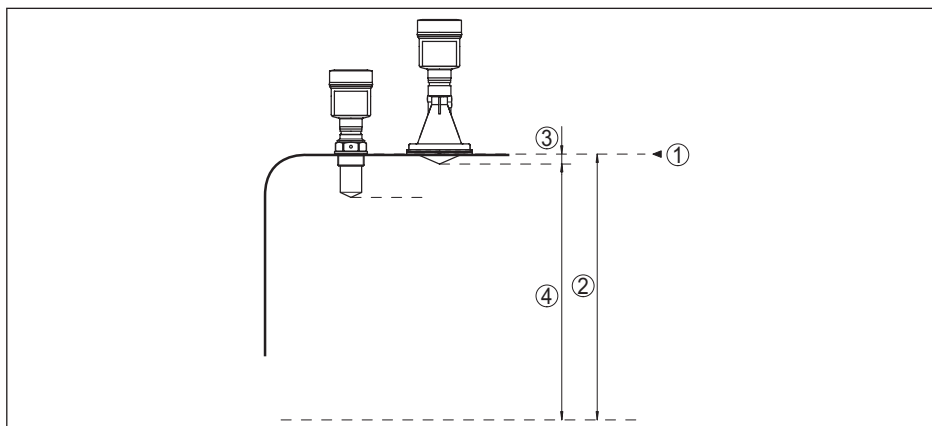
Рис. 54: Данные для входной величины
