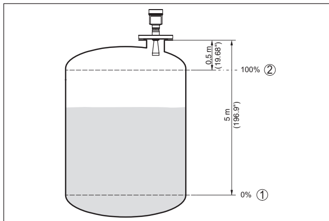
Рис. 36: Пример выполнения Установки Min./Max.
