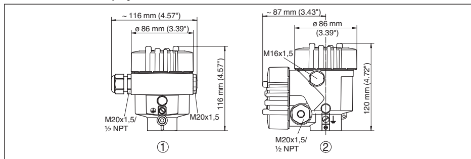
Рис. 67: Корпуса в исполнении IP 66/IP 68 (0,2 bar) - с установленным модулем индикации и настройки корпус выше на 9 mm/0.35 in
