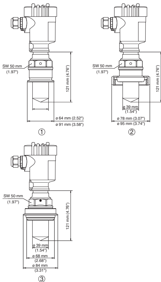
Рис. 72: VEGAPULS 61, гигиеническое присоединение
