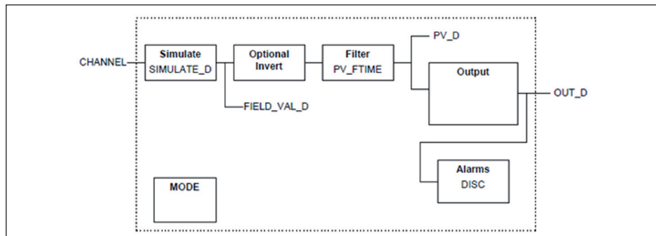
Рис. 59: Схема функционального блока Discret Input (DI)
