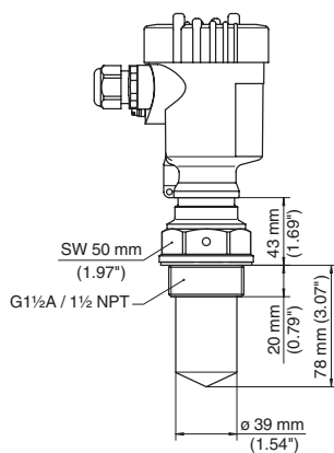
Рис. 71: VEGAPULS 61, резьбовое исполнение G1½ и 1½ NPT
