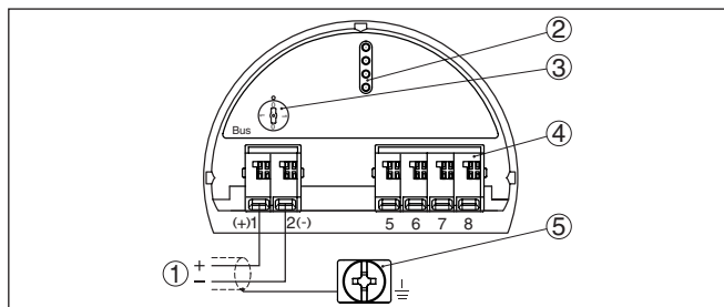
Рис. 25: Отсек электроники и подключения (однокамерный корпус)
