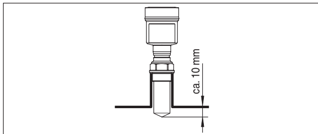
Рис. 15: Рекомендуемая высота монтажного патрубка
