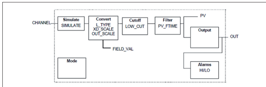
Рис. 58: Схема функционального блока Analog Input (AI)
