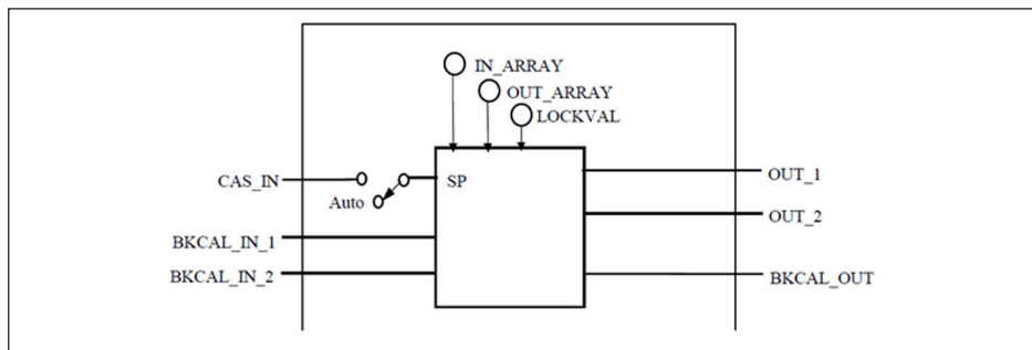
Рис. 61: Схема функционального блока Output Splitter
