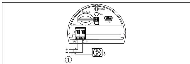
Рис. 28: Подключение модуля мобильной связи к питанию
