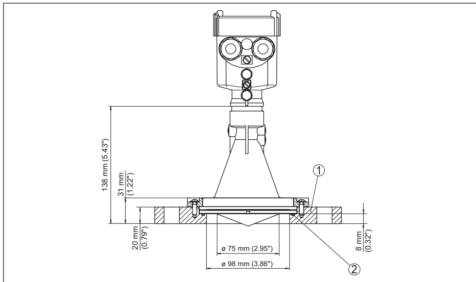
Рис. 76: VEGAPULS 61, адаптерный фланец
