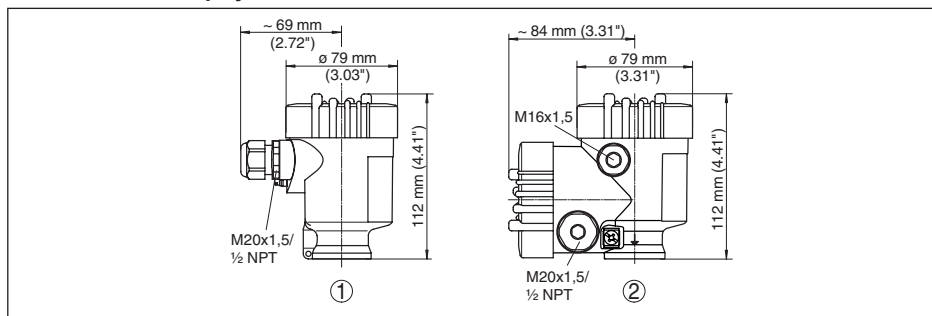
Рис. 66: Корпуса в исполнении IP 66/IP 68 (0,2 bar) - с установленным модулем индикации и настройки корпус выше на 9 mm/0.35 in
