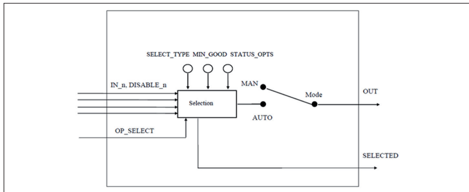
Рис. 64: Схема функционального блока Input Selector
