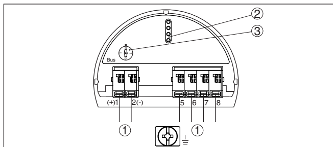
Рис. 26: Отсек электроники (двухкамерный корпус)
