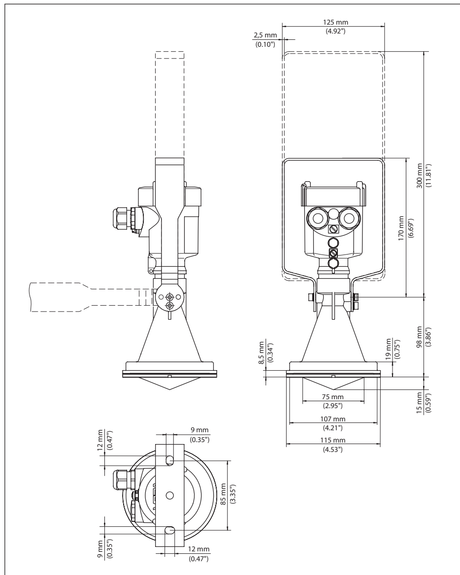
Рис. 73: VEGAPULS 61, монтажная скоба длиной 170 или 300 мм
