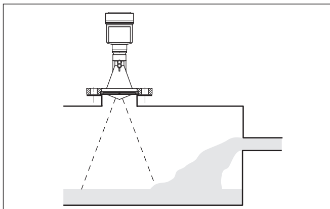
Рис. 12: Монтаж радарного датчика при втекающем продукте
