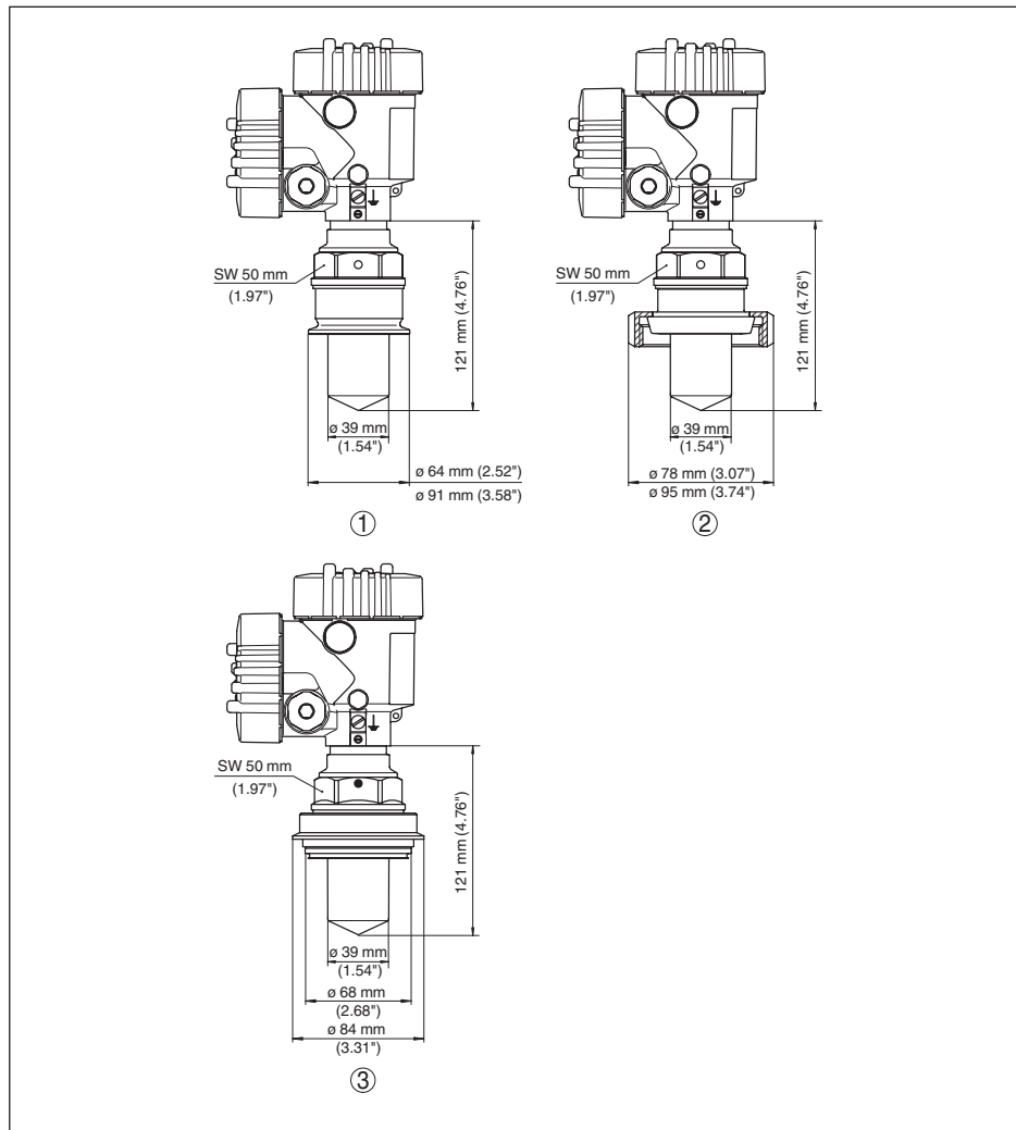
Рис. 62: VEGAPULS 61, гигиеническое присоединение
