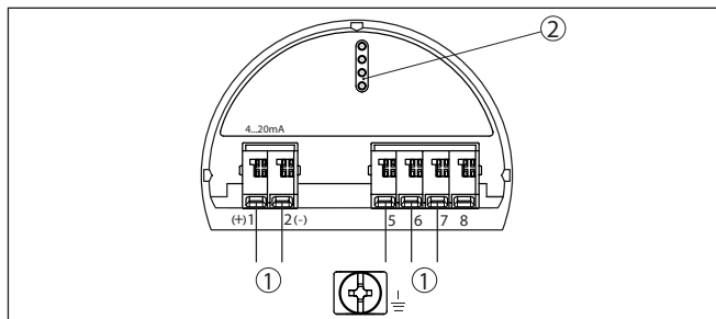
Рис. 27: Отсек электроники (двухкамерный корпус)
