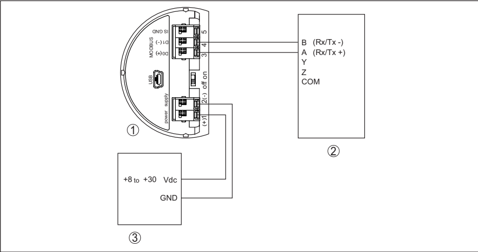
Рис. 55: Подключение VEGAPULS 61 к RTU Fisher ROC 809
