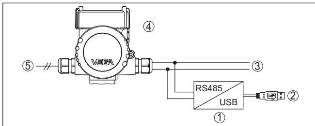
Рис. 34: Подключение ПК через интерфейсный адаптер к кабелю RS 485
