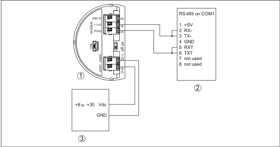
Рис. 58: Подключение VEGAPULS 61 к RTU Bristol ControlWave Micro
