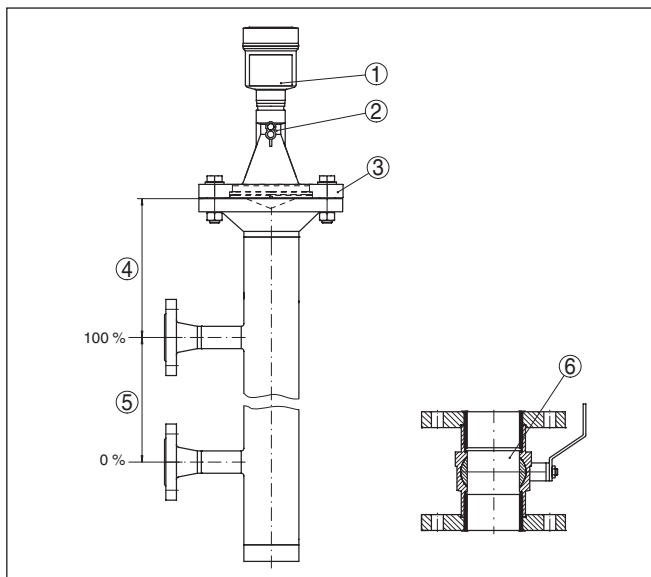
Рис. 22: Монтаж в выносной трубе
