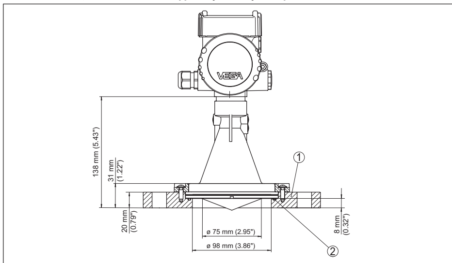
Рис. 65: VEGAPULS 61, адаптерный фланец
