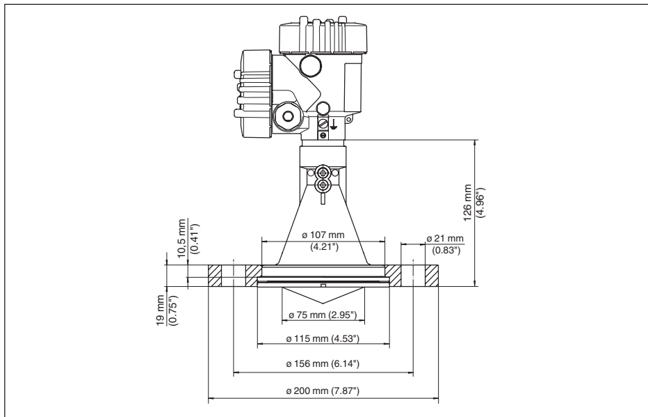
Рис. 64: VEGAPULS 61, накидной фланец для DN 80 PN 16/ ASME 3" 150lbs/ JIS80 10K
