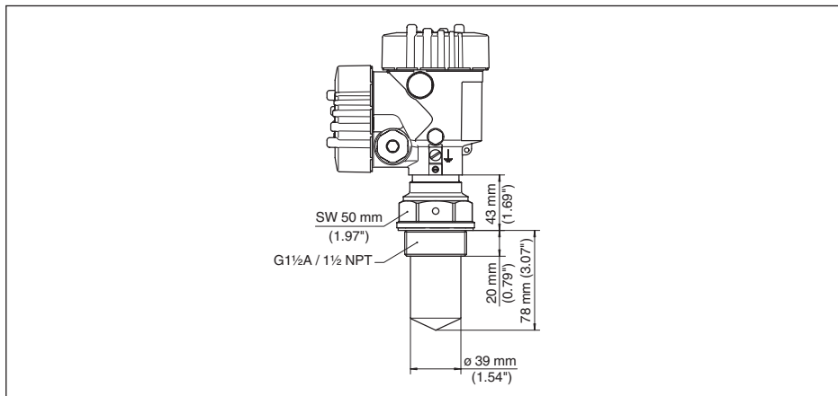
Рис. 61: VEGAPULS 61, резьбовое исполнение G1½ и 1½ NPT
