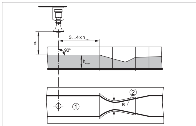
Рис. 24: Измерение расхода с лотком Хафаги-Вентури: d = минимальное расстояние датчика; h_{max} = максимальное заполнение лотка; B = наибольшее сужение лотка
