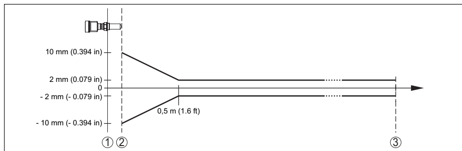
Рис. 52: Погрешность измерения при эталонных условиях - герметизированная антенная система
