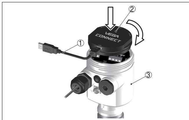
Рис. 32: Подключение ПК через интерфейсный адаптер прямо к датчику
