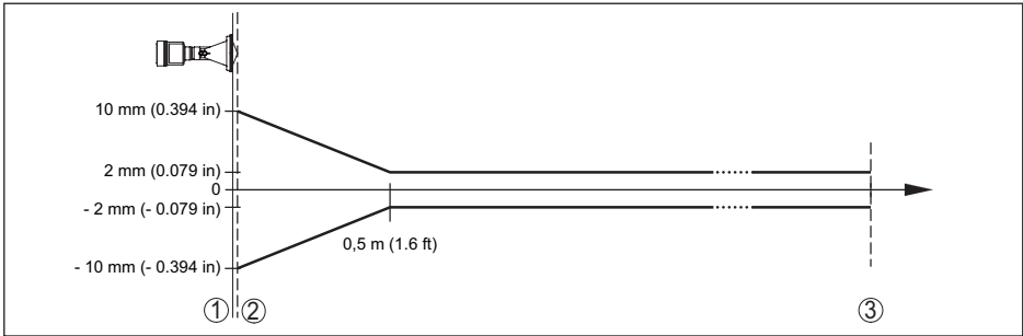
Рис. 53: Погрешность измерения при эталонных условиях - пластиковая рупорная антенна
