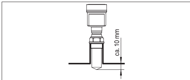
Рис. 16: Рекомендуемая высота монтажного патрубка
