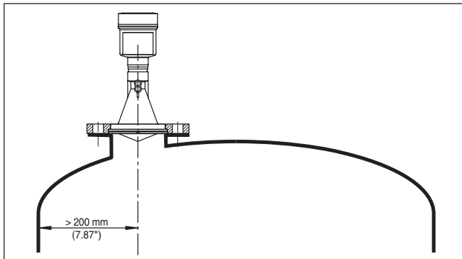
Рис. 10: Монтаж радарного датчика на округлой крыше емкости
