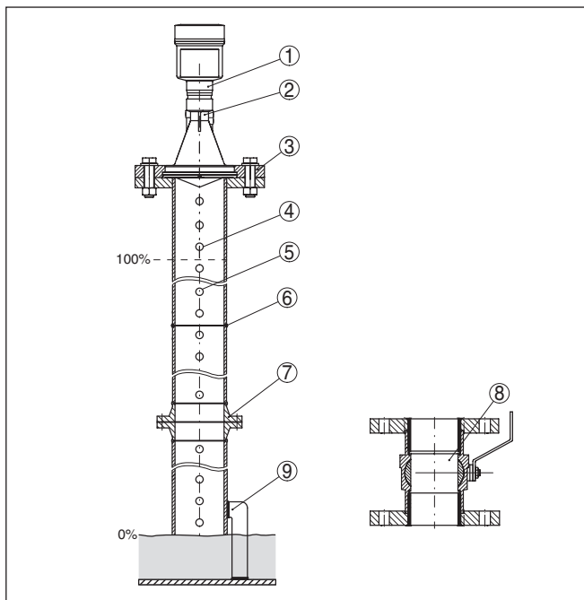
Рис. 21: Монтаж в уравнильной трубе
