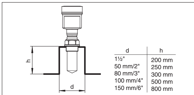
Рис. 17: Ориентировочные размеры патрубков
