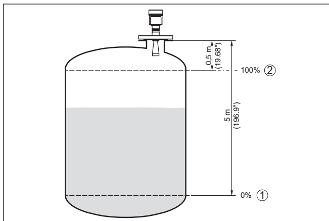
Рис. 31: Пример выполнения Установки Min./Max.
