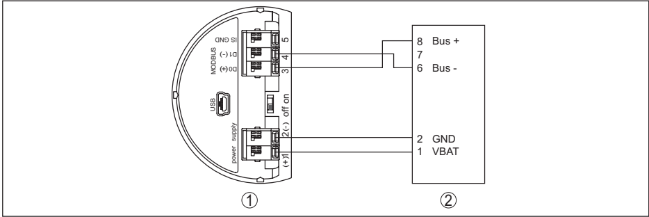
Рис. 56: Подключение VEGAPULS 61 к RTU ABB Total Flow
