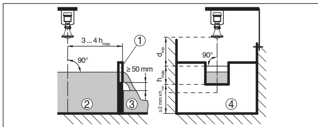
Рис. 23: Измерение расхода с прямоугольным водосливом: d_{min} = минимальное расстояние датчика (см. гл. "Технические данные"); h_{max} = max. наполнение прямоугольного водослива
