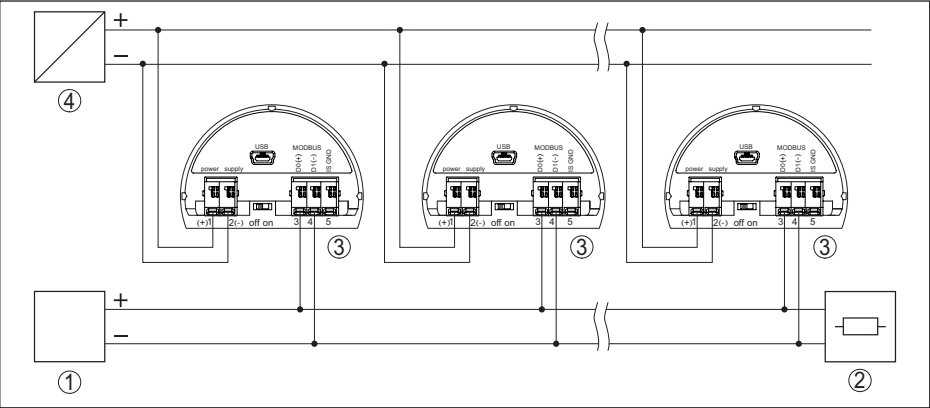
Рис. 54: Архитектура шины Modbus
