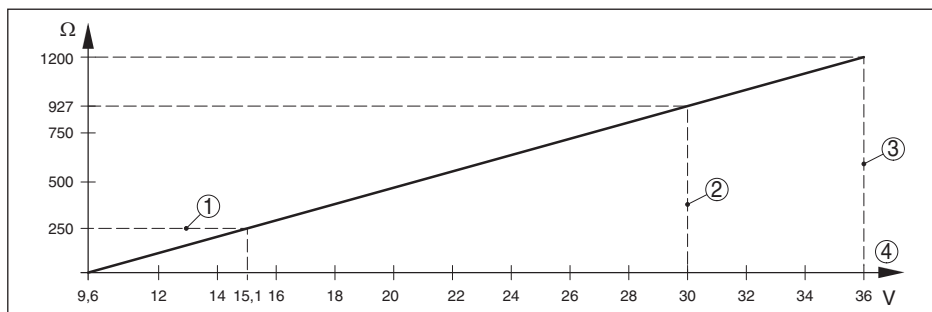
Рис. 57: Диаграмма напряжения
