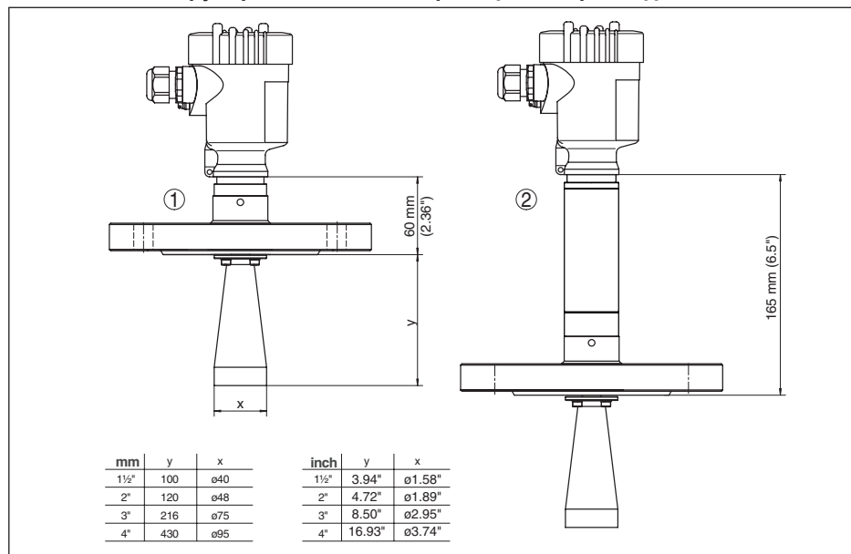
Рис. 64: VEGAPULS 62, с рупорной антенной и фланцевым присоединением
