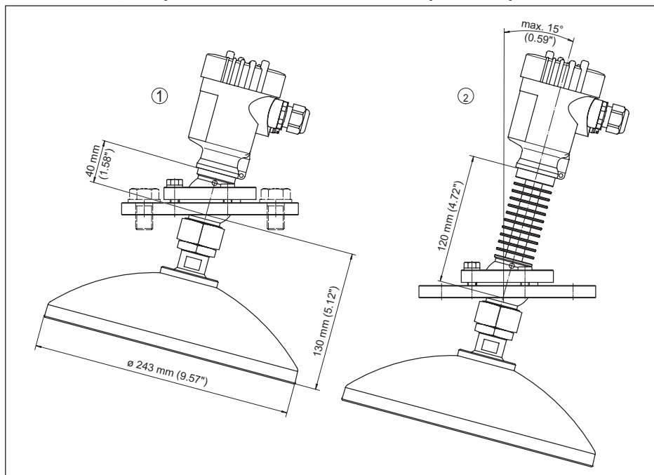
Рис. 67: VEGAPULS 62, с параболической антенной и поворотным креплением
