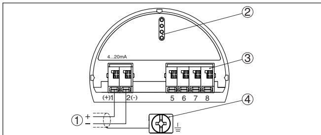
Рис. 25: Отсек электроники и подключения (однокамерный корпус)
