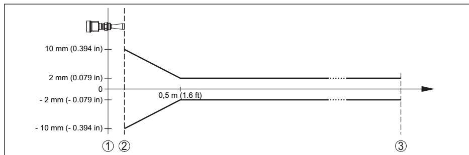
Рис. 56: Погрешность измерения при эталонных условиях
