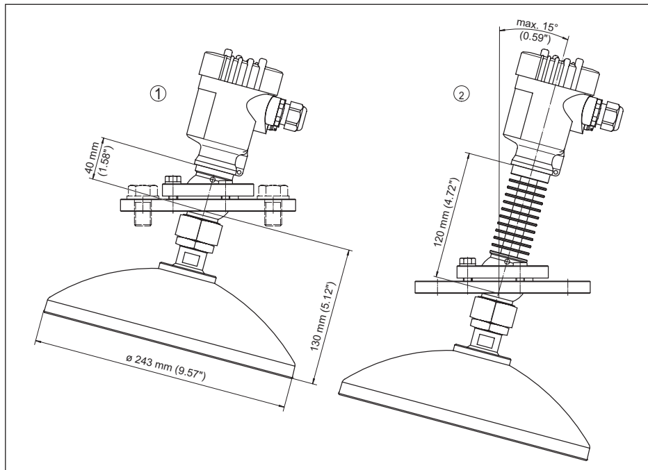
Рис. 75: VEGAPULS 62, с параболической антенной и поворотным креплением
