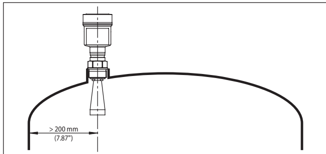
Рис. 8: Монтаж радарного датчика на округлой крыше емкости
