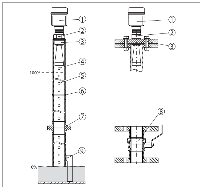
Рис. 19: Монтаж в уравнильной трубе
