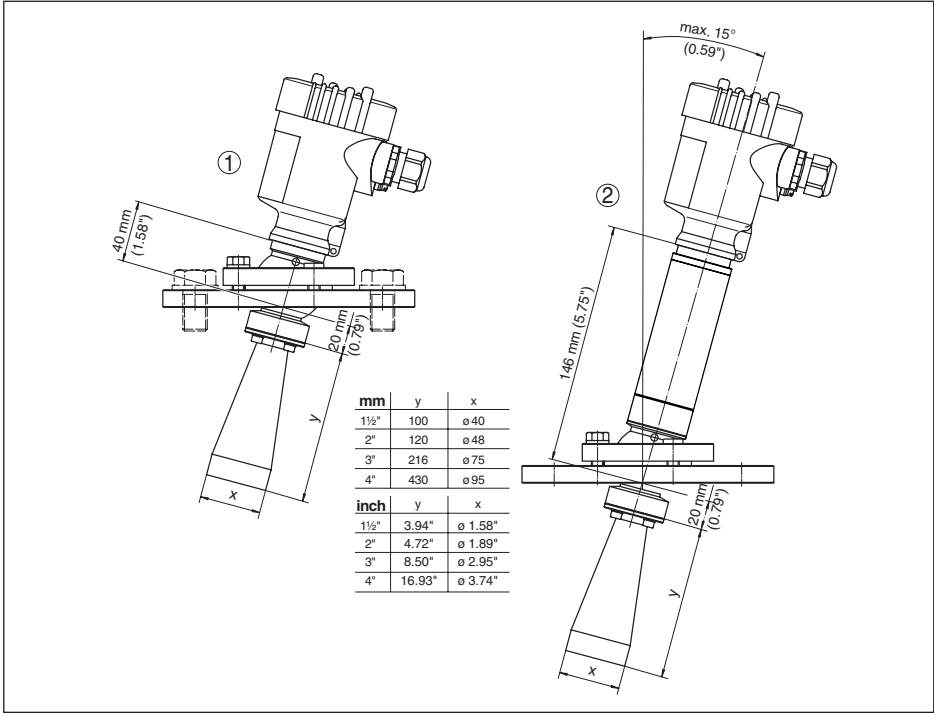
Рис. 74: VEGAPULS 62, с рупорной антенной и поворотным креплением
