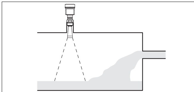
Рис. 10: Монтаж радарного датчика при втекающем продукте
