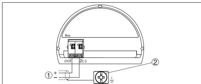
Рис. 31: Отсек подключения (двухкамерный корпус Ex d)
