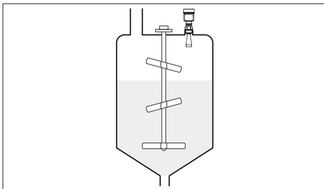
Рис. 18: Мешалки
