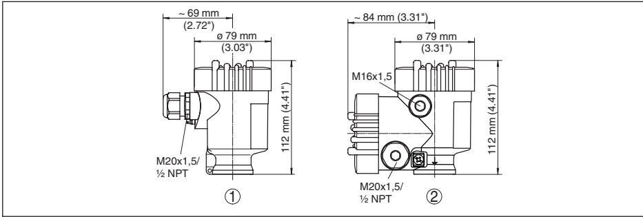
Рис. 66: Корпуса в исполнении IP 66/IP 68 (0,2 bar) - с установленным модулем индикации и настройки корпус выше 9 mm/0.35 in
