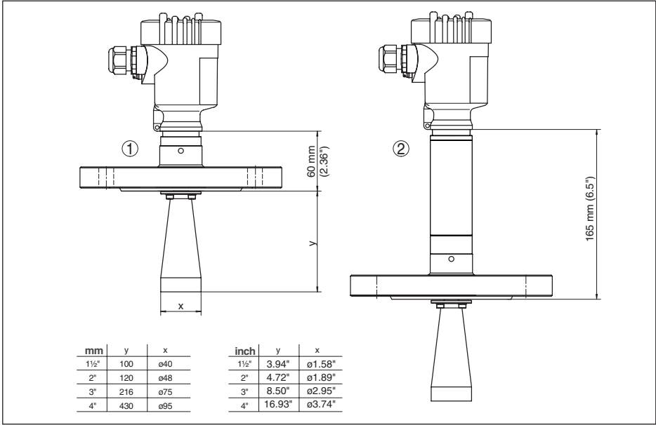
Рис. 72: VEGAPULS 62, с рупорной антенной и фланцевым присоединением
