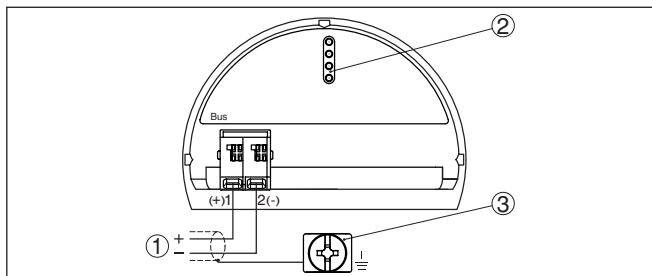
Рис. 28: Отсек подключения (двухкамерный корпус)
