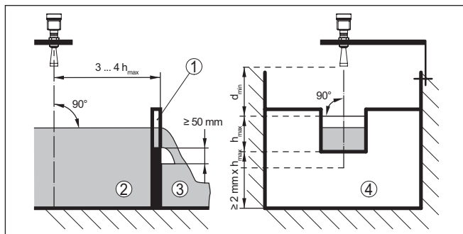
Рис. 23: Измерение расхода с прямоугольным водосливом: d_{min.} = минимальное расстояние датчика (см. гл. "Технические данные"); h_{max.} = max. заполнение прямоугольного водослива
