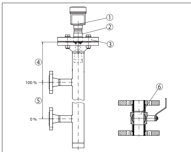
Рис. 20: Монтаж в выносной трубе
