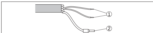
Рис. 33: Назначение проводов постоянно подключенного соединительного кабеля
