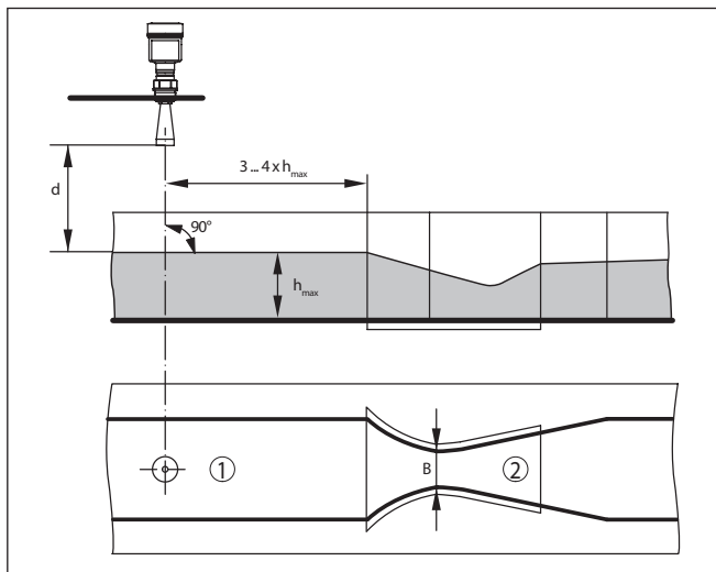
Рис. 24: Измерение расхода с лотком Хафаги-Вентури: d = минимальное расстояние датчика; h_{\max} = максимальное заполнение лотка; B = наибольшее сужение лотка
