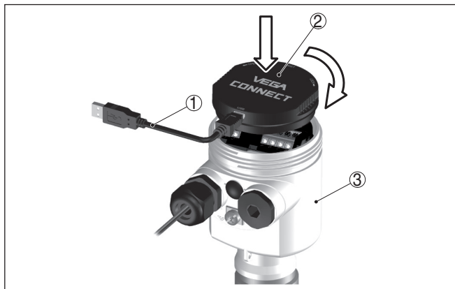
Рис. 38: Подключение ПК через интерфейсный адаптер прямо к датчику
