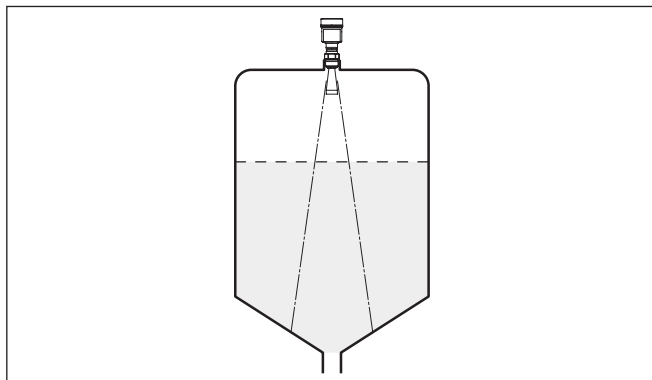
Рис. 9: Монтаж радарного датчика на емкостях с коническим дном
