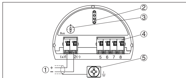
Рис. 26: Отсек электроники и подключения (однокамерный корпус)
