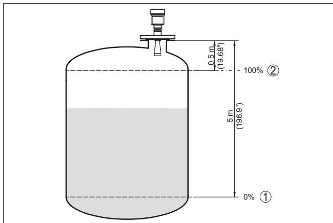
Рис. 37: Пример выполнения Установки Min./Max.
