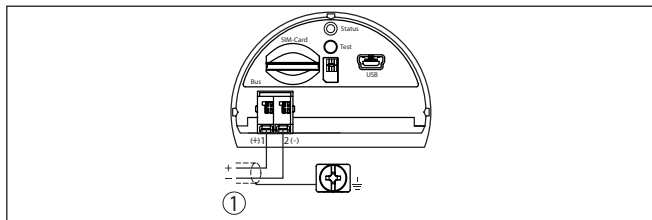
Рис. 29: Подключение модуля мобильной связи к питанию
