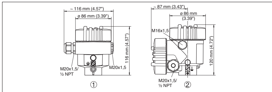
Рис. 61: Корпуса в исполнении IP 66/IP 68 (0,2 bar) - с установленным модулем индикации и настройки корпус выше на 9 mm/0.35 in
