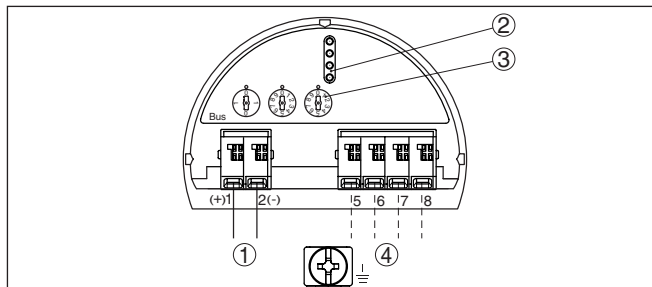
Рис. 29: Отсек электроники (двухкамерный корпус)
