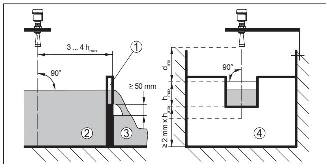
Рис. 22: Измерение расхода с прямоугольным водосливом: d_{min} = минимальное расстояние датчика (см. гл. "Технические данные"); h_{max} = max. заполнение прямоугольного водослива
