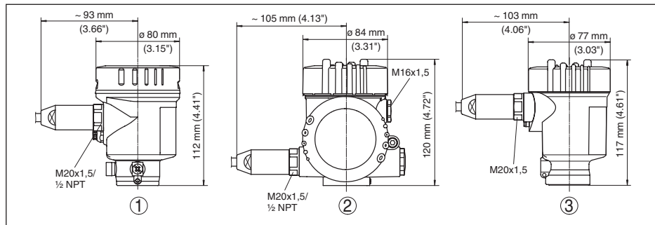
Рис. 64: Корпуса в исполнении IP 66/IP 68 (1 bar) - с установленным модулем индикации и настройки корпус выше на 9 mm/0.35 in
