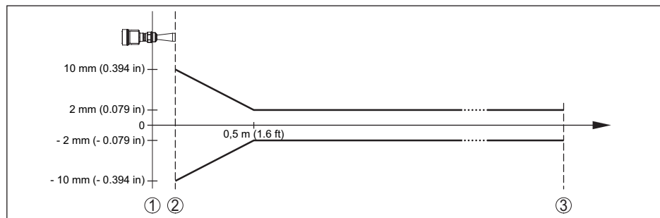
Рис. 56: Погрешность измерения при эталонных условиях
