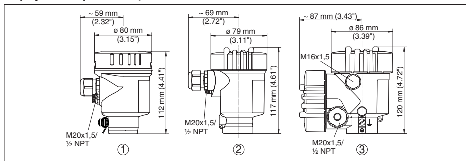
Рис. 63: Корпуса в исполнении IP 66/IP 68 (0,2 bar) - с установленным модулем индикации и настройки корпус выше на 9 mm/0.35 in
