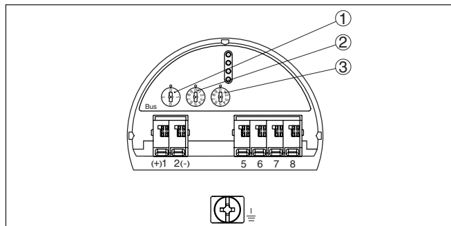
Рис. 33: Переключатели выбора адреса
