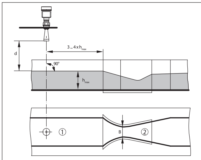
Рис. 23: Измерение расхода с лотком Хафаги-Вентури: d = минимальное расстояние датчика; h_{max} = максимальное заполнение лотка; B = наибольшее сужение лотка
