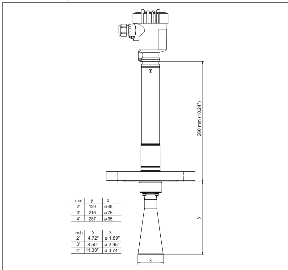
Рис. 67: VEGAPULS 62, с рупорной антенной и фланцевым присоединением, с температурной вставкой до 450 °C
