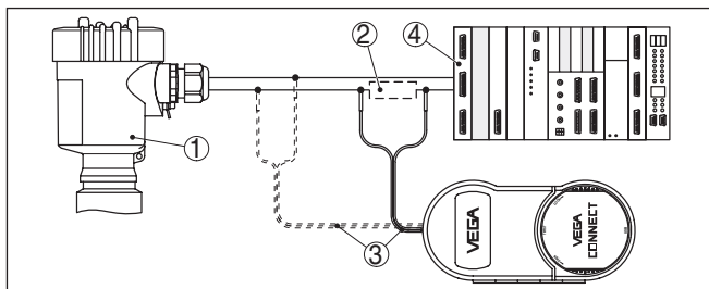
Рис. 29: Подключение ПК к сигнальному кабелю через HART
