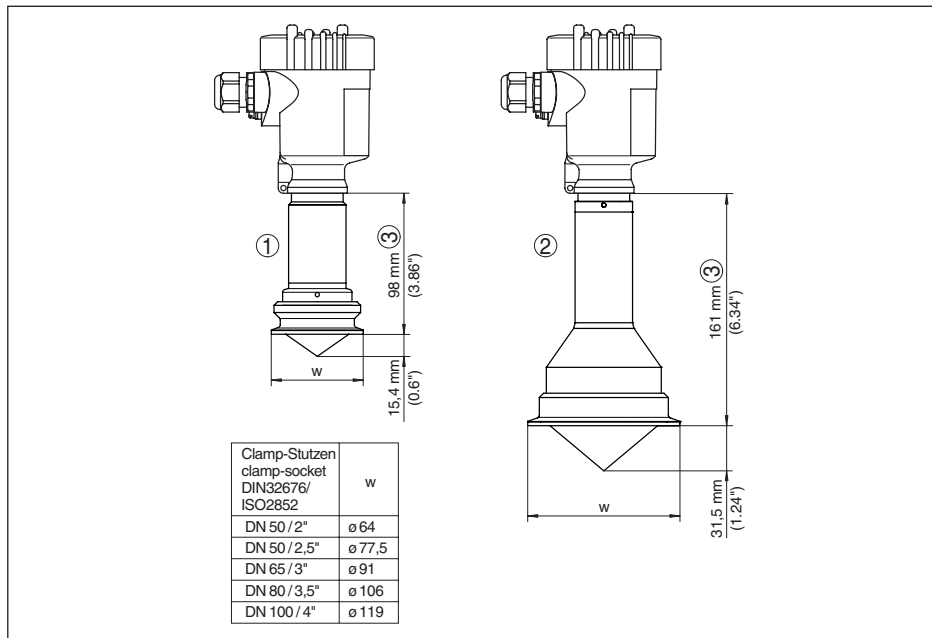
Рис. 57: VEGAPULS 63, гигиеническое присоединение 2
