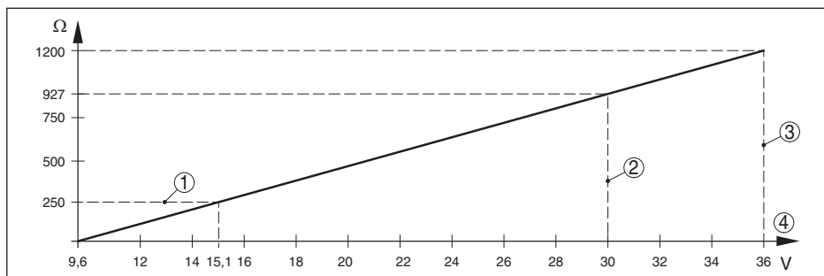
Рис. 48: Диаграмма напряжения
