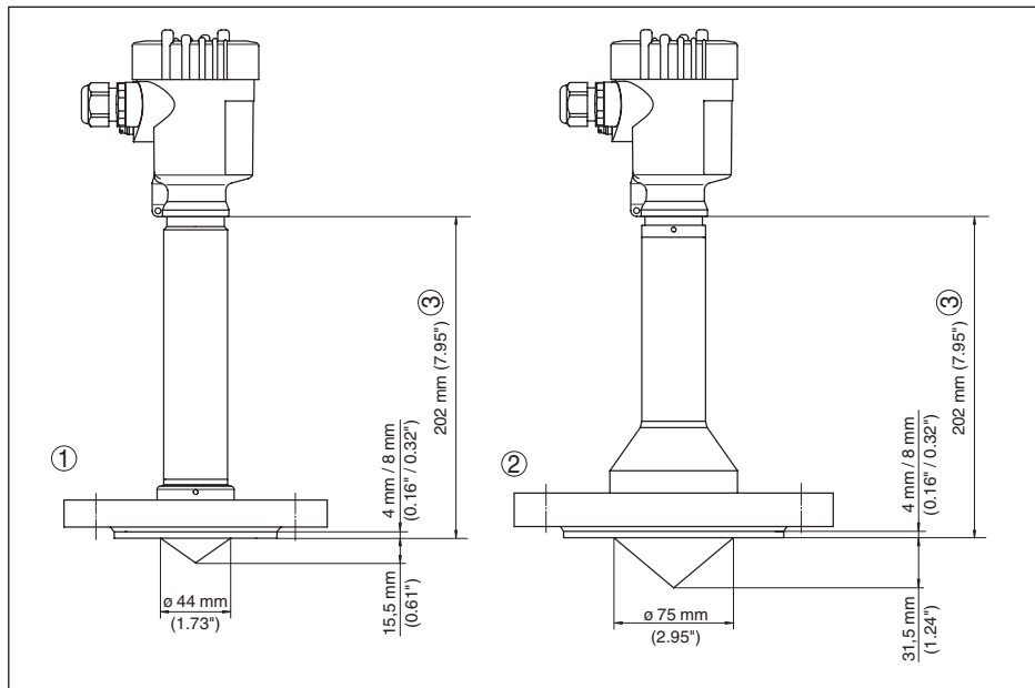
Рис. 55: VEGAPULS 63, фланцевое исполнение, для низких температур
