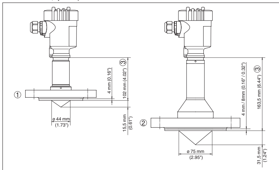
Рис. 54: VEGAPULS 63, фланцевое исполнение
