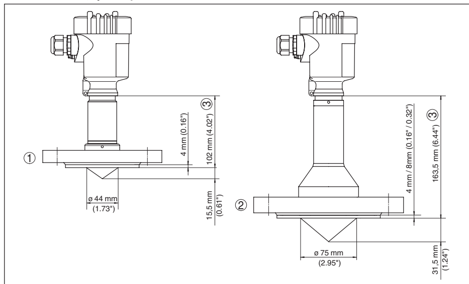
Рис. 61: VEGAPULS 63, фланцевое исполнение
