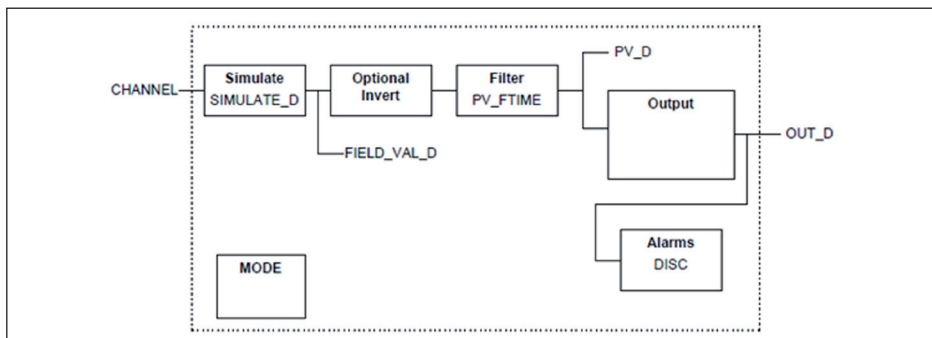
Рис. 49: Схема функционального блока Discret Input (DI)
