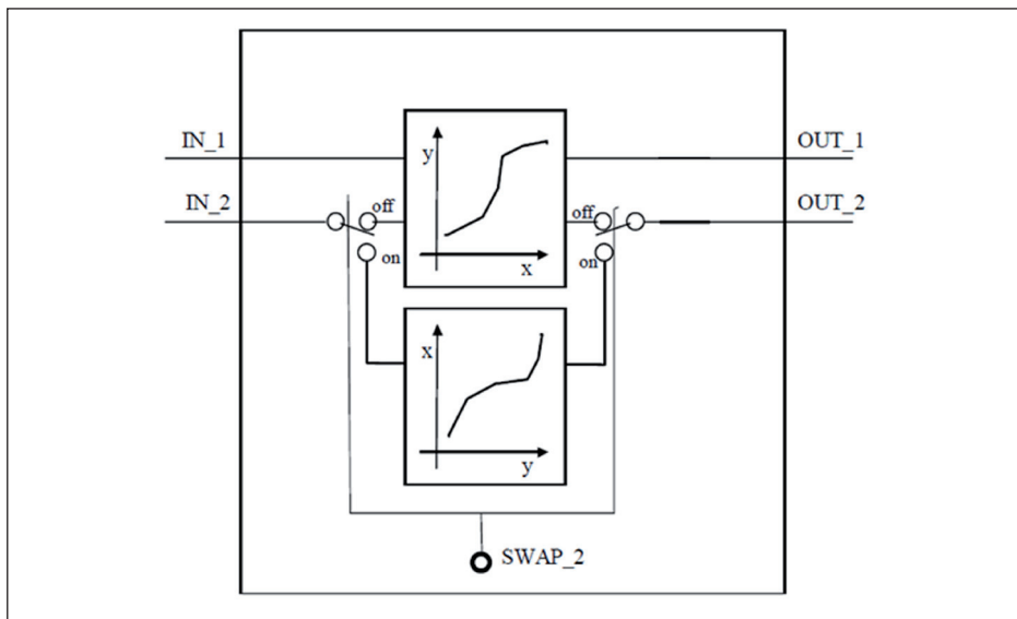
Рис. 52: Схема функционального блока Signal Characterizer
