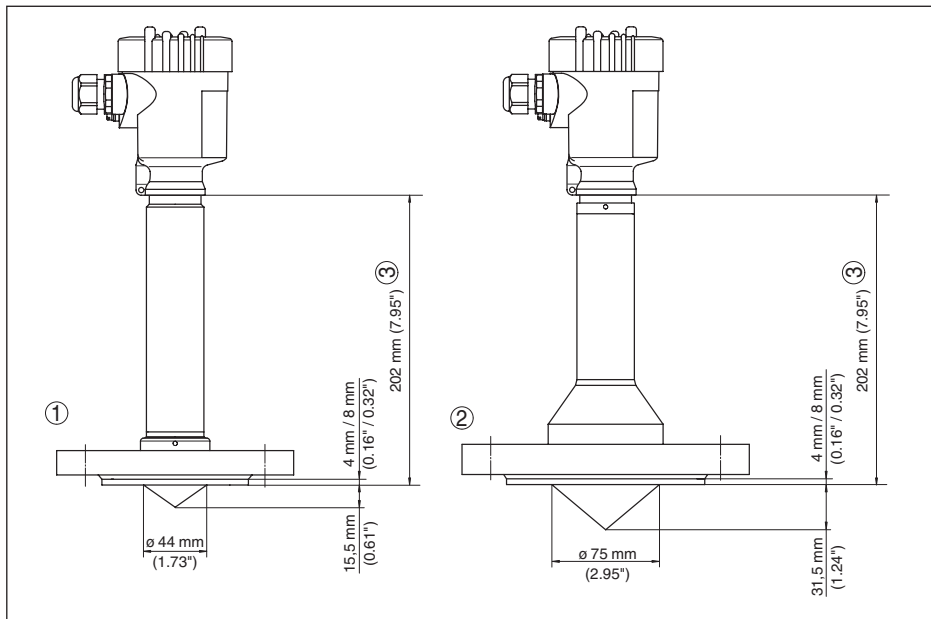
Рис. 62: VEGAPULS 63, фланцевое исполнение, для низких температур
