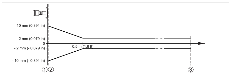
Рис. 46: Погрешность измерения при эталонных условиях
