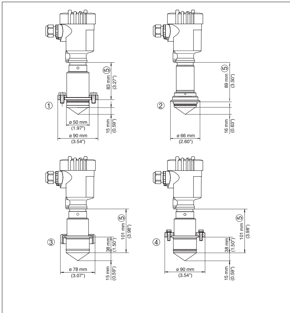
Рис. 63: VEGAPULS 63, гигиеническое присоединение 1
