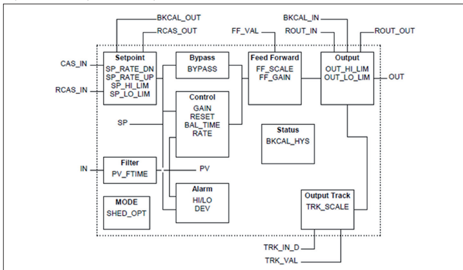
Рис. 50: Схема функционального блока PID Control
