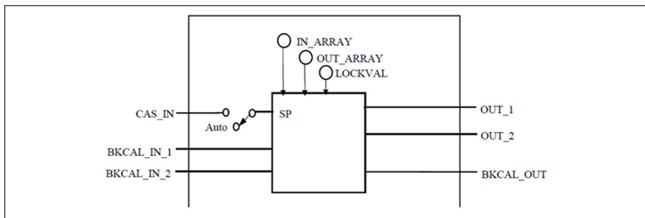
Рис. 51: Схема функционального блока Output Splitter
