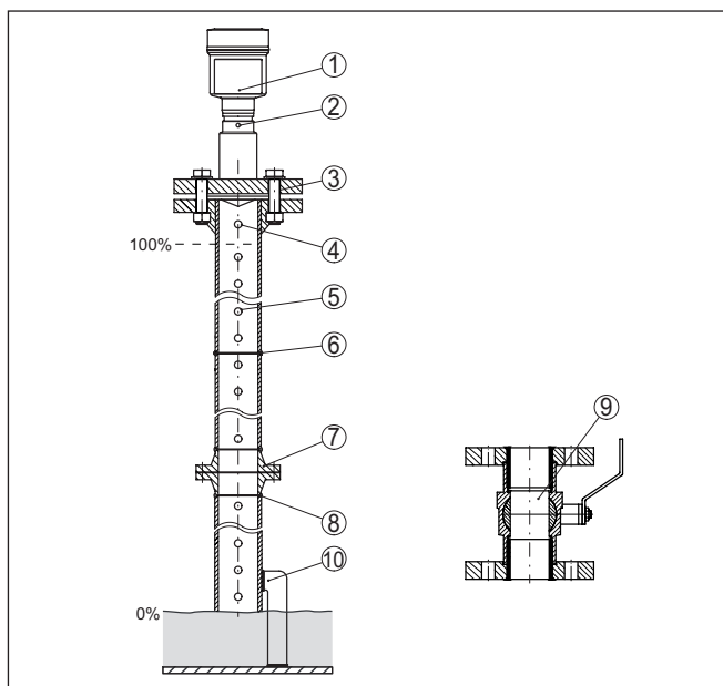
Рис. 13: Монтаж в уравнильной трубе
