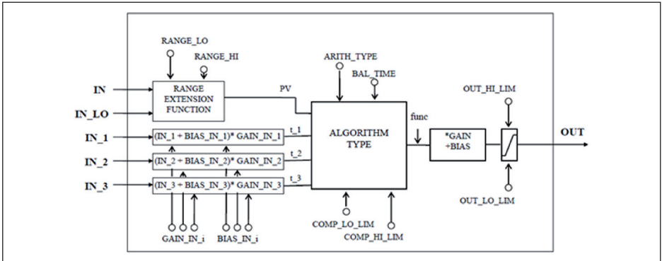
Рис. 55: Схема функционального блока Arithmetic
