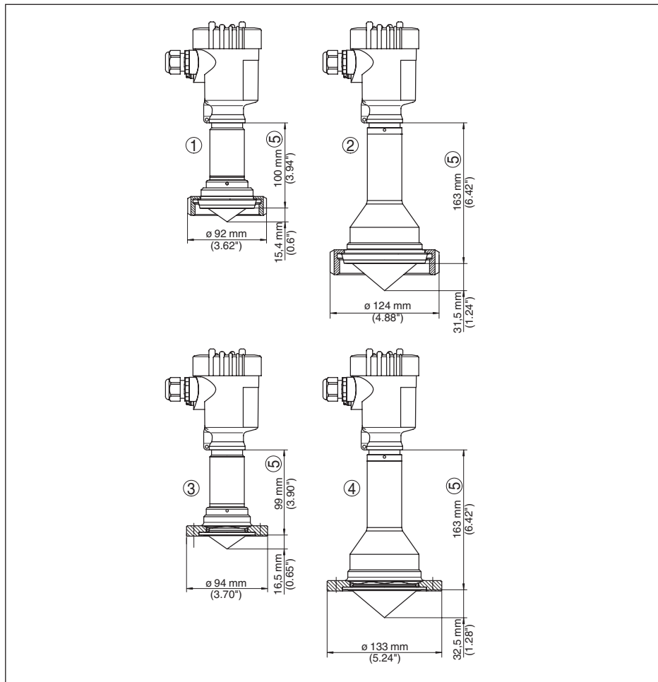
Рис. 65: VEGAPULS 63, гигиеническое присоединение 3
