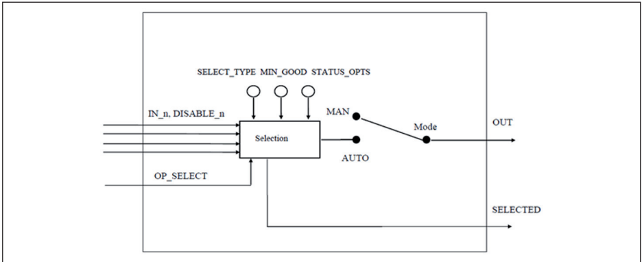
Рис. 54: Схема функционального блока Input Selector
