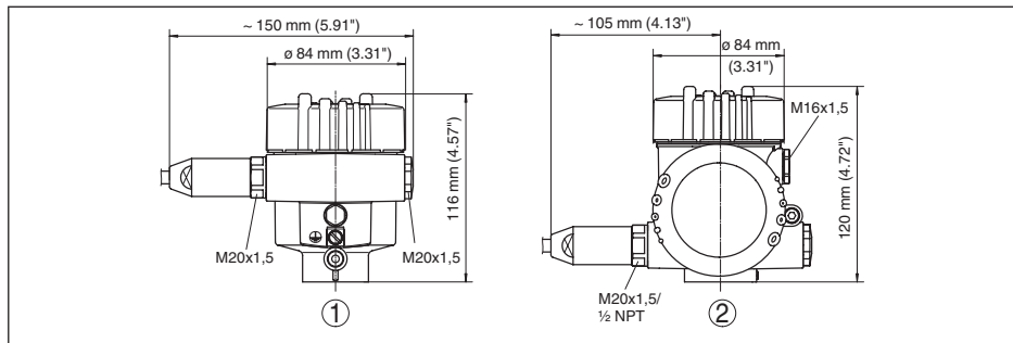
Рис. 58: Корпуса в исполнении IP 66/IP 68 (1 bar) - с установленным модулем индикации и настройки корпус выше на 9 mm/0.35 in
