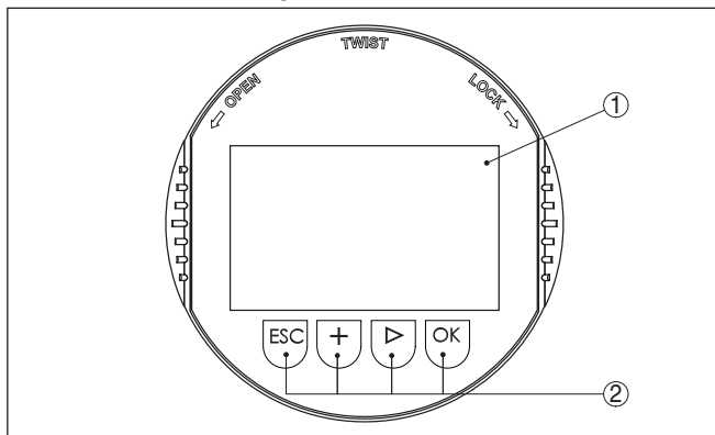
Рис. 26: Элементы индикации и настройки
