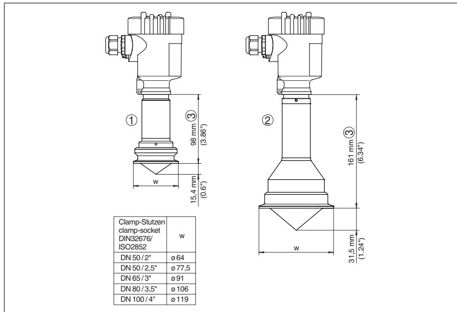
Рис. 64: VEGAPULS 63, гигиеническое присоединение 2
