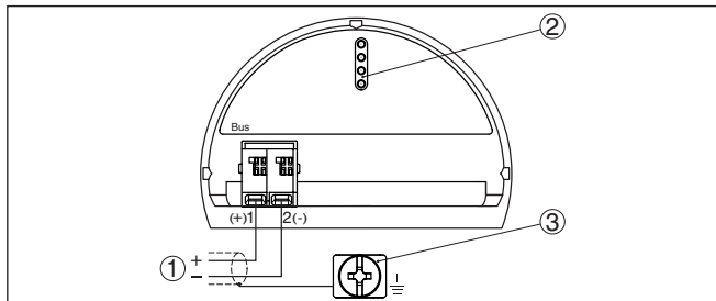
Рис. 18: Отсек подключения (двухкамерный корпус)
