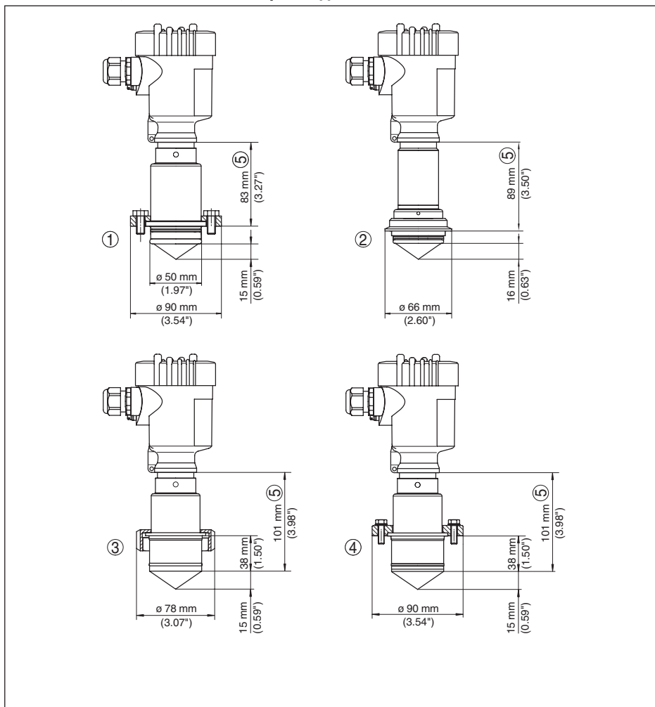
Рис. 58: VEGAPULS 63, гигиеническое присоединение 1
