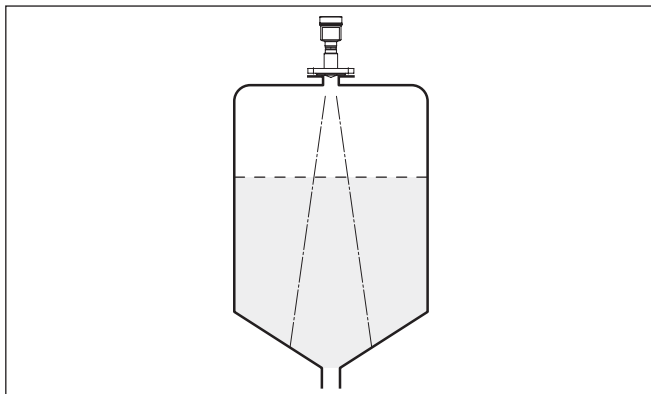
Рис. 7: Монтаж радарного датчика на емкостях с коническим дном
