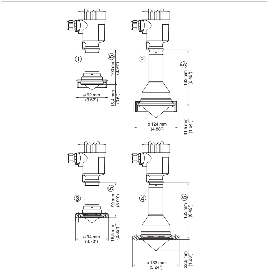
Рис. 60: VEGAPULS 63, гигиеническое присоединение 3
