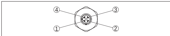
Рис. 22: Вид штекерного разъема
