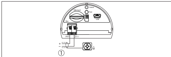
Рис. 19: Подключение модуля мобильной связи к питанию
