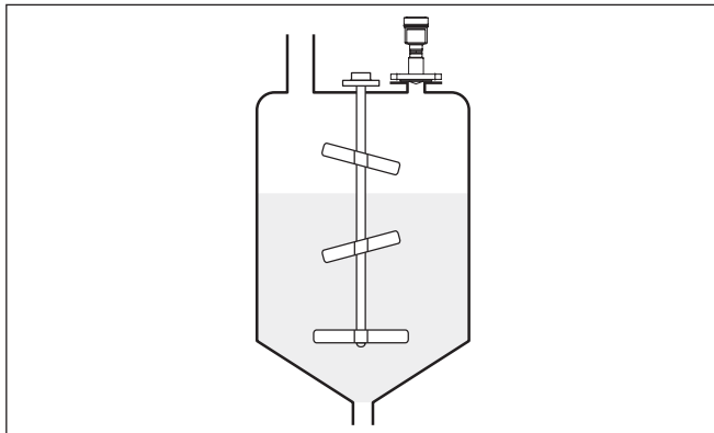
Рис. 12: Мешалки
