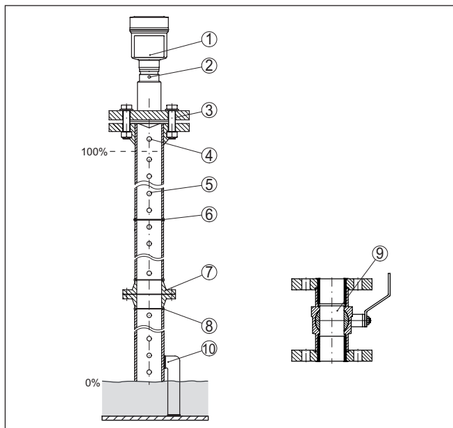
Рис. 13: Монтаж в уравнивной трубе
