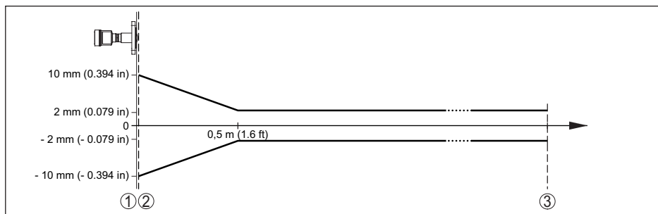
Рис. 47: Погрешность измерения при эталонных условиях
