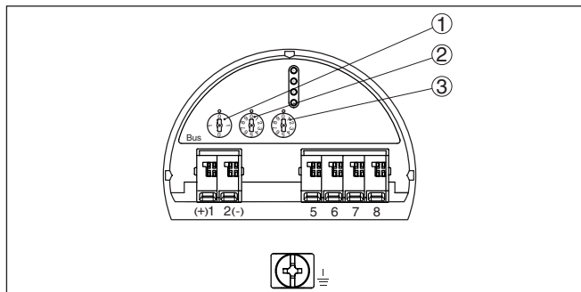
Рис. 24: Переключатели выбора адреса
