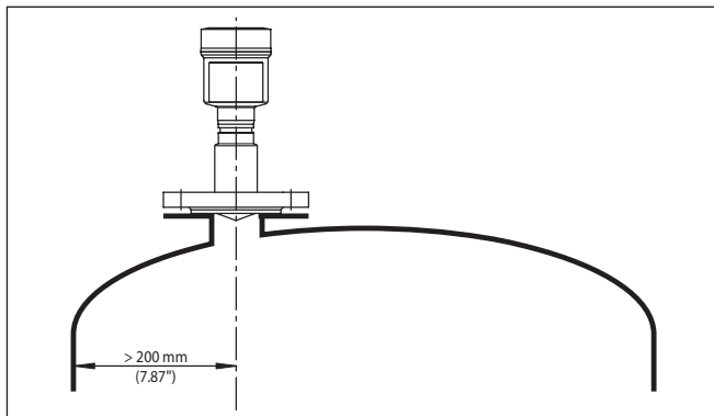
Рис. 6: Монтаж радарного датчика на округлой крыше емкости
