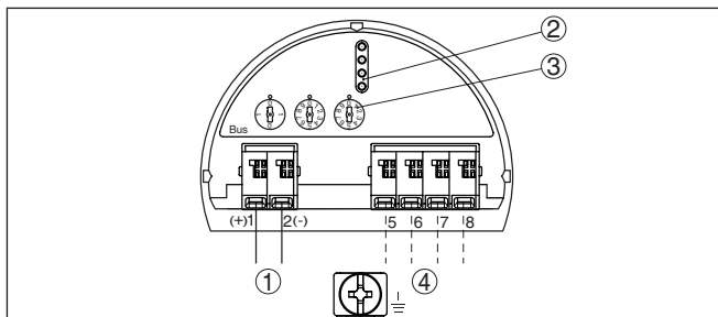
Рис. 20: Отсек электроники (двухкамерный корпус)
