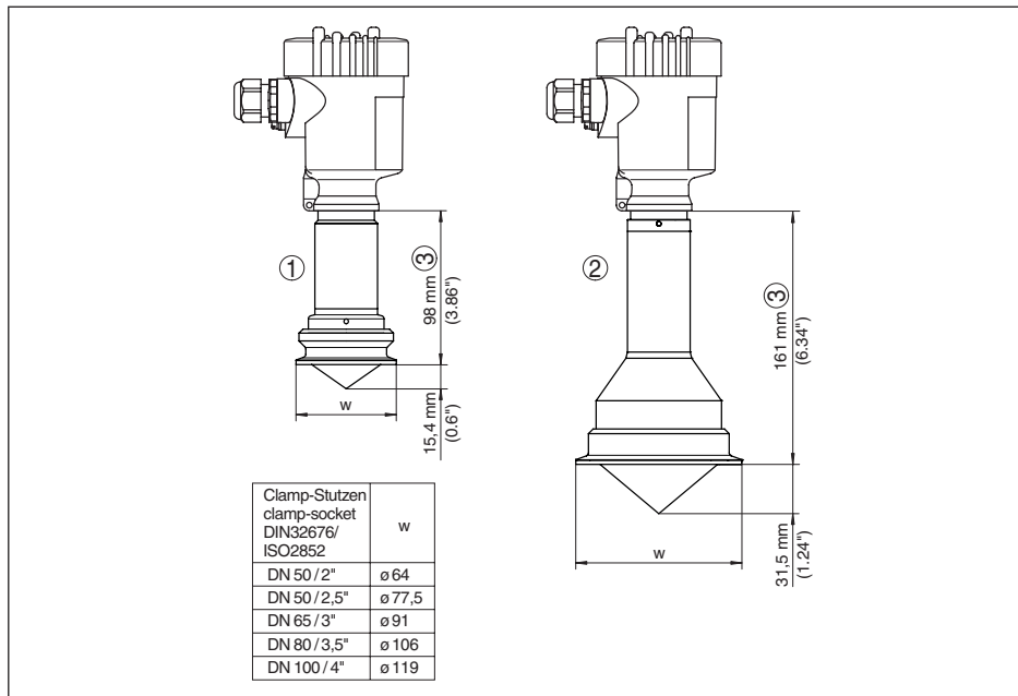
Рис. 59: VEGAPULS 63, гигиеническое присоединение 2
