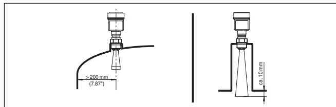
Рис. 1: Расстояние от антенны до стенки емкости/крыши емкости
