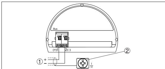
Рис. 21: Отсек подключения (двухкамерный корпус Ex d)
