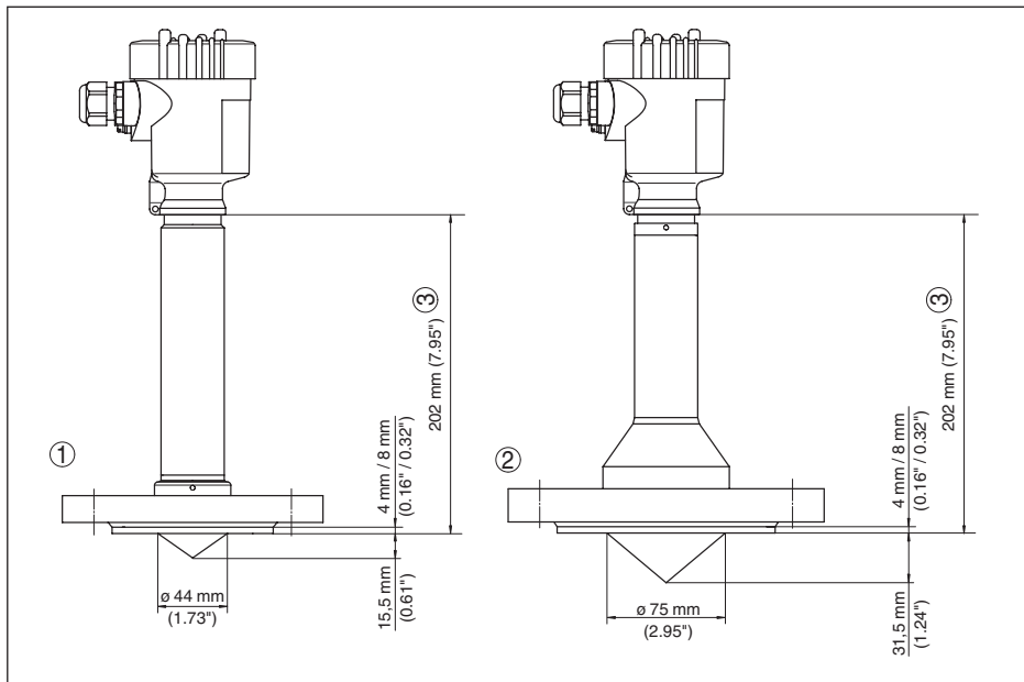
Рис. 57: VEGAPULS 63, фланцевое исполнение, для низких температур
