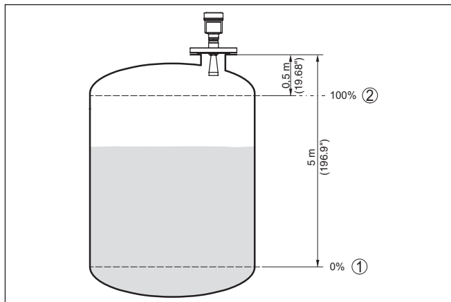
Рис. 28: Пример выполнения Установки Min./Max.
