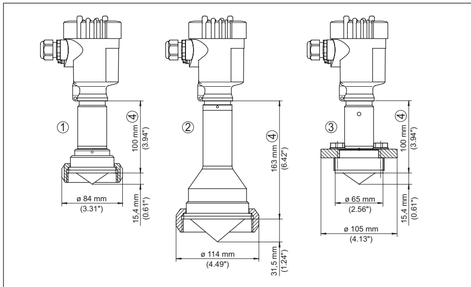
Рис. 61: VEGAPULS 63, гигиеническое присоединение 4
