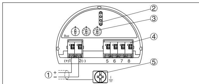
Рис. 16: Отсек электроники и подключения (однокамерный корпус)
