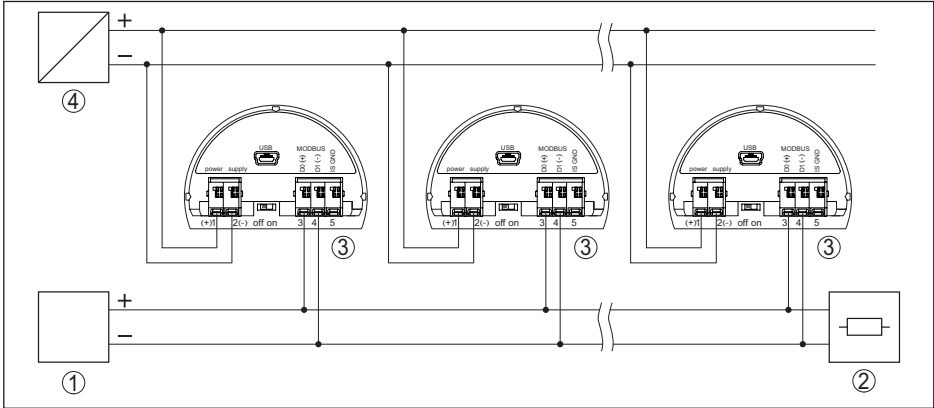
Рис. 28: Архитектура шины Modbus
