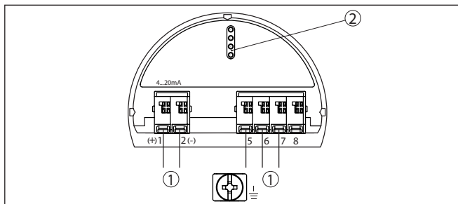
Рис. 16: Отсек электроники (двухкамерный корпус)
