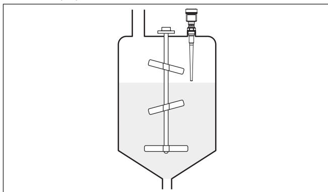
Рис. 13: Мешалки
