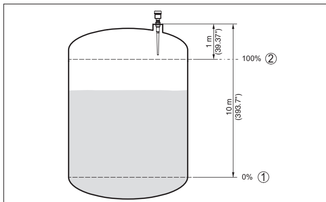
Рис. 20: Пример выполнения Установки Min./Max.
