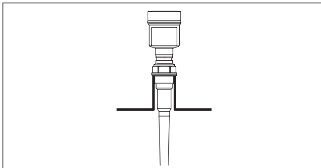
Рис. 10: Рекомендуемая высота монтажного патрубка
