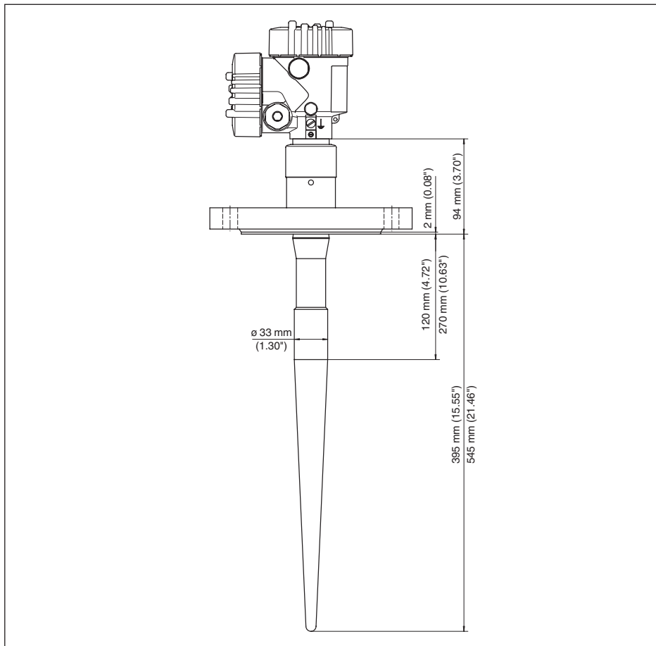
Рис. 36: VEGAPULS 65 во фланцевом исполнении для патрубков высотой 100 мм (неактивная длина 120 мм) или 250 мм (неактивная длина 270 мм)
