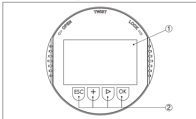
Рис. 19: Элементы индикации и настройки
