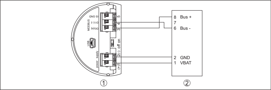
Рис. 30: Подключение VEGAPULS 65 к RTU ABB Total Flow
