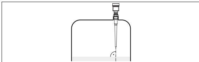
Рис. 11: Ориентация датчика на жидкостях
