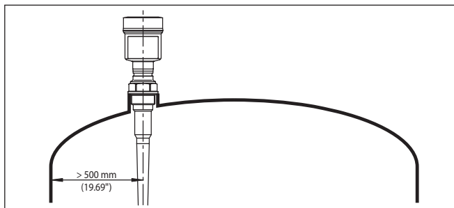
Рис. 7: Монтаж радарного датчика на округлой крыше емкости
