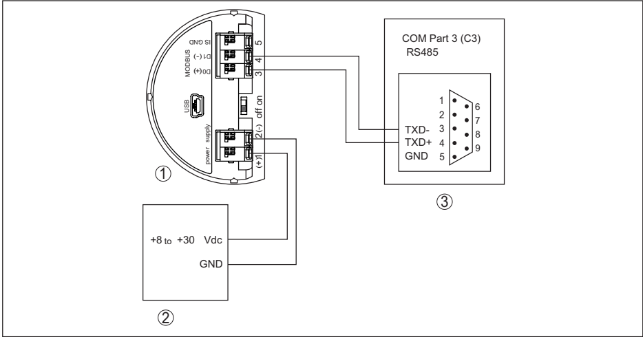
Рис. 33: Подключение VEGAPULS 65 к RTU ScadaPack
