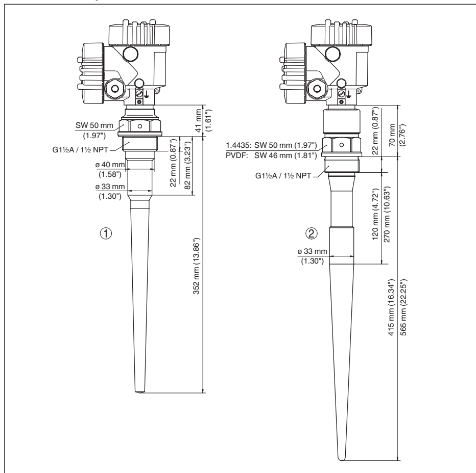
Рис. 35: VEGAPULS 65, резьбовое исполнение
