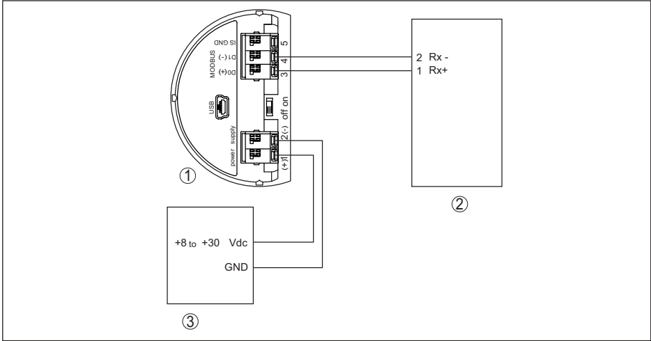
Рис. 31: Подключение VEGAPULS 65 к RTU Thermo Electron Autopilot
