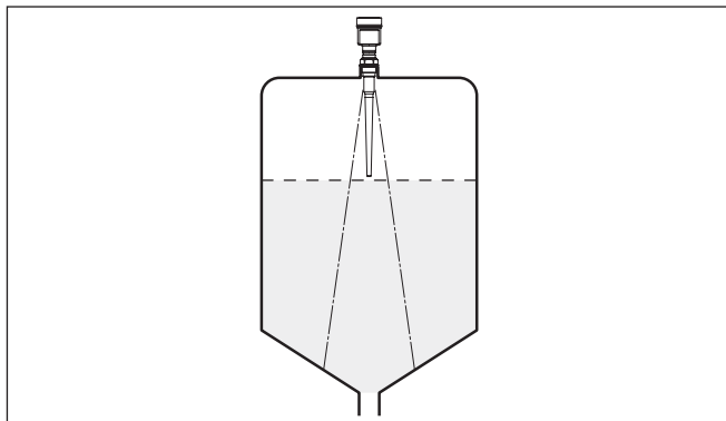
Рис. 8: Монтаж радарного датчика на емкостях с коническим дном
