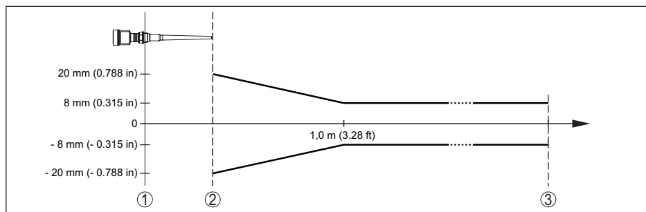
Рис. 27: Погрешность измерения при эталонных условиях
