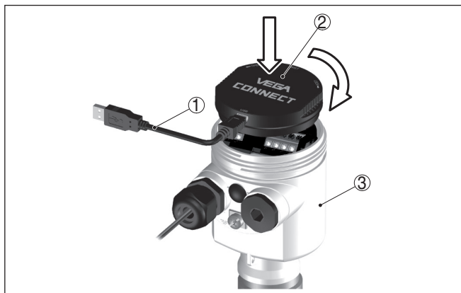
Рис. 21: Подключение ПК через интерфейсный адаптер прямо к датчику
