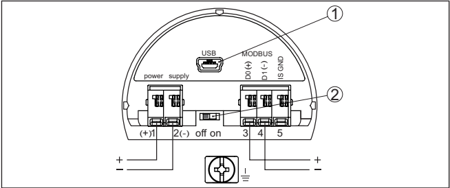
Рис. 17: Отсек подключения
