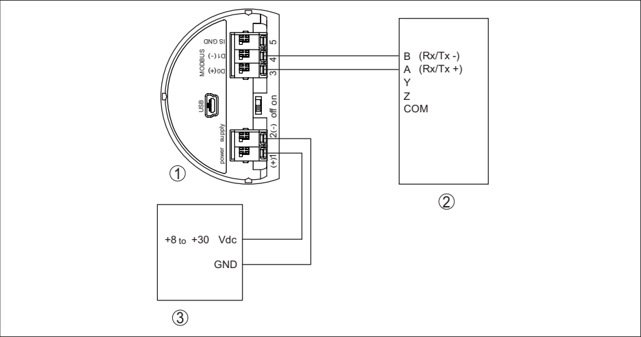
Рис. 29: Подключение VEGAPULS 65 к RTU Fisher ROC 809
