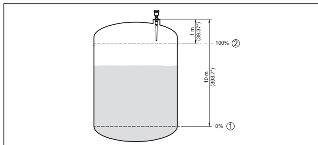
Рис. 3: Пример параметрирования
