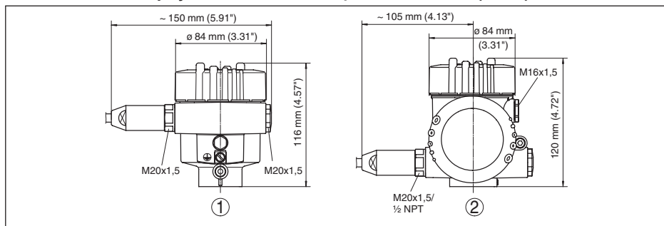
Рис. 51: Корпуса в исполнении IP 66/IP 68 (1 bar) - с установленным модулем индикации и настройки корпус выше на 9 mm/0.35 in
