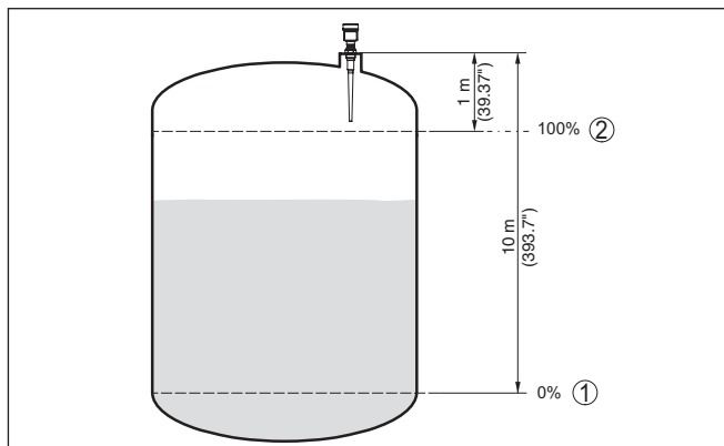
Рис. 26: Пример выполнения Установки Min./Max.
