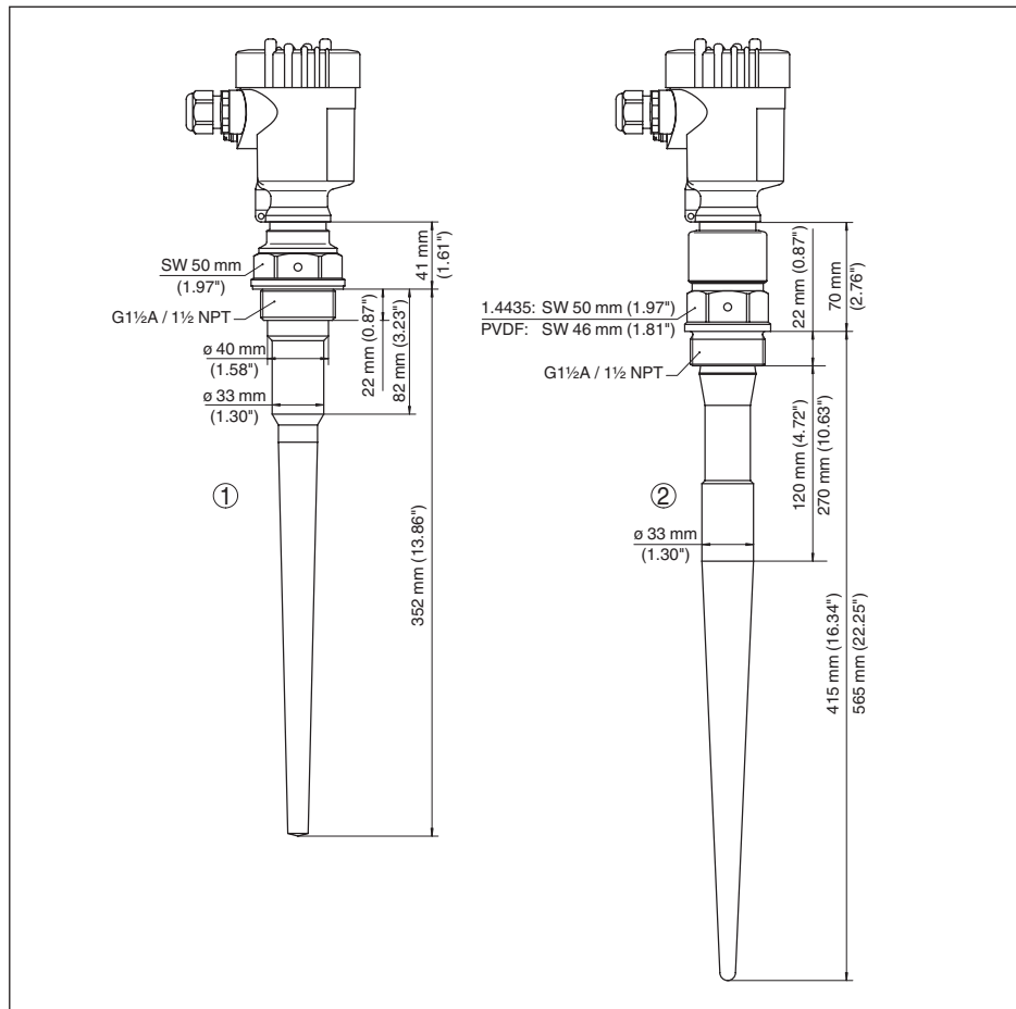
Рис. 52: VEGAPULS 65, резьбовое исполнение
