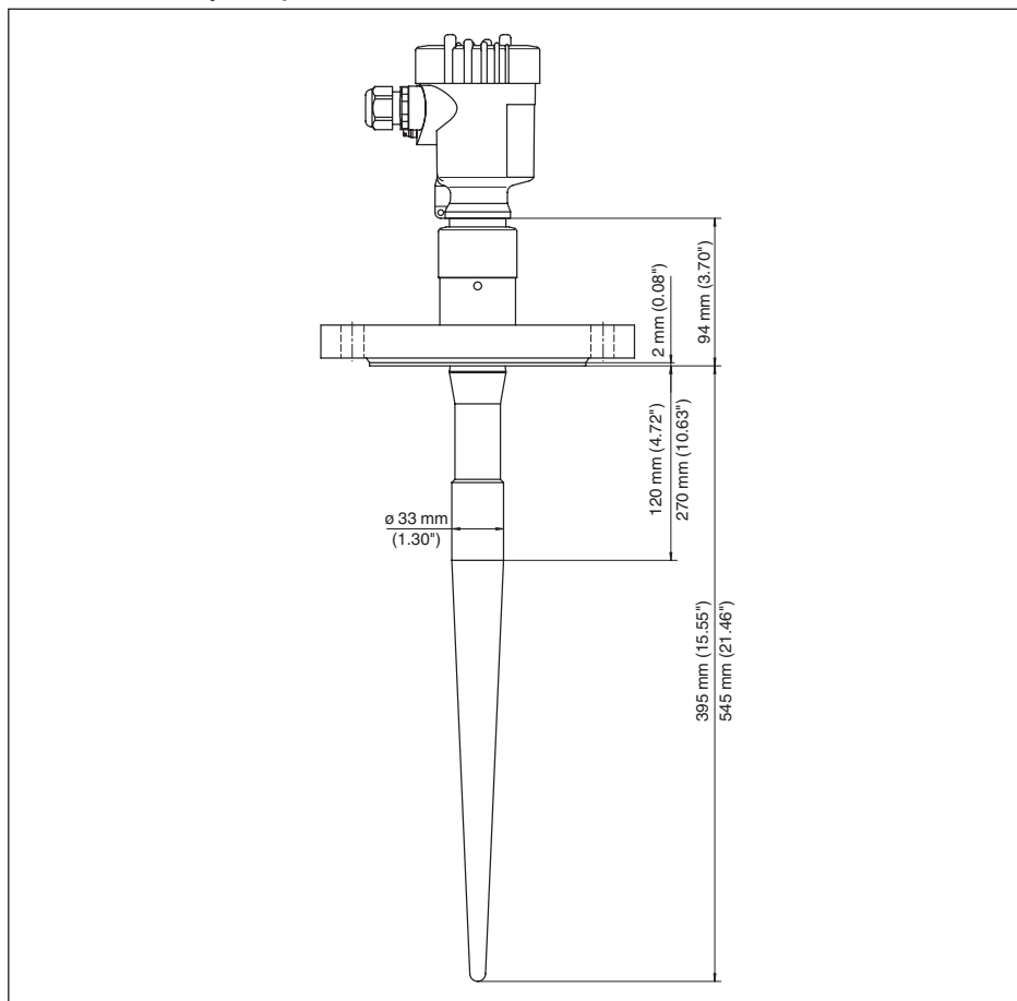
Рис. 53: VEGAPULS 65 во фланцевом исполнении для патрубков высотой 100 мм (неактивная длина 120 мм) или 250 мм (неактивная длина 270 мм)
