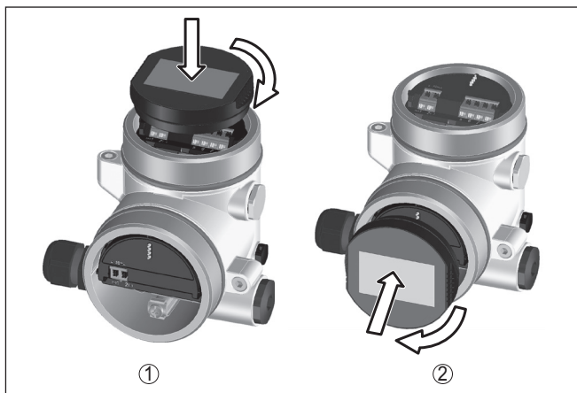
Рис. 24: Установка модуля индикации и настройки в двухкамерном корпусе
