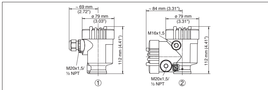
Рис. 49: Корпуса в исполнении IP 66/IP 68 (0,2 bar) - с установленным модулем индикации и настройки корпус выше на 9 mm/0.35 in
